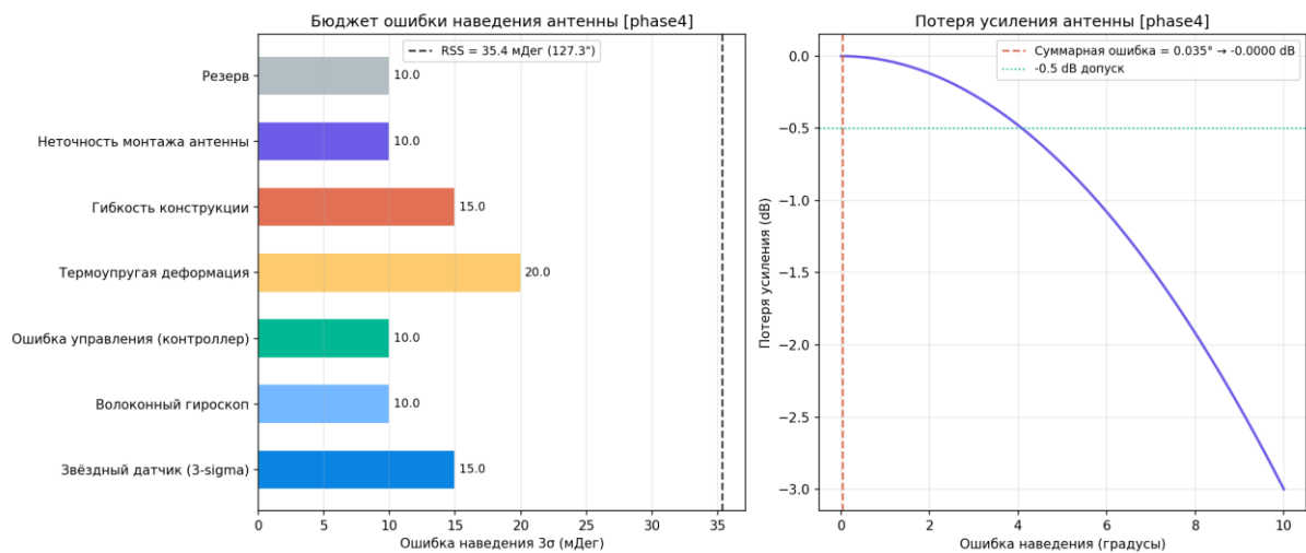
Рисунок 96 — Бюджет наведения антенны
