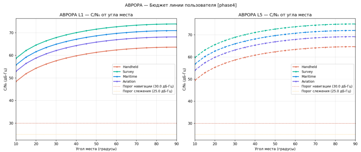
Рисунок 26 — Бюджет линии C/N 0 от угла места
