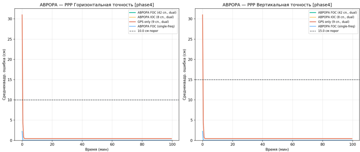
Рисунок 89 — Сравнение сходимости PPP
