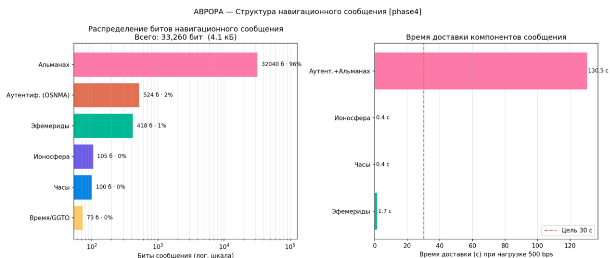
Рисунок 17 — Структура навигационного сообщения
