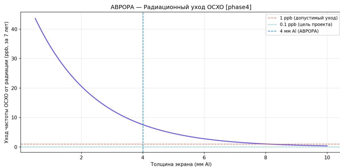
Рисунок 79 — Радиационный уход ОСХО
