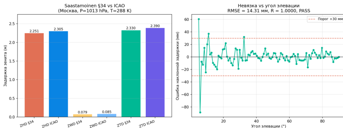
Рисунок 175 — Saastamoinen + NMF vs ICAO ISA
