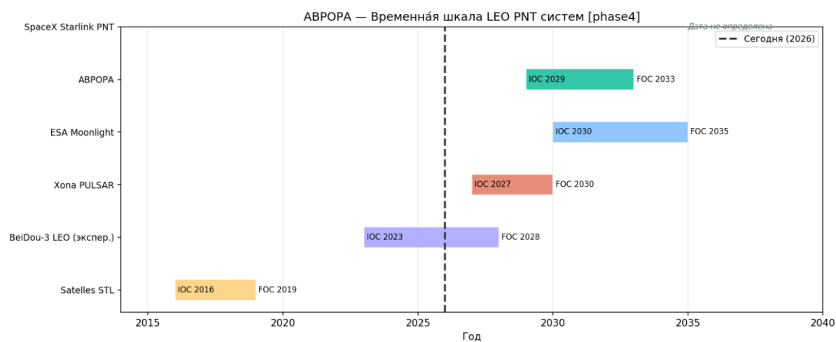
Рисунок 109 — Временная шкала LEO PNT
