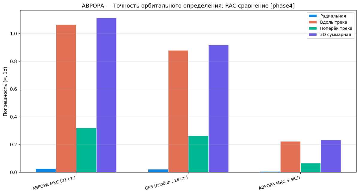
Рисунок 36 — Сравнение RAC ошибок
