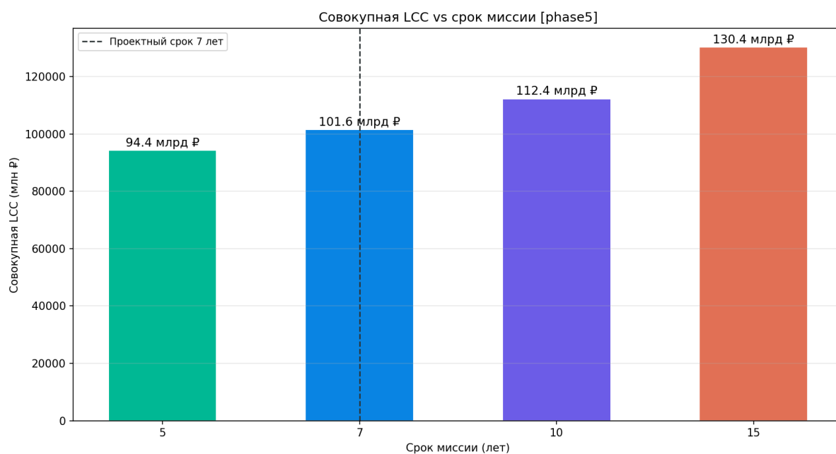
Рисунок 153 — LCC vs срок миссии
