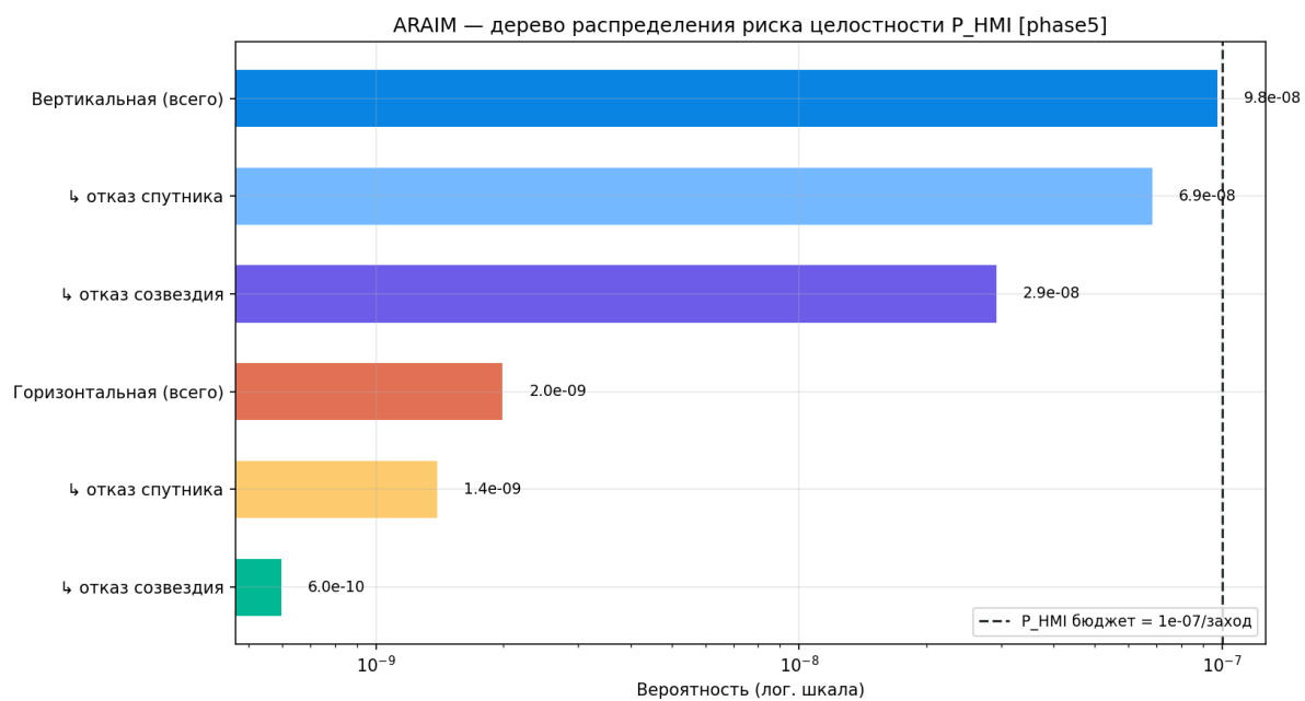
Рисунок 144 — Дерево распределения P_HMI
