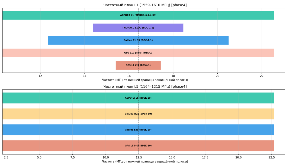
Рисунок 121 — Частотный план RNSS
