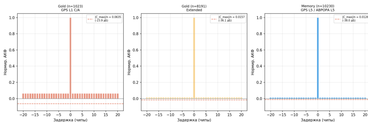
Рисунок 14 — АКФ сравнение кодов
