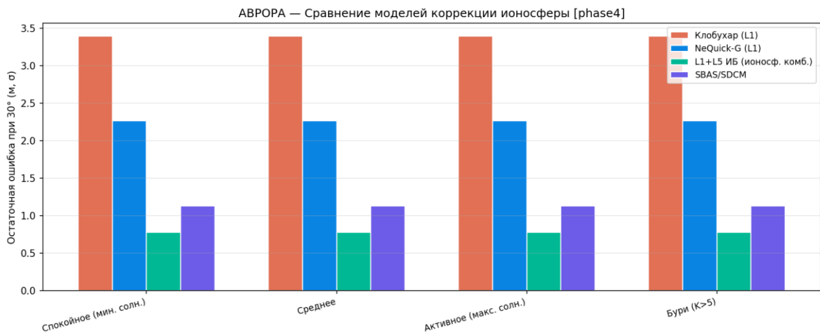
Рисунок 30 — Сравнение методов коррекции
