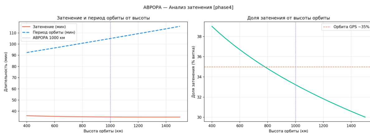
Рисунок 55 — Затенение и период vs высота
