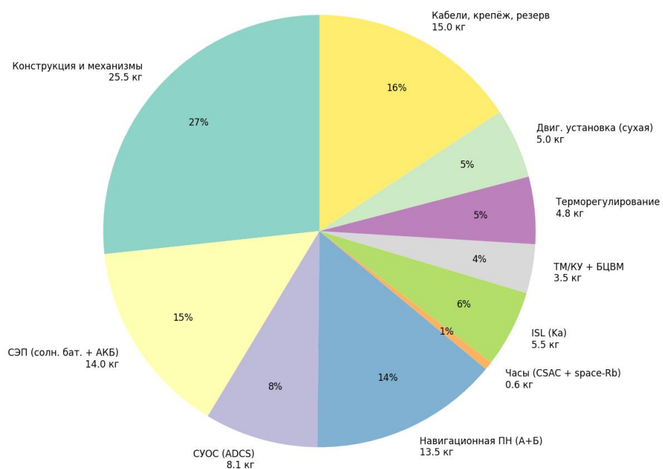
Рисунок 51 — Секторная диаграмма масс
