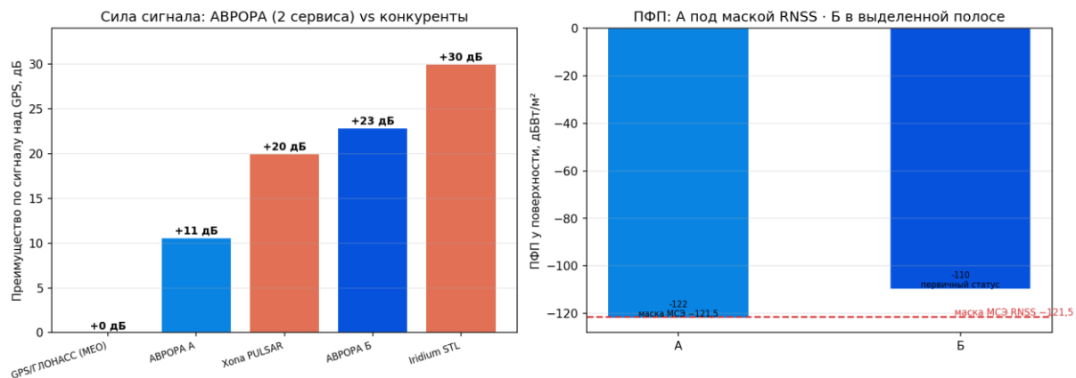
Рисунок 184 — Двухсервисная архитектура: сигнал и ПФП
