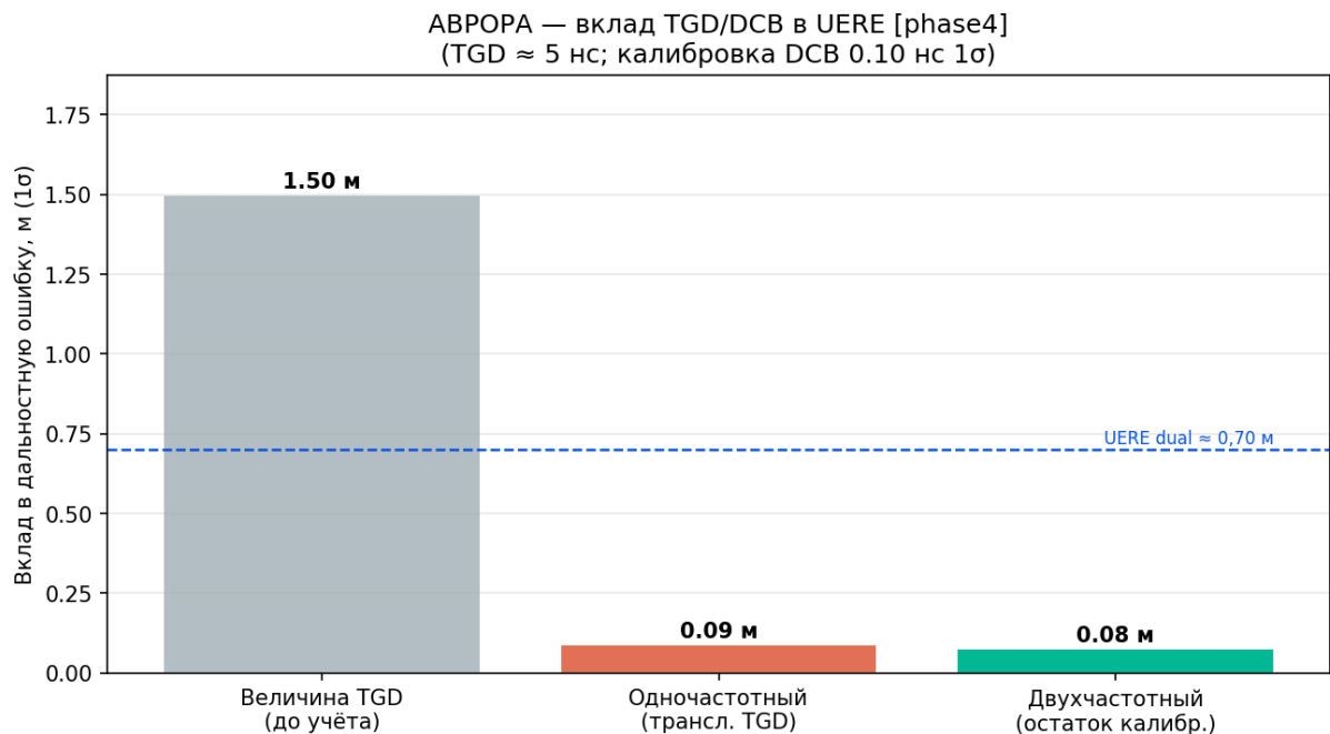
Рисунок 94 — Вклад TGD/DCB в UERE
