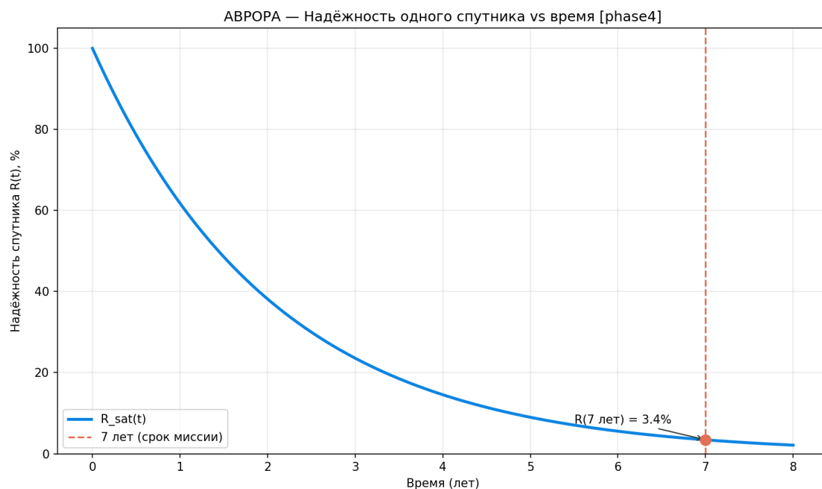
Рисунок 87 — Надёжность спутника vs время
