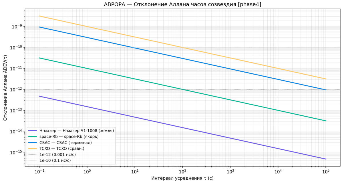
Рисунок 19 — ADEV — все типы часов
