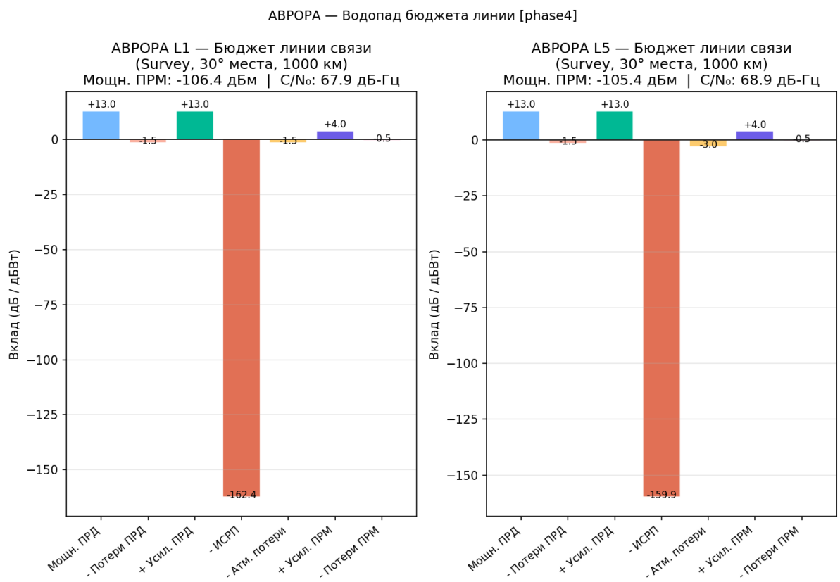
Рисунок 27 — Бюджет линии: составляющие
