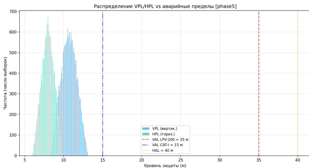
Рисунок 148 — PL vs AL
