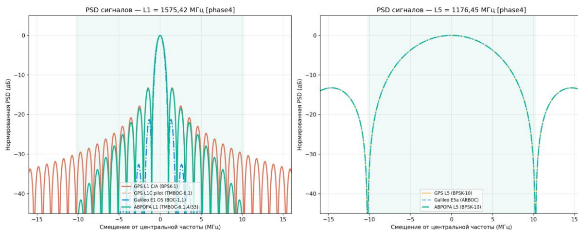
Рисунок 119 — PSD сигналов L1/L5
