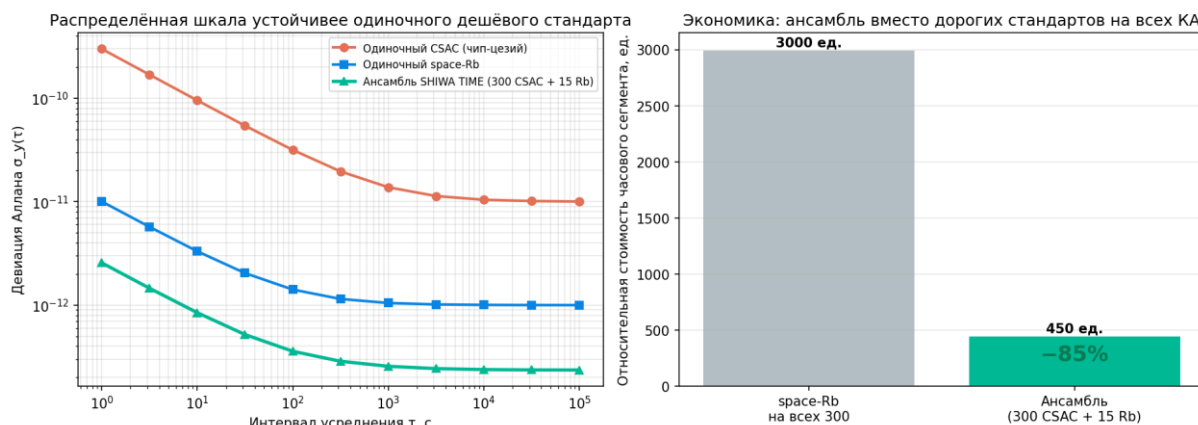
Рисунок 71 — SHIWA TIME-Space: ансамблевый эталон и экономика
