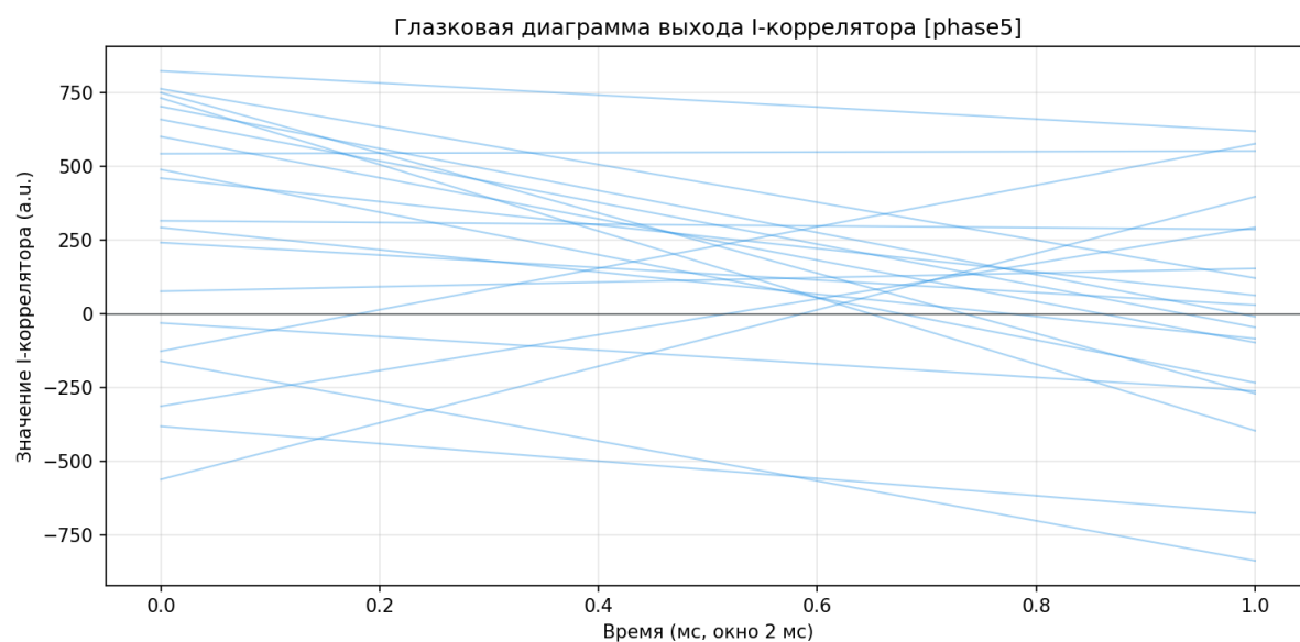
Рисунок 118 — Eye-диаграмма после слежения
