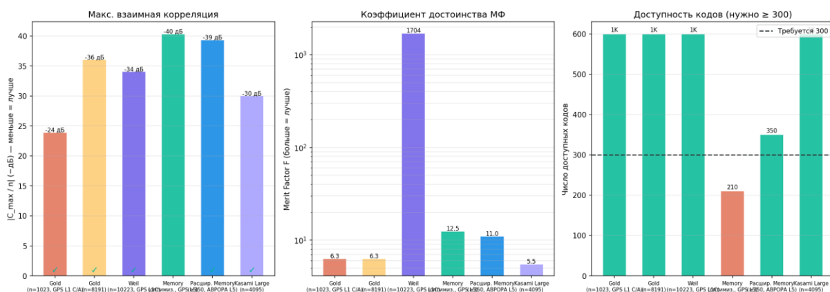
Рисунок 13 — Семейства кодов: Merit Factor и взаимная корреляция
