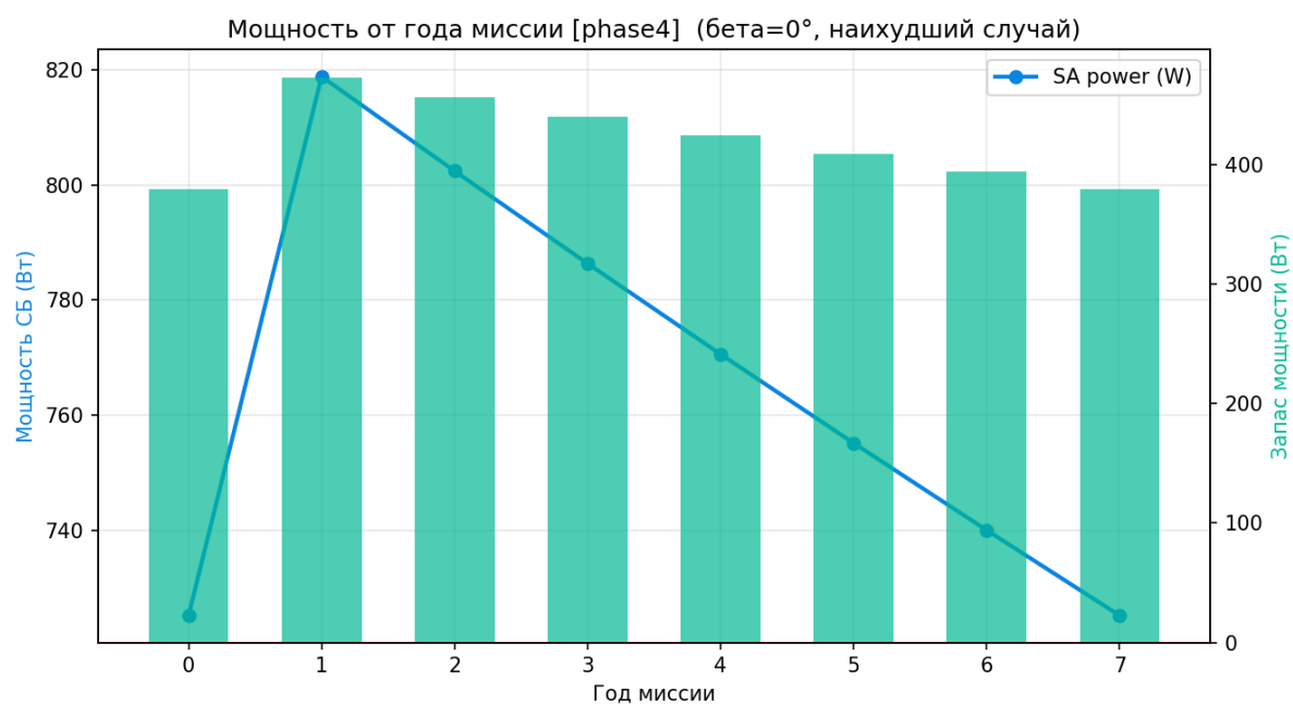
Рисунок 48 — Мощность СБ vs год миссии
