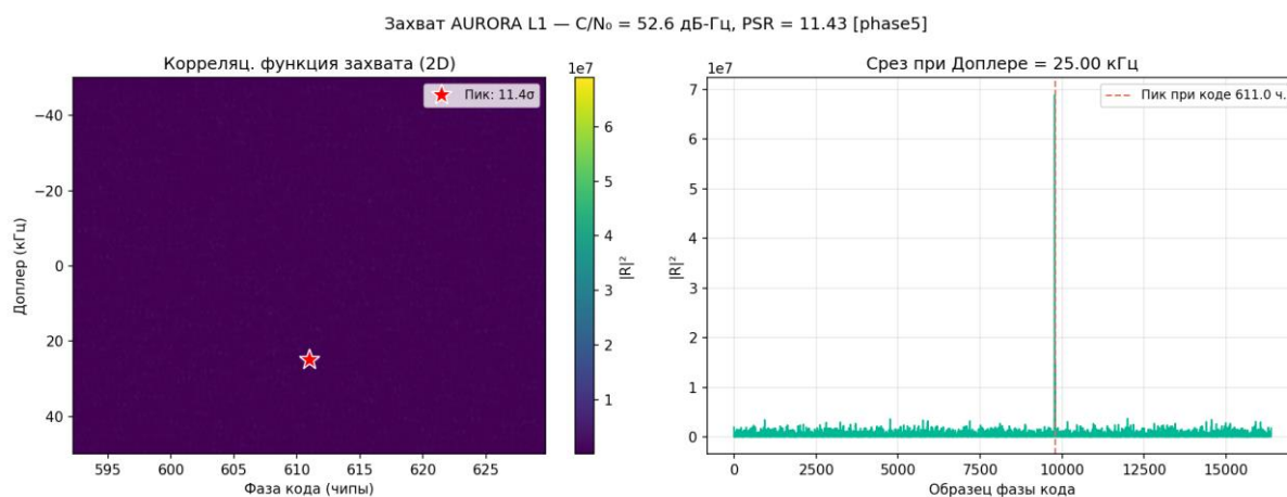
Рисунок 115 — 2D корреляц. функция захвата
