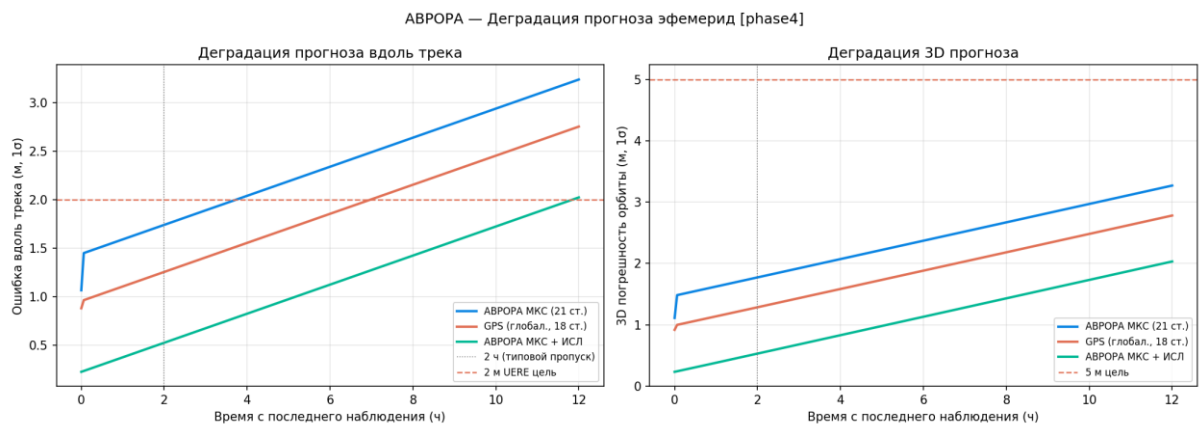
Рисунок 37 — Деградация прогноза эфемерид
