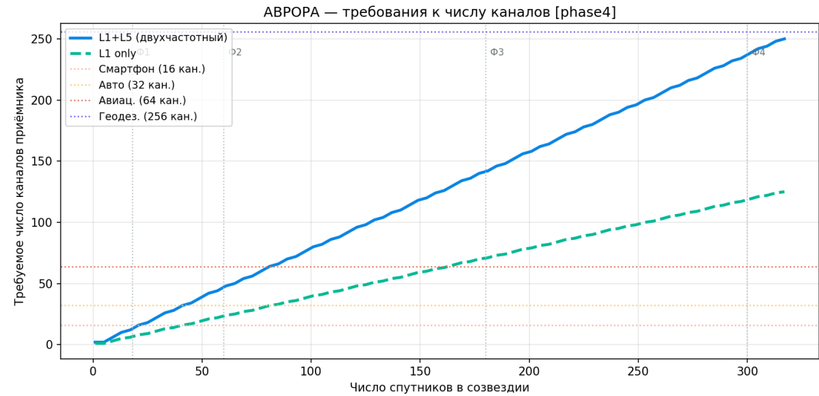
Рисунок 112 — Необходимое число каналов по фазам
