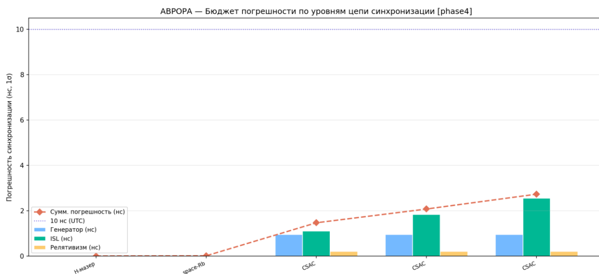
Рисунок 22 — Бюджет цепочки синхронизации
