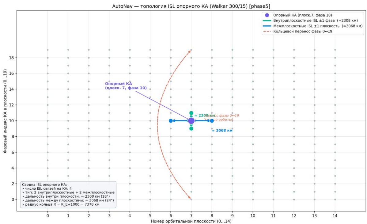
Рисунок 141 — Геометрия ISL-связей
