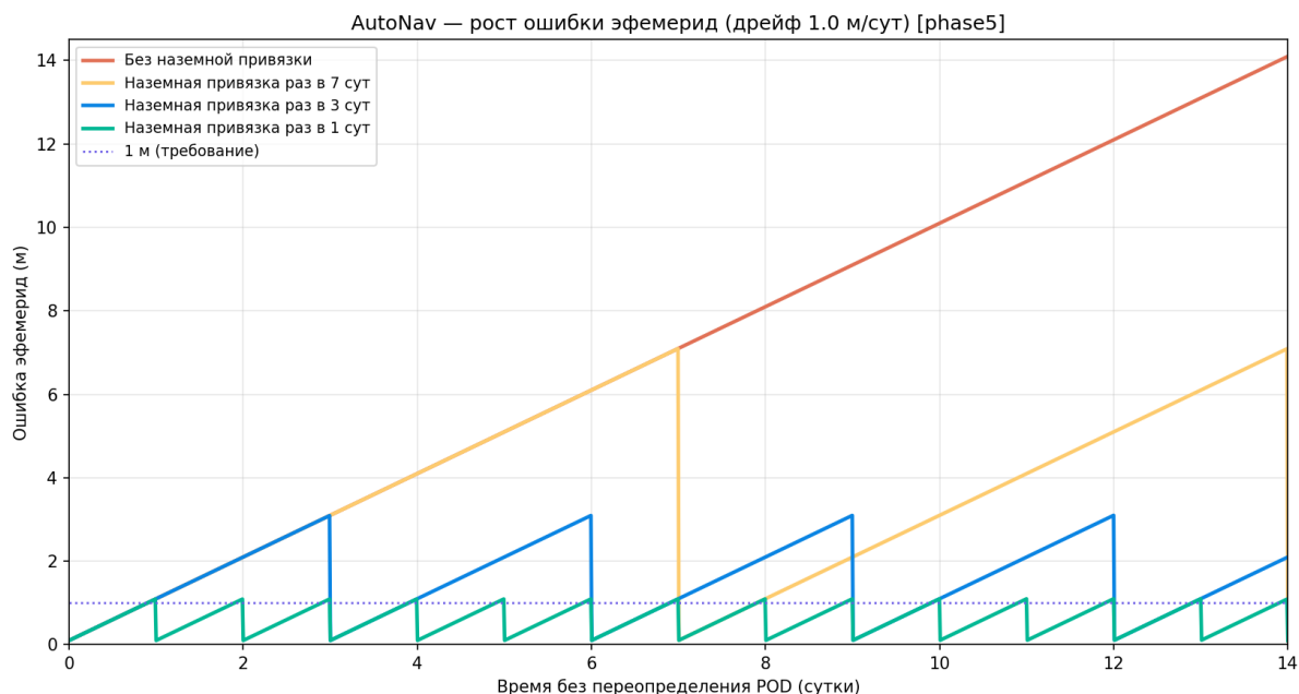
Рисунок 139 — Рост ошибки эфемерид
