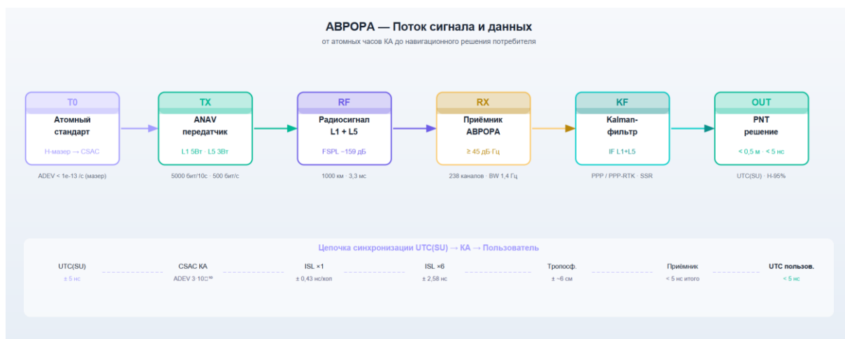
Рисунок 4 — Поток сигнала АВРОРА
