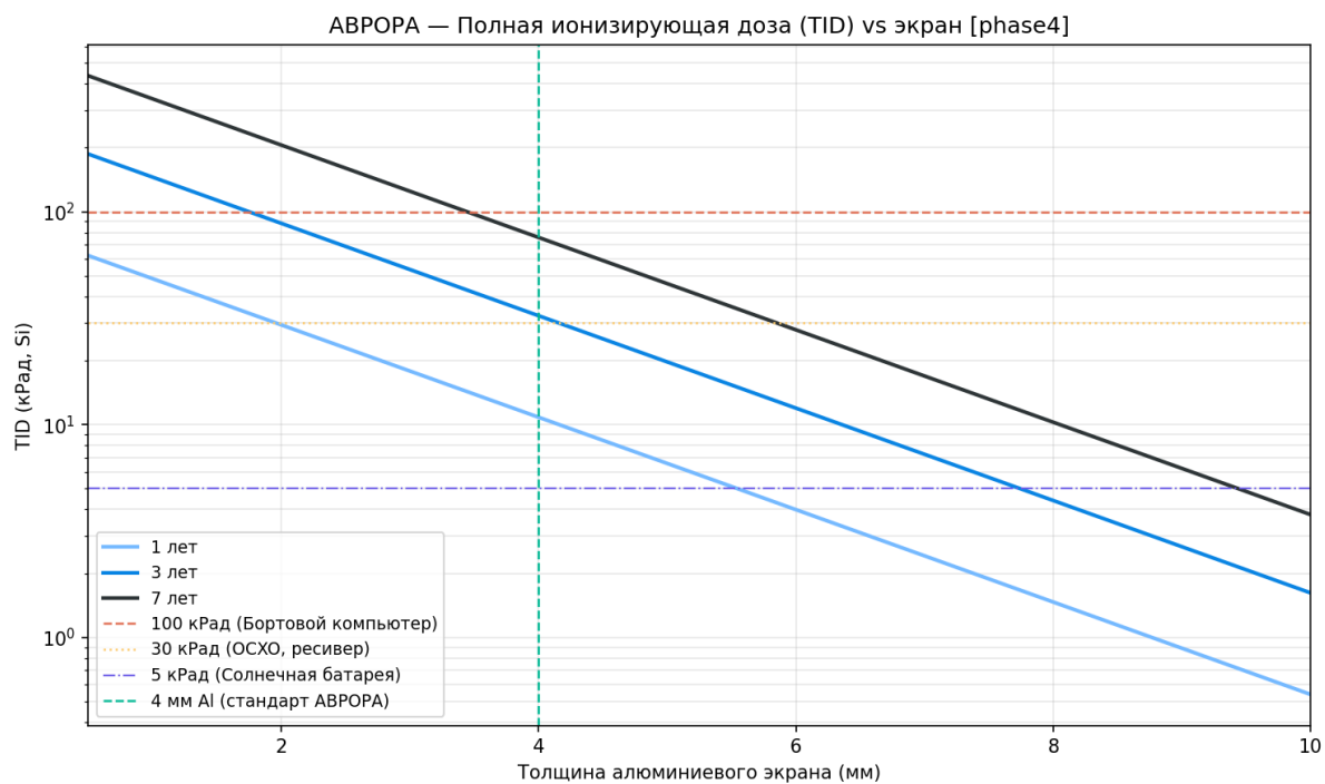
Рисунок 76 — TID vs толщина экрана
