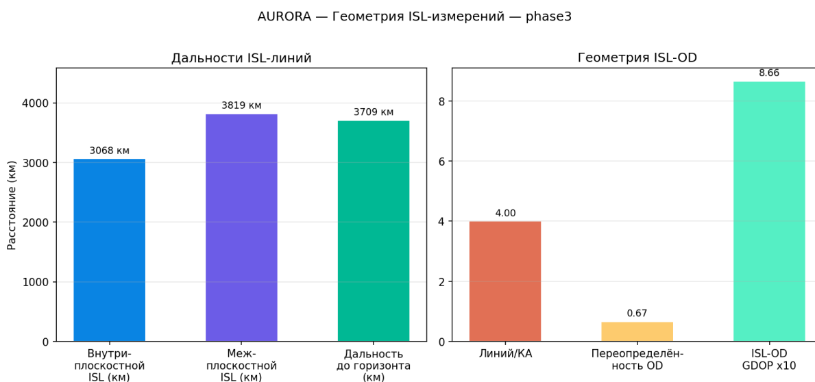
Рисунок 24 — ISL геометрия
