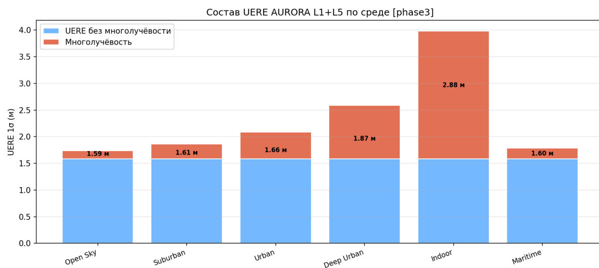
Рисунок 46 — UERE от многолучёвости
