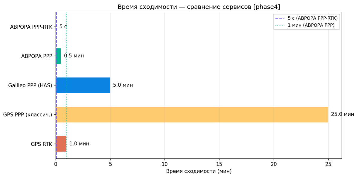
Рисунок 124 — Время сходимости — сравнение
