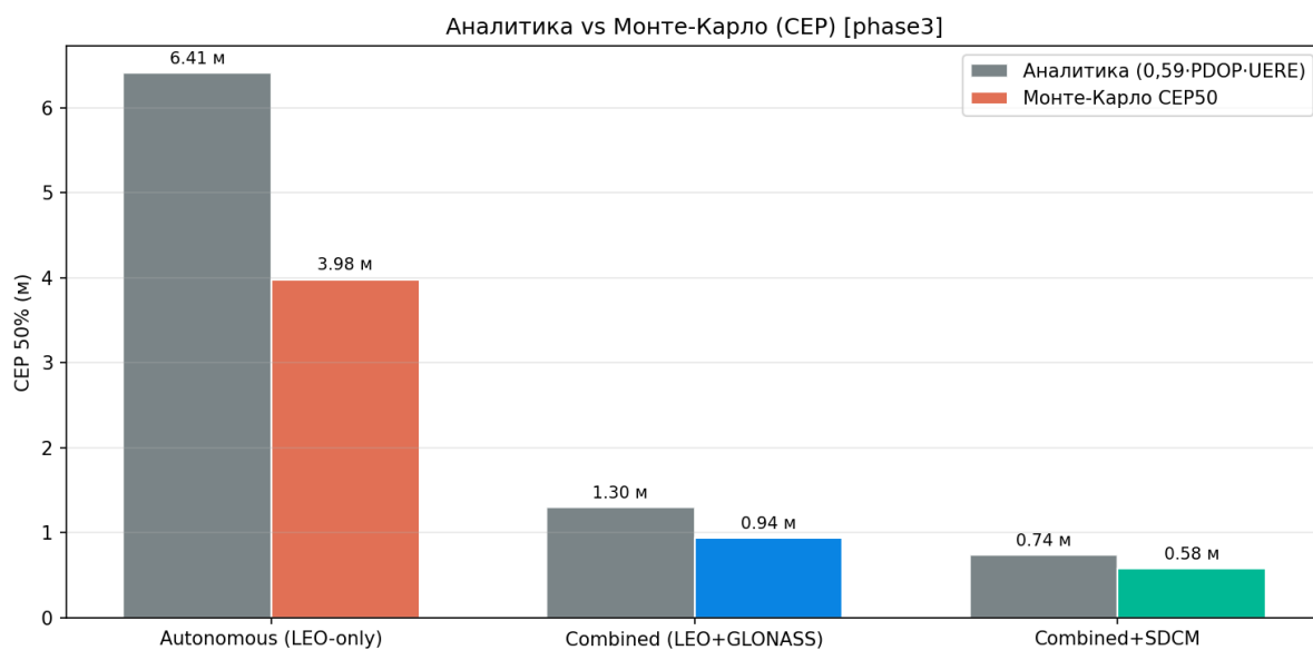
Рисунок 65 — Монте-Карло vs аналитика
