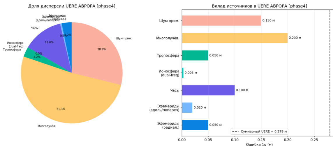
Рисунок 93 — Бюджет UERE ABPOPA
