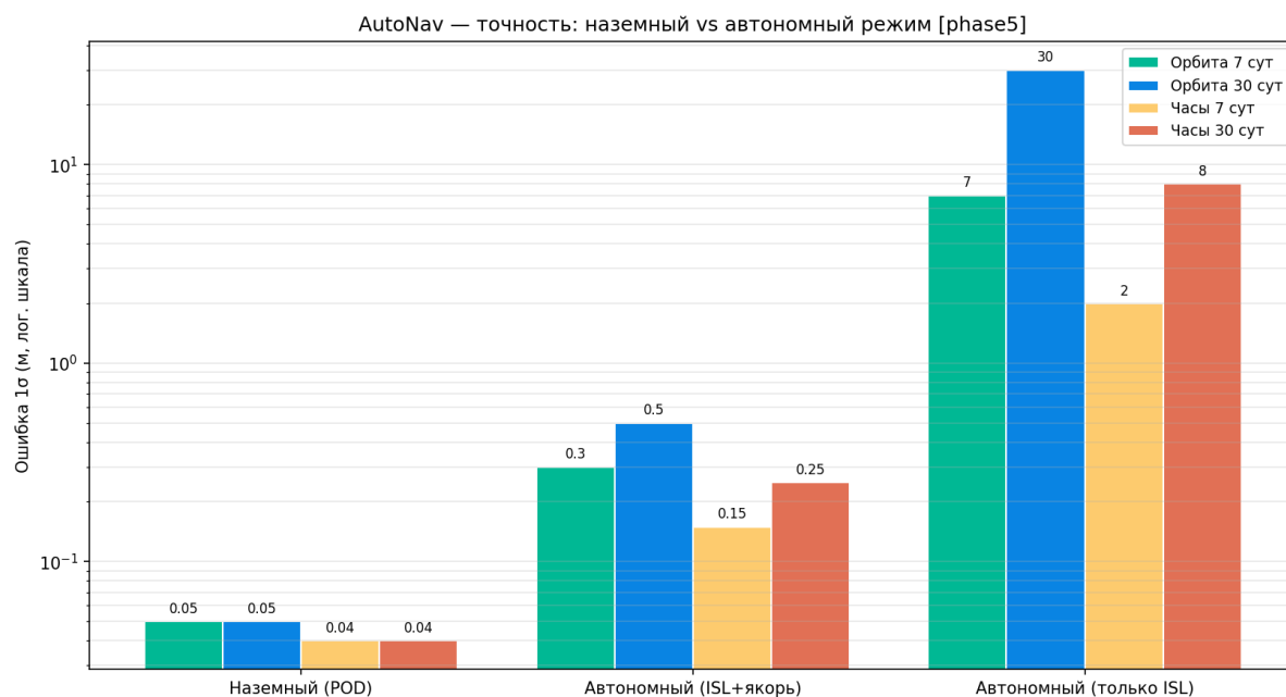
Рисунок 142 — Автономия vs наземный сегмент
