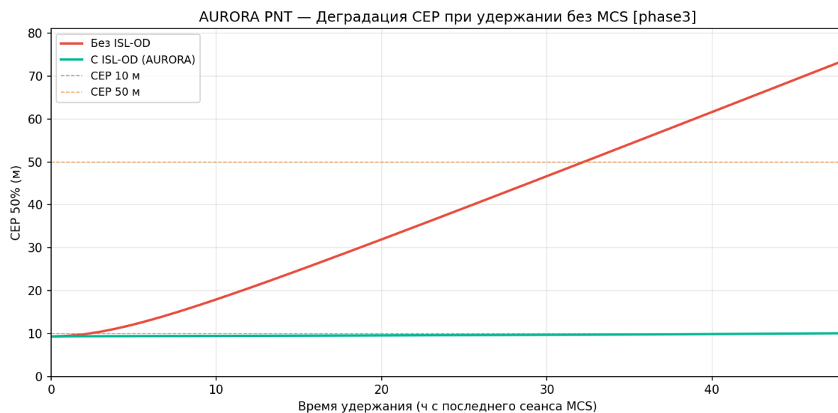
Рисунок 25 — ISL ухудшение CEP
