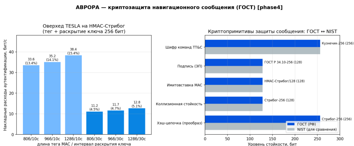
Рисунок 44 — Криптозащита навигационного сообщения на ГОСТ
