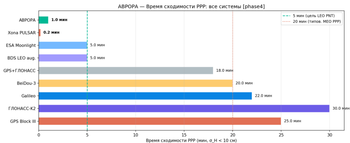
Рисунок 108 — Время сходимости PPP
