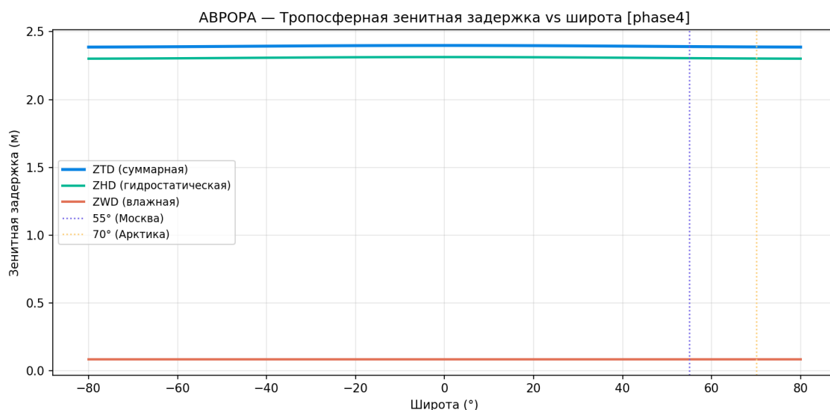
Рисунок 82 — ZTD по широте
