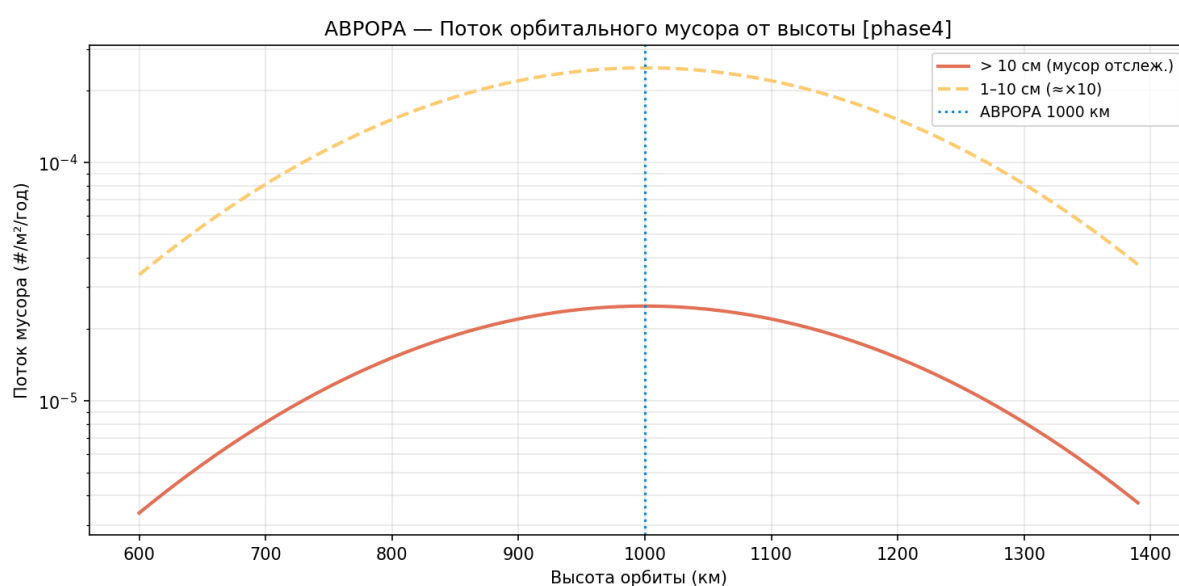
Рисунок 58 — Поток мусора vs высота
