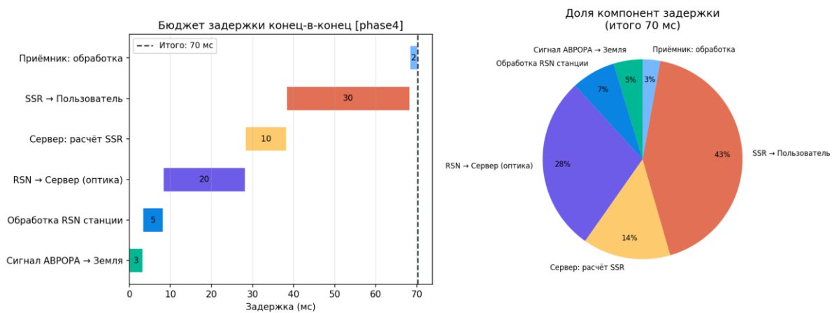
Рисунок 125 — Бюджет задержки E2E
