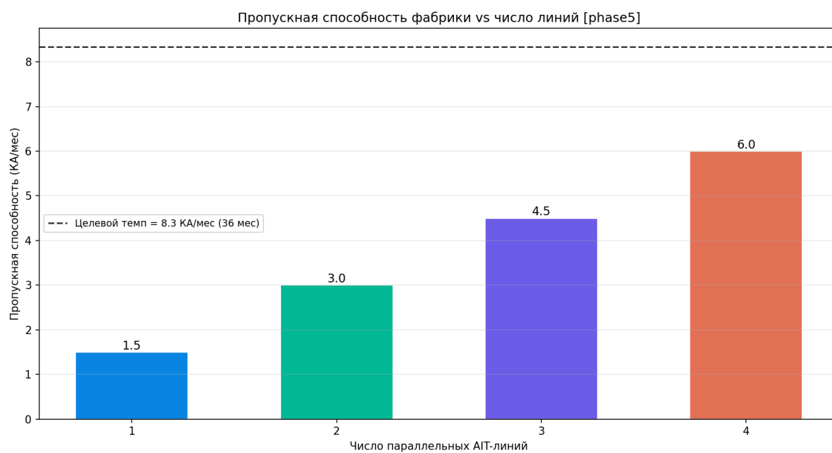
Рисунок 157 — Пропускная способность завода
