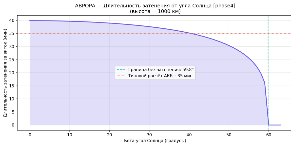
Рисунок 54 — Затенение vs бета-угол
