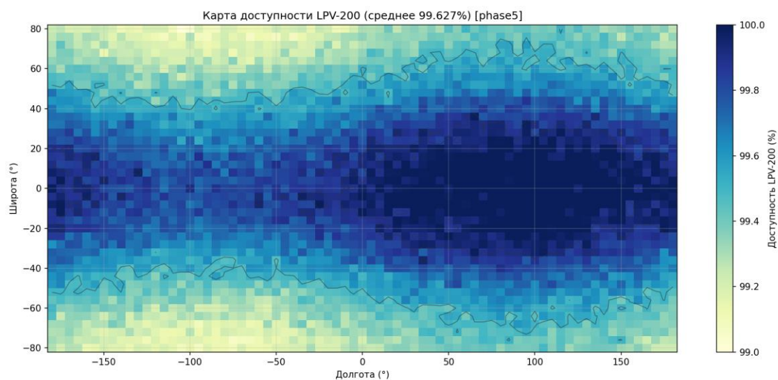
Рисунок 149 — Карта доступности LPV-200
