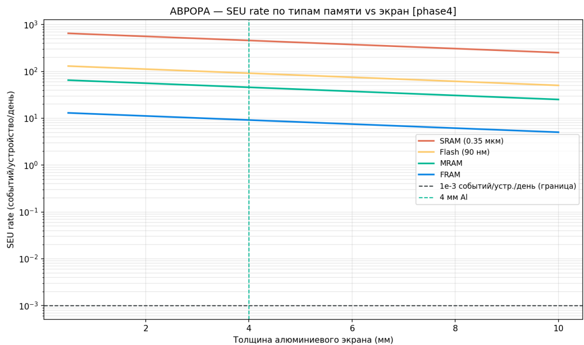
Рисунок 77 — SEU rate по типам памяти
