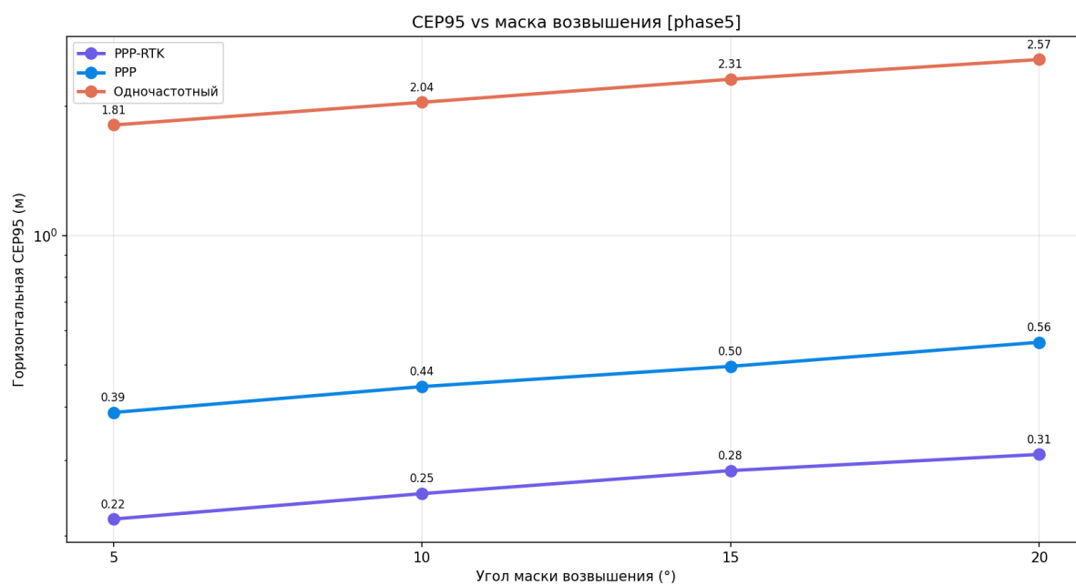
Рисунок 129 — СЕР95 vs маска возвышения
