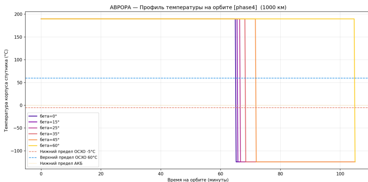
Рисунок 52 — Тепловой профиль за виток
