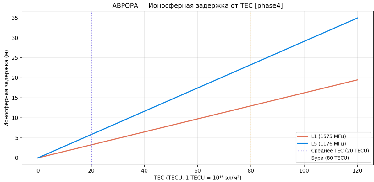
Рисунок 29 — Ионосферная задержка по частотам
