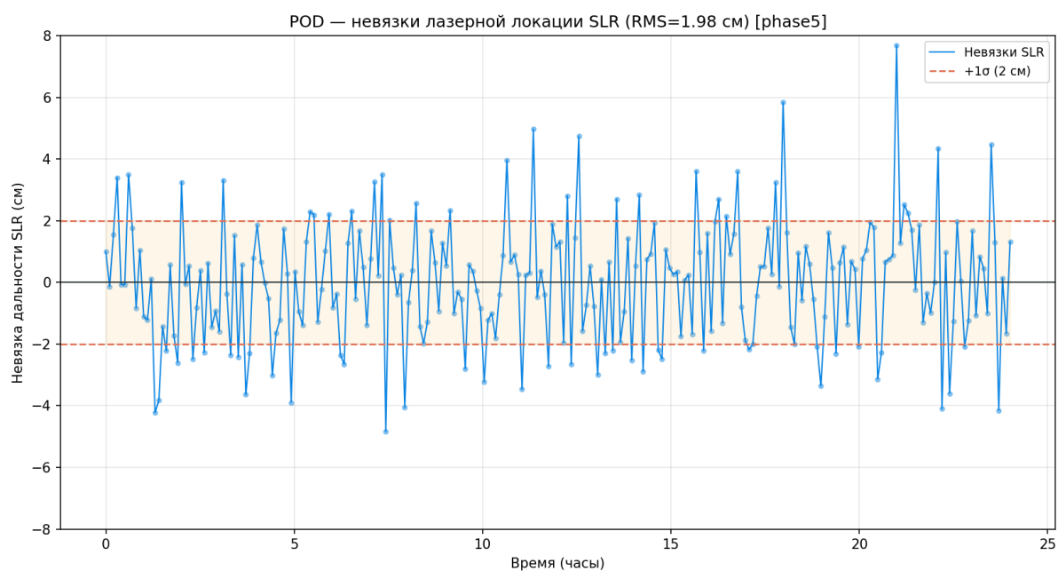
Рисунок 137 — Остатки валидации SLR
