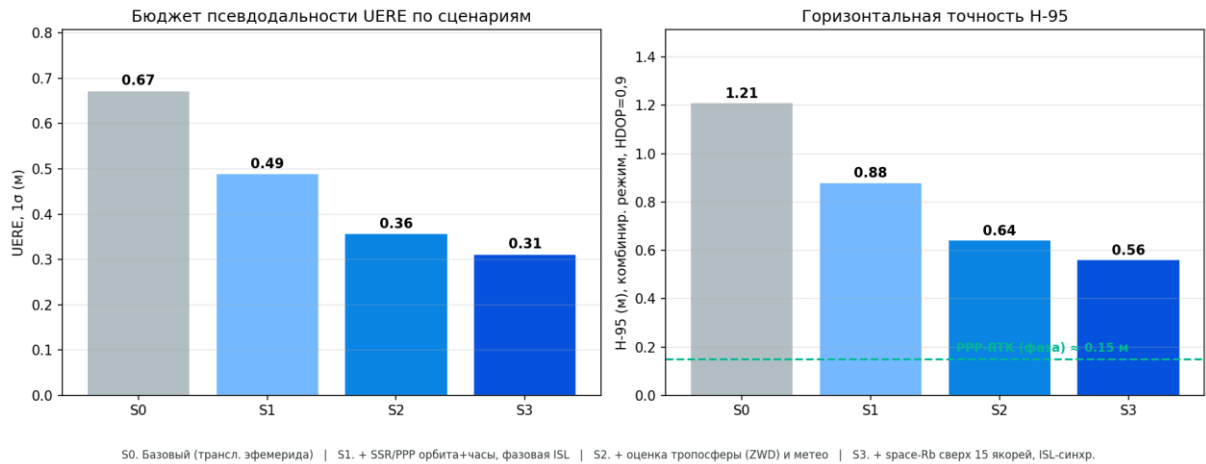
Рисунок 182 — Пути повышения точности позиционирования
