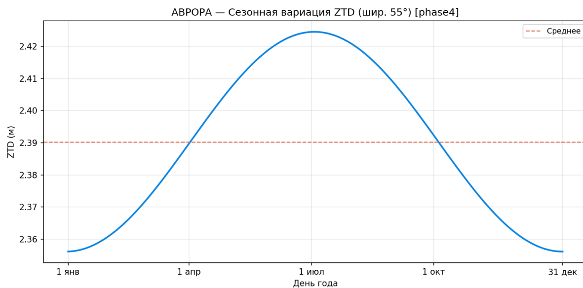
Рисунок 84 — Сезонные вариации ZTD
