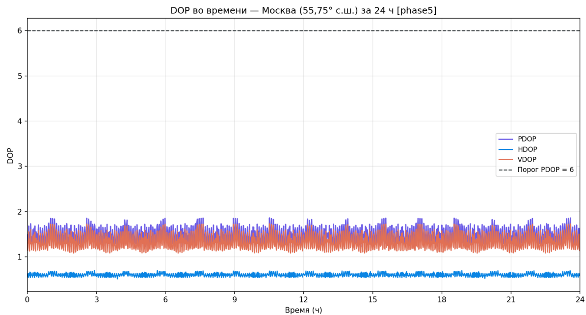
Рисунок 133 — PDOP за сутки (Москва)
