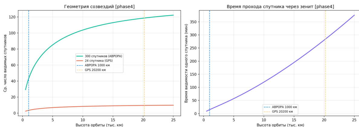
Рисунок 91 — Геометрия LEO vs MEO
