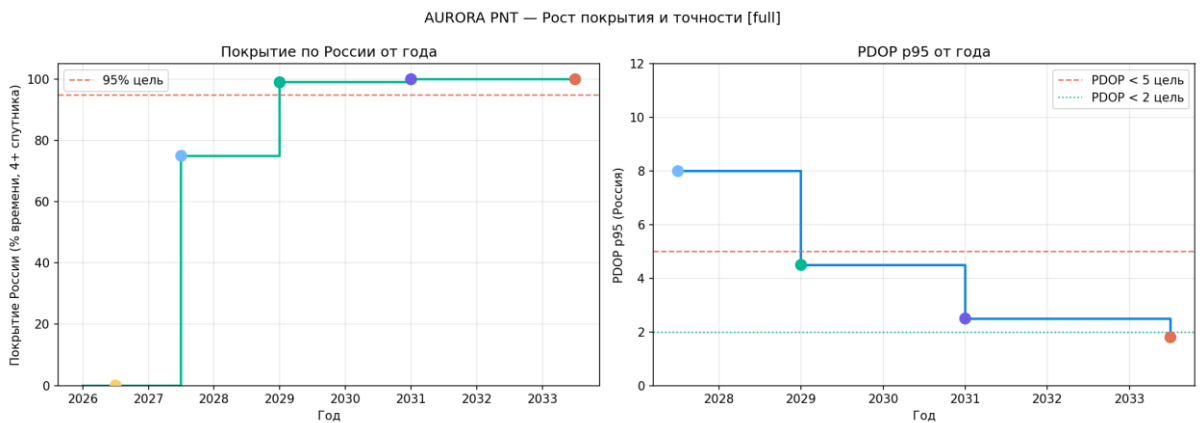
Рисунок 74 — Покрывание и PDOP vs год
