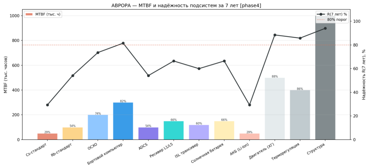
Рисунок 86 — MTBF и надёжность подсистем
