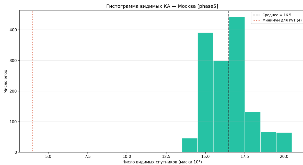
Рисунок 134 — Гистограмма числа спутников
