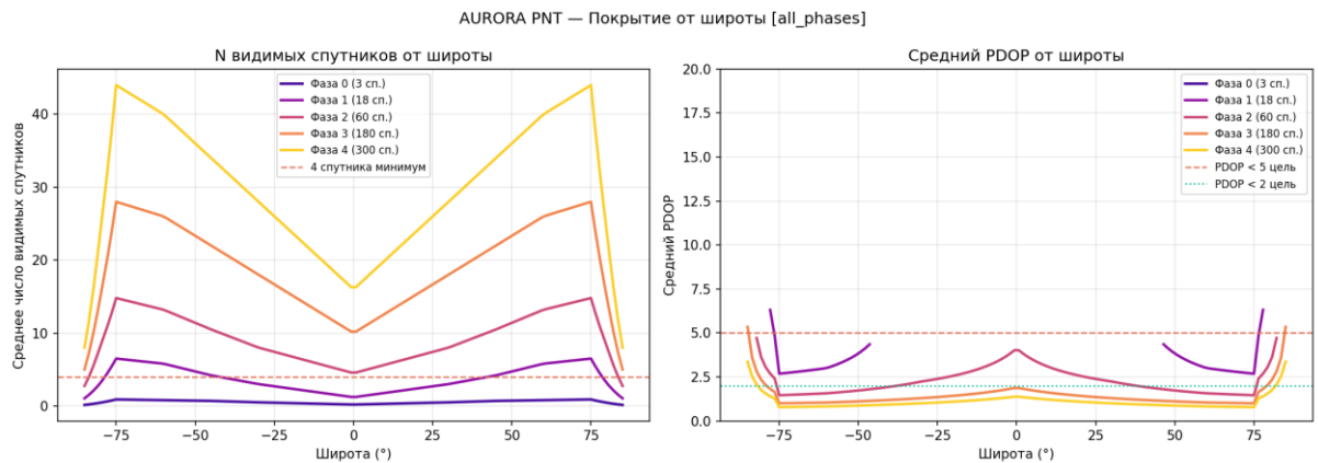
Рисунок 7 — Покрытие от широты
