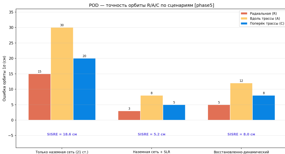
Рисунок 136 — Точность R/A/C по сценариям
