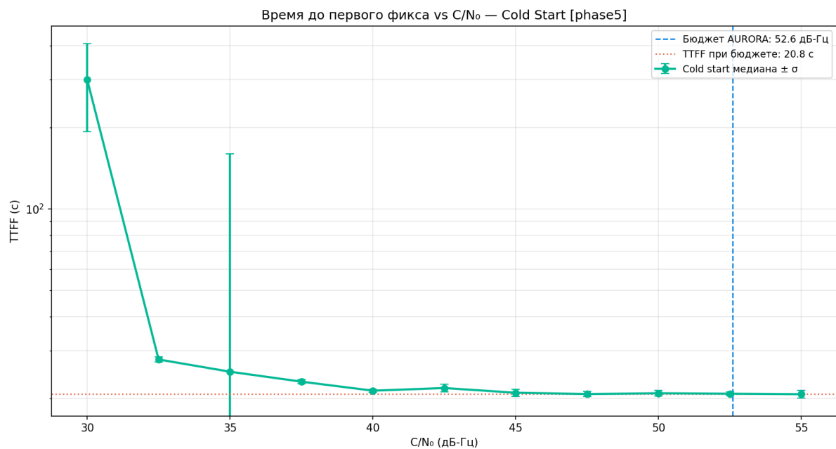
Рисунок 117 — TTFF vs C/N_0 (cold start)
