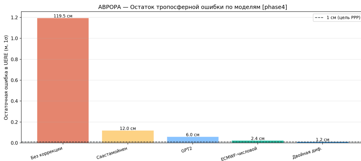
Рисунок 85 — Сравнение моделей коррекции
