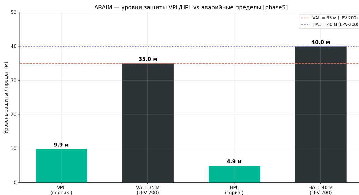
Рисунок 143 — VPL/HPL vs пределы
