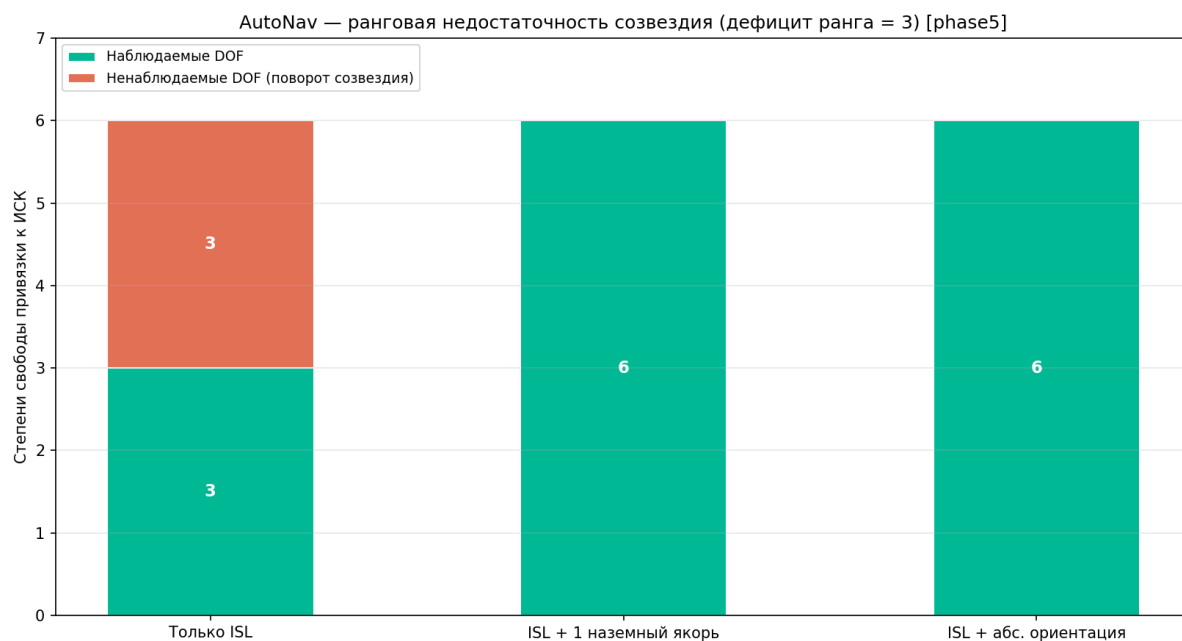
Рисунок 140 — Наблюдаемые/ненаблюдаемые DOF
