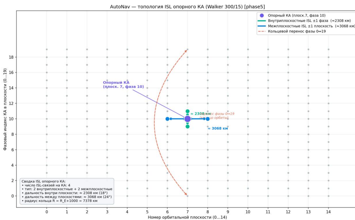
Рисунок 141 — Геометрия ISL-связей
