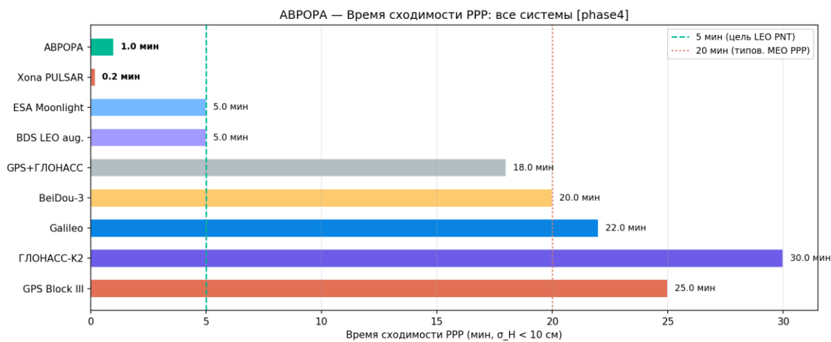
Рисунок 114 — Время сходимости PPP
