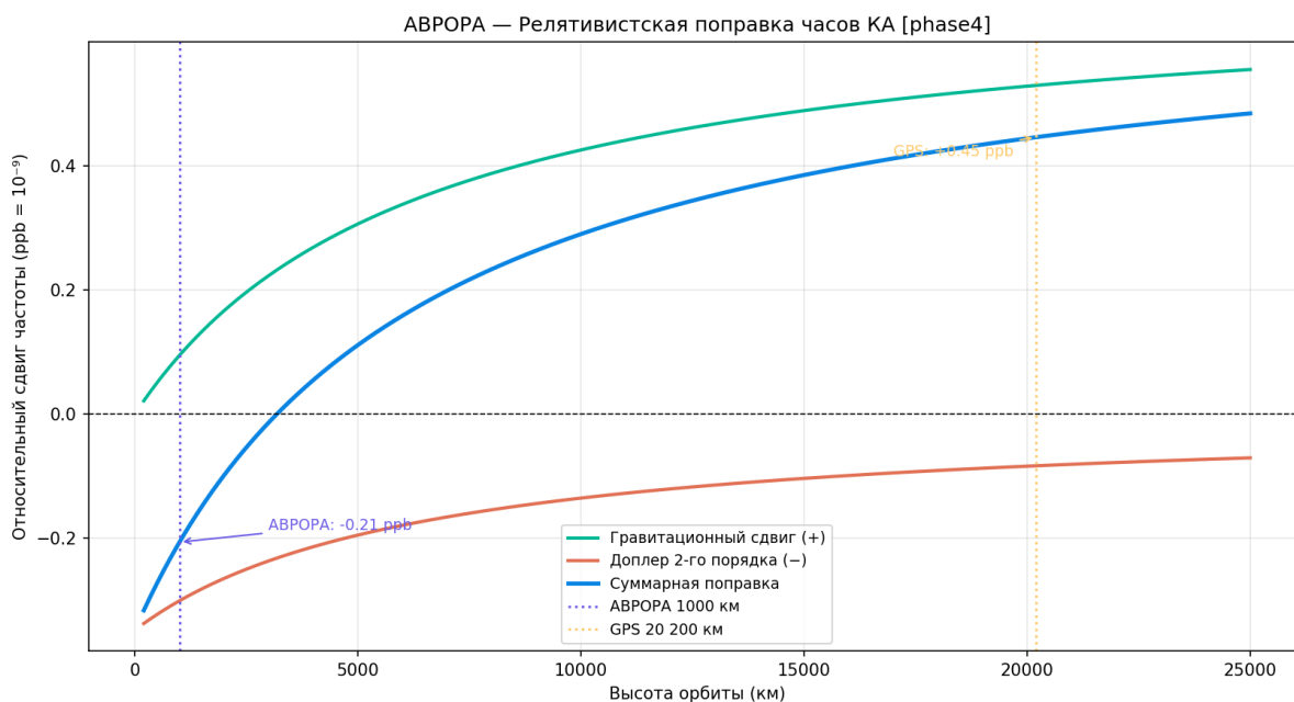
Рисунок 85 — Релятивистские поправки: часовой сдвиг
