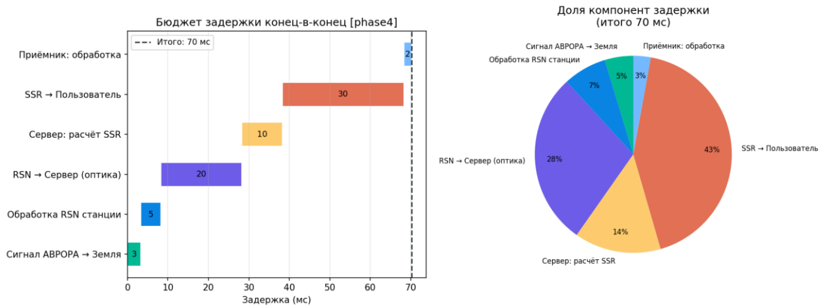
Рисунок 132 — Бюджет задержки E2E
