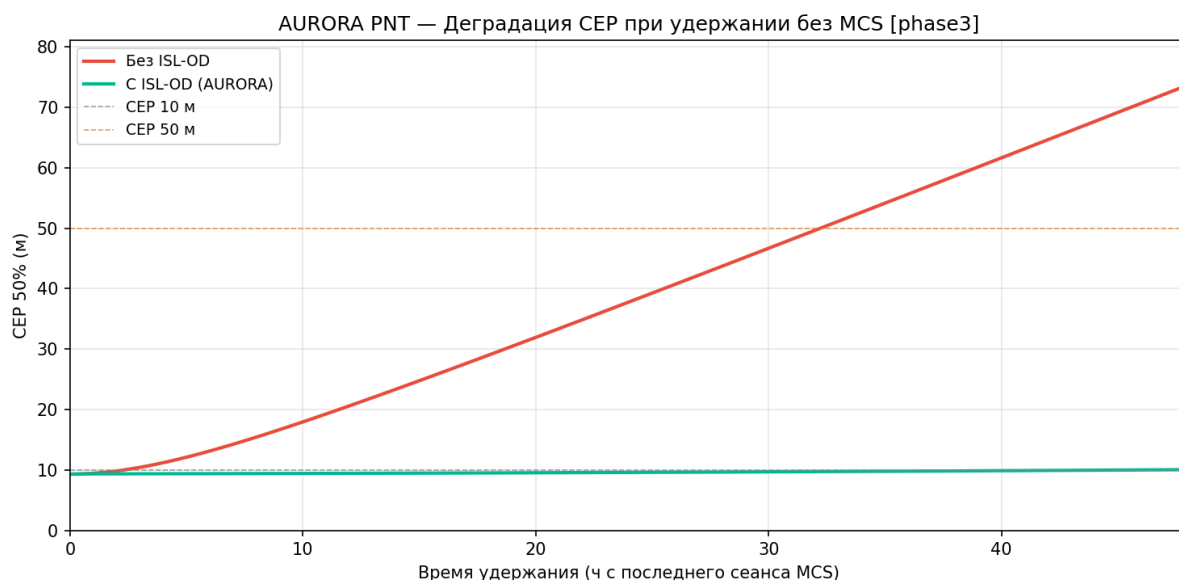
Рисунок 29 — ISL ухудшение CEP
