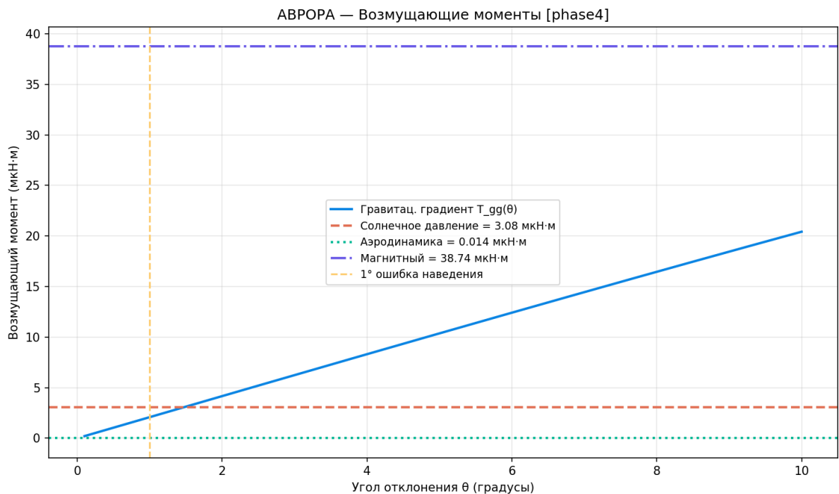
Рисунок 101 — Возмущающие моменты
