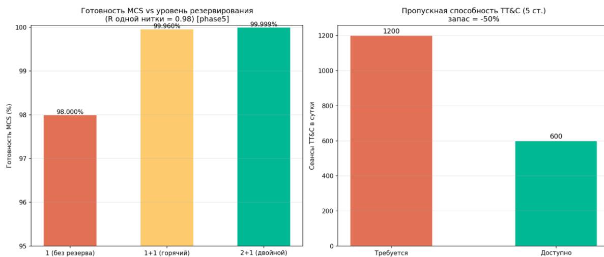
Рисунок 173 — Резервирование MCS
