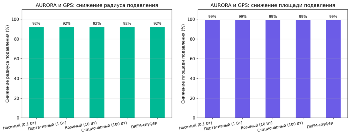
Рисунок 45 — Антиджамминг преимущество
