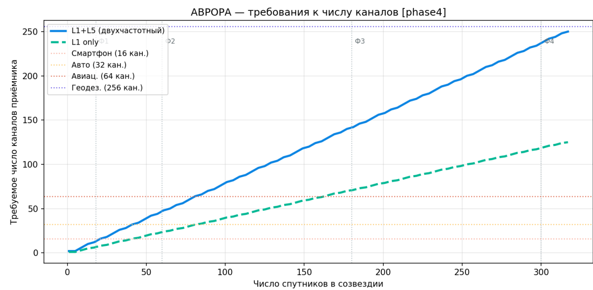
Рисунок 119 — Необходимое число каналов по фазам
