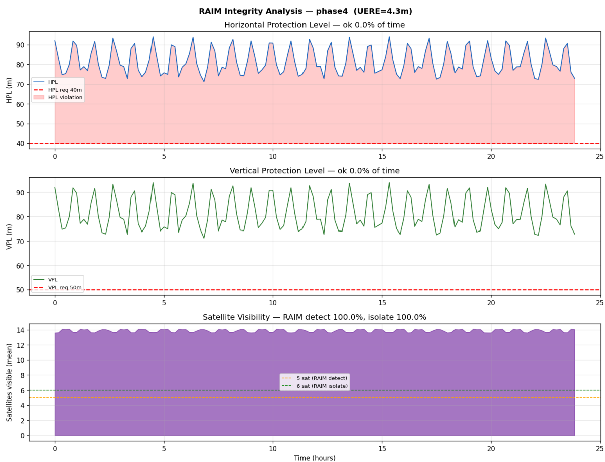
Рисунок 44 — RAIM доступность
