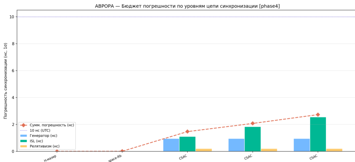
Рисунок 26 — Бюджет цепочки синхронизации
