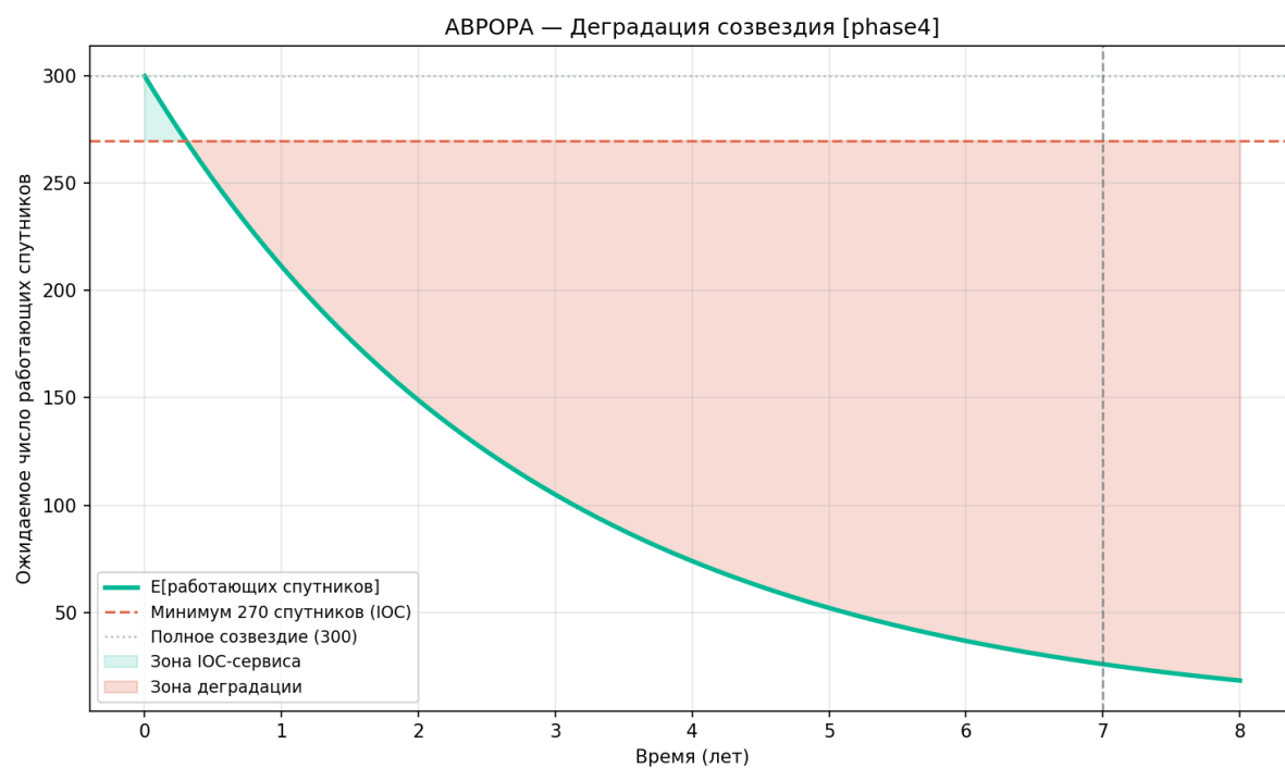
Рисунок 93 — Дegradация созвездия
