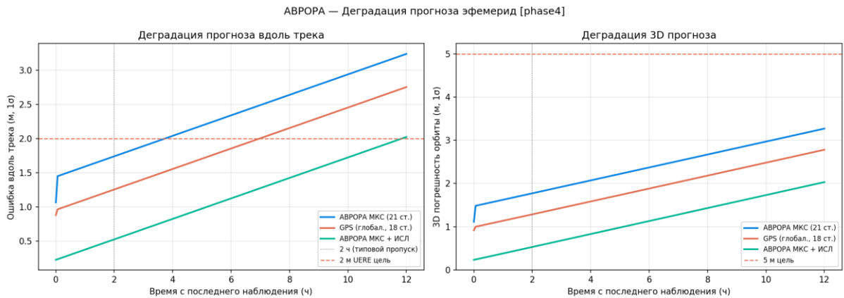
Рисунок 42 — Деградация прогноза эфемерид
