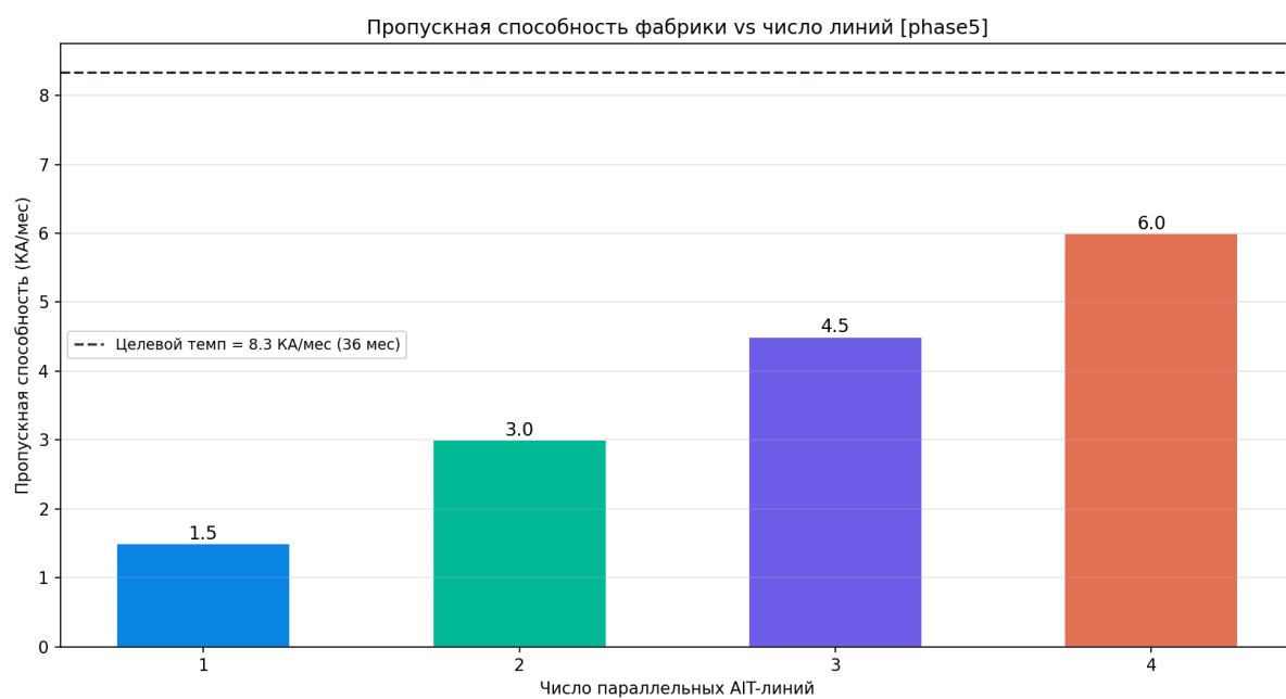
Рисунок 165 — Пропускная способность завода
