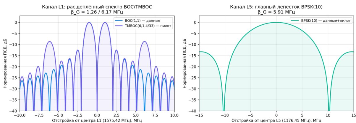
Рисунок 19 — Спектр рекомендованного сигнала АВРОРА: ПСД каналов L1 (BOC/TMBOC) и L5 (BPSK(10))
