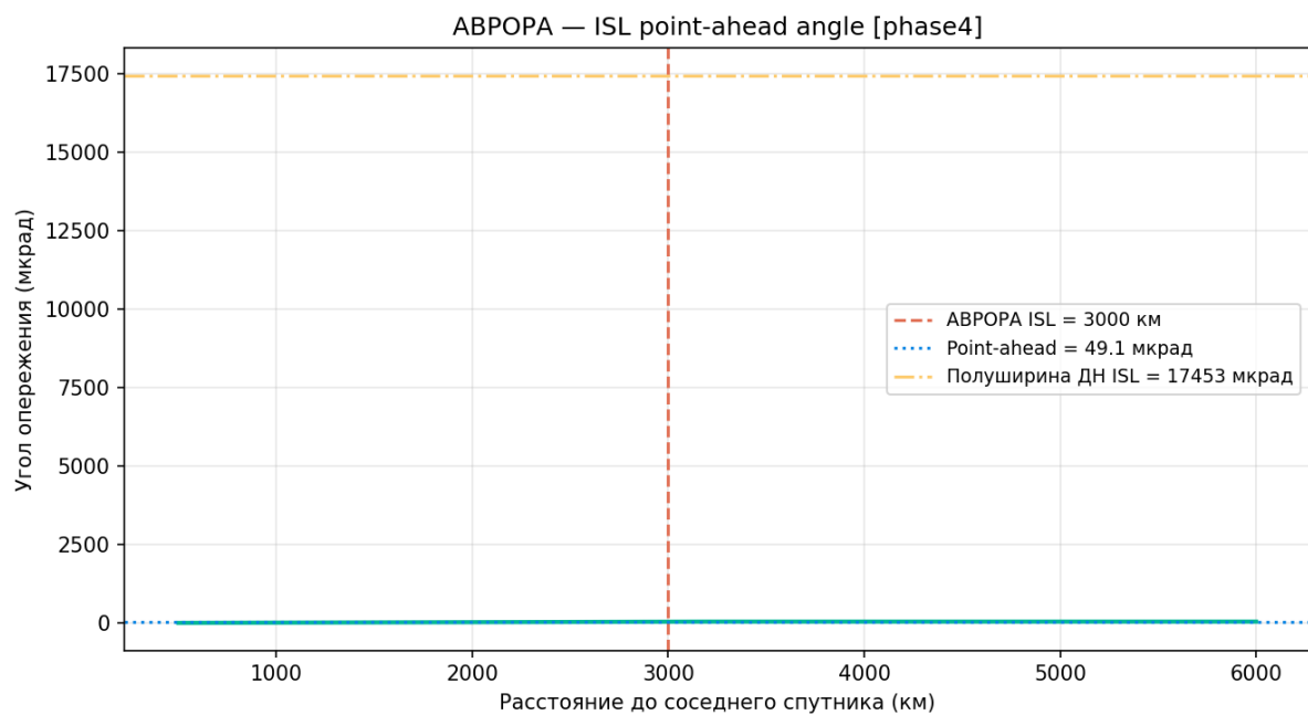
Рисунок 103 — ISL point-ahead angle
