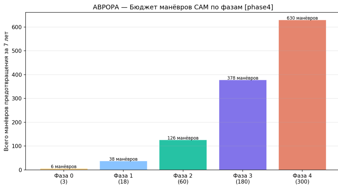
Рисунок 65 — Бюджет манёвров САМ
