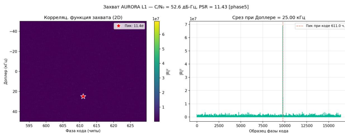
Рисунок 122 — 2D корреляц. функция захвата
