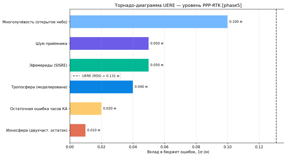
Рисунок 135 — Tornado-вклад UERE
