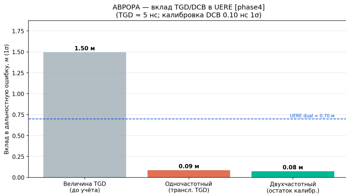
Рисунок 100 — Вклад TGD/DCB в UERE
