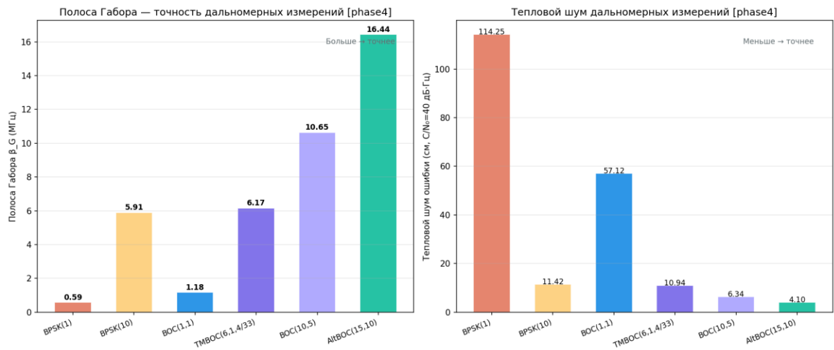
Рисунок 14 — Ширина полосы Габора по модуляциям
