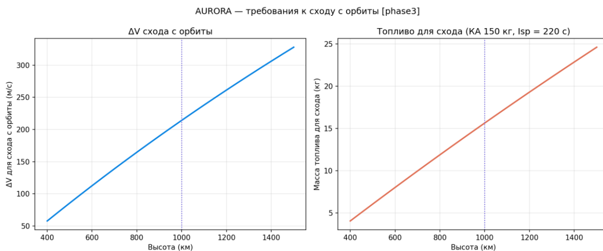
Рисунок 62 — \Delta V схода с орбиты
