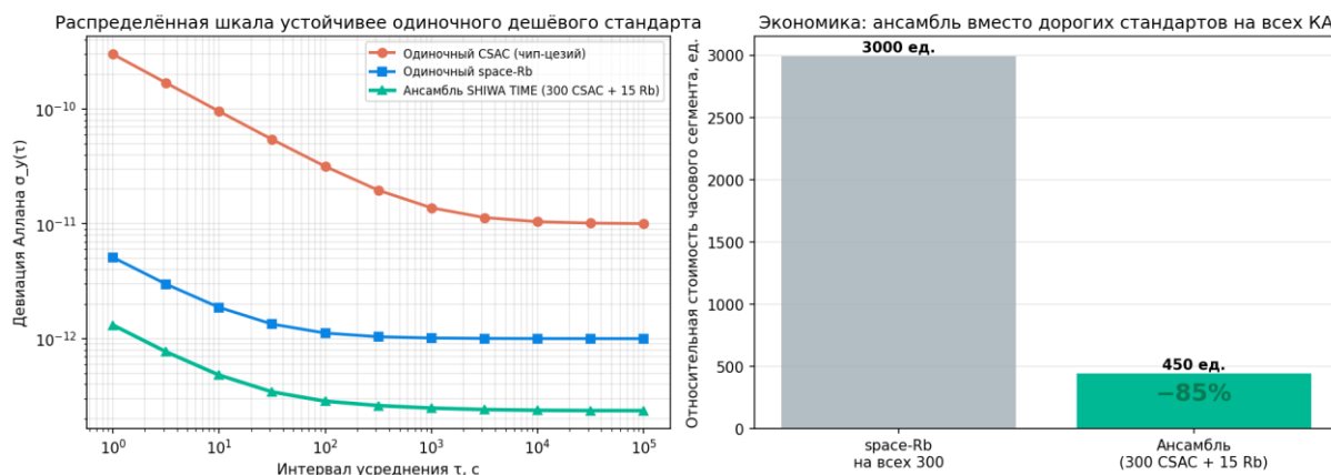
Рисунок 76 — SHIWA TIME-Space: ансамблевый эталон и экономика
