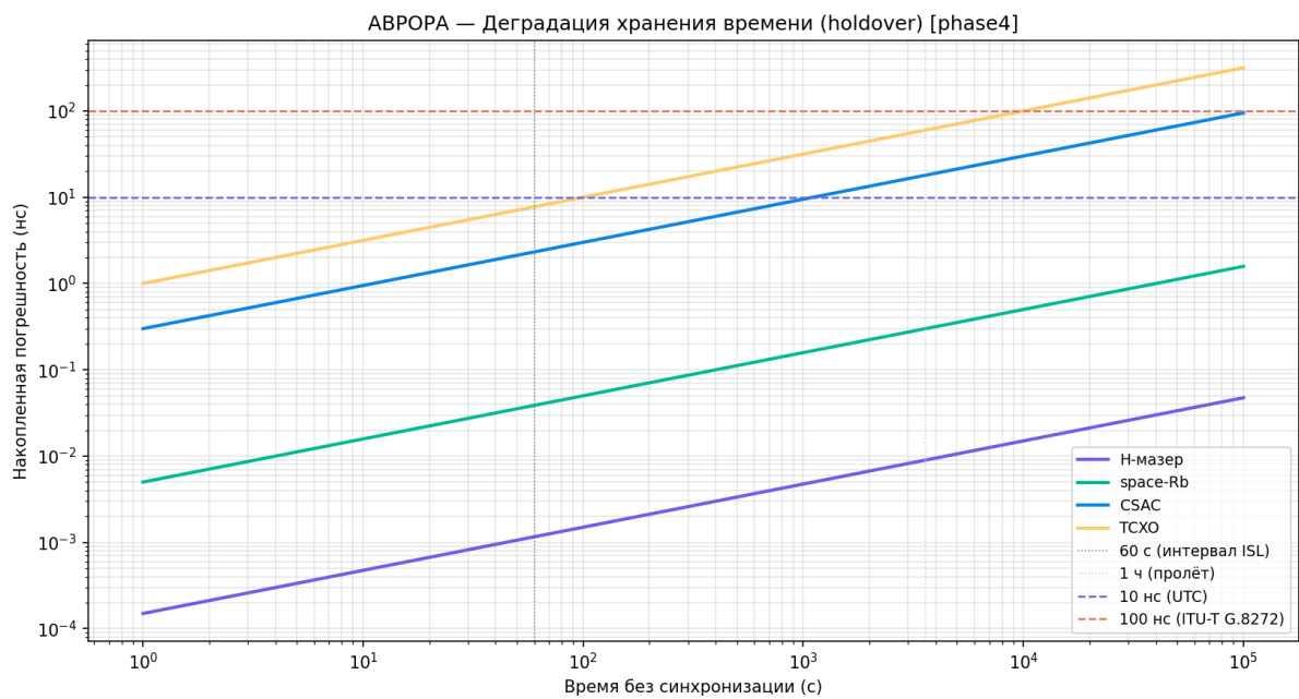
Рисунок 25 — Удержание синхронизации
