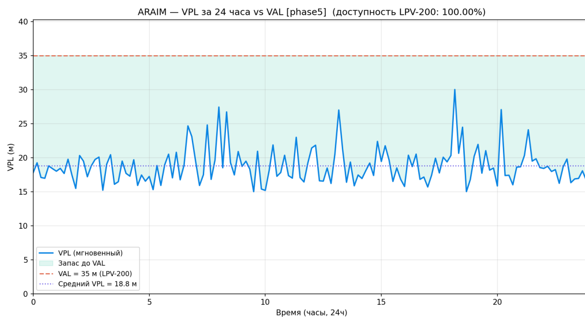
Рисунок 154 — VPL за сутки
