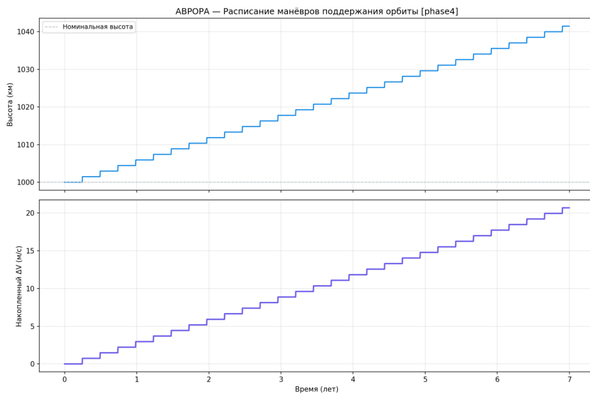
Рисунок 110 — Расписание манёвров
