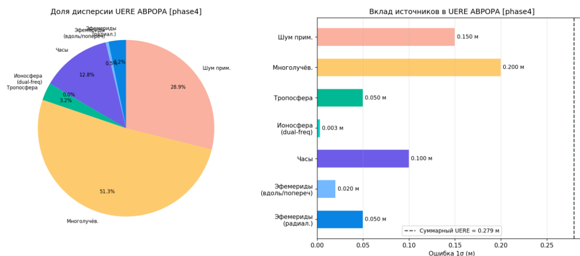
Рисунок 98 — Бюджет UERE ABPOPA
