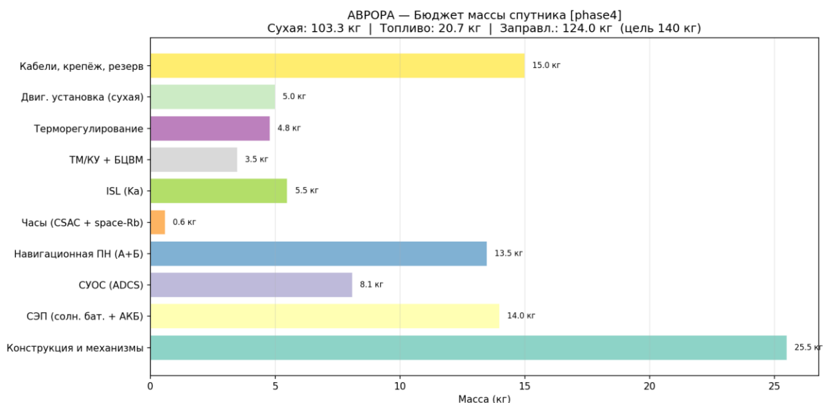
Рисунок 55 — Распределение масс
