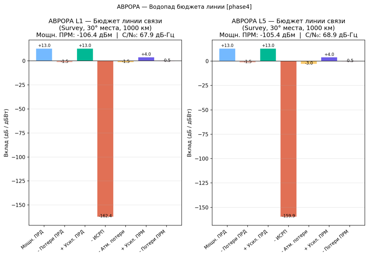
Рисунок 32 — Бюджет линии: составляющие
