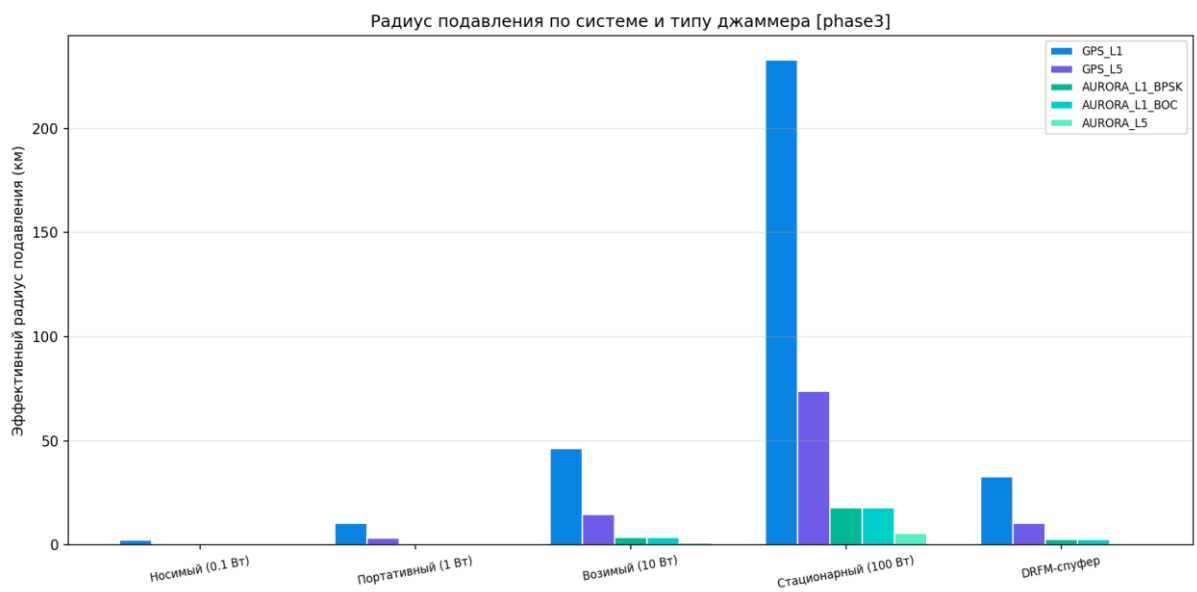
Рисунок 46 — Радиус зоны подавления
