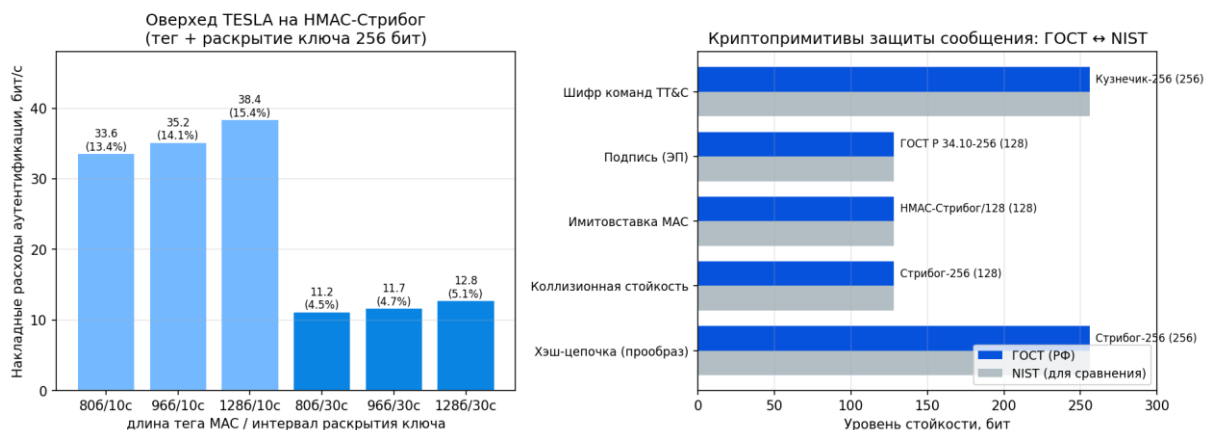
Рисунок 49 — Криптозащита навигационного сообщения на ГОСТ
