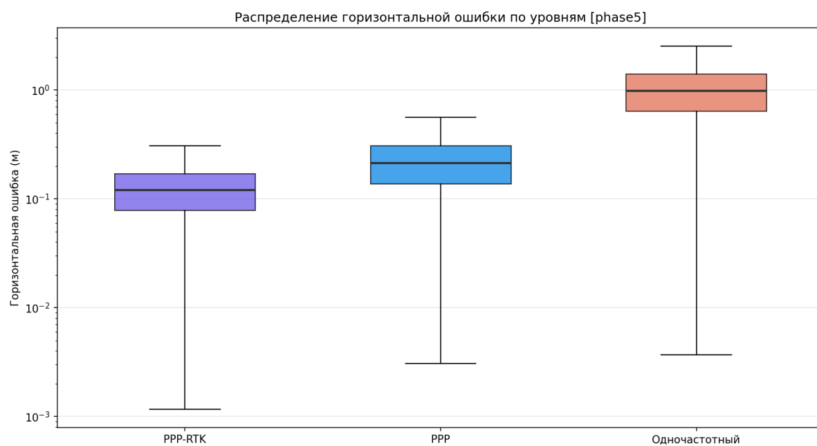
Рисунок 137 — Распределение ошибки по классам
