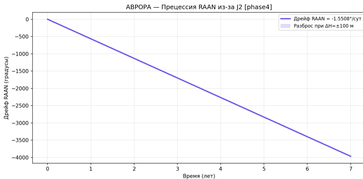
Рисунок 108 — Прецессия RAAN
