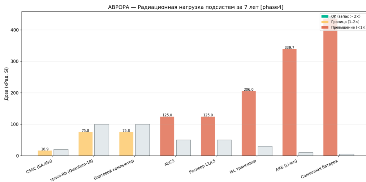
Рисунок 83 — Радиационная нагрузка подсистем
