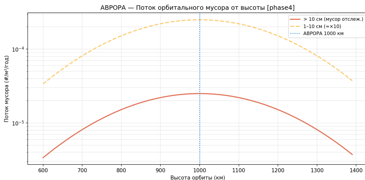
Рисунок 63 — Поток мусора vs высота
