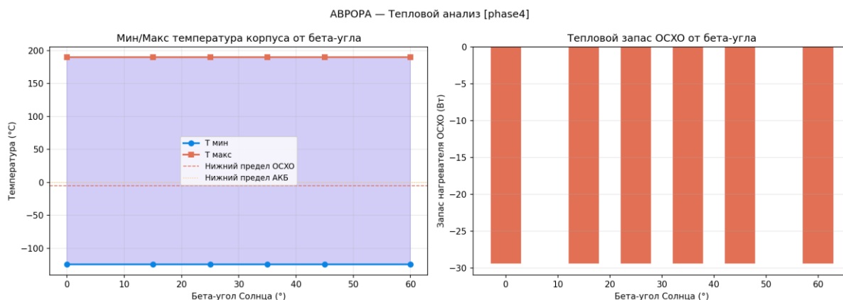
Рисунок 58 — Тепловой режим vs бета-угол
