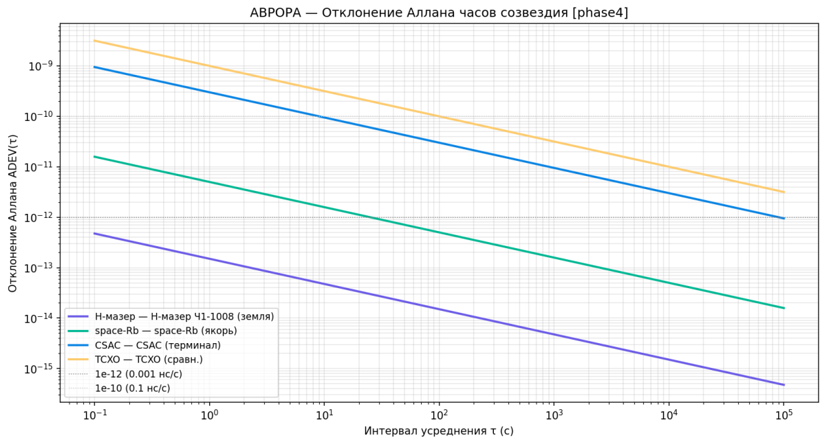
Рисунок 23 — ADEV — все типы часов
