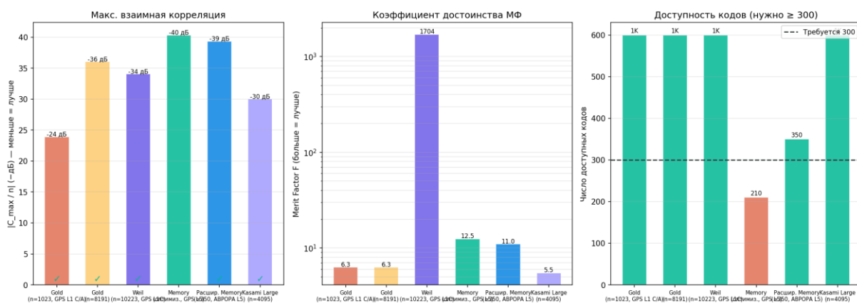
Рисунок 16 — Семейства кодов: Merit Factor и взаимная корреляция
