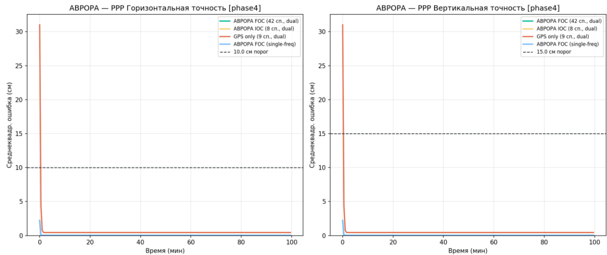
Рисунок 94 — Сравнение сходимости PPP
