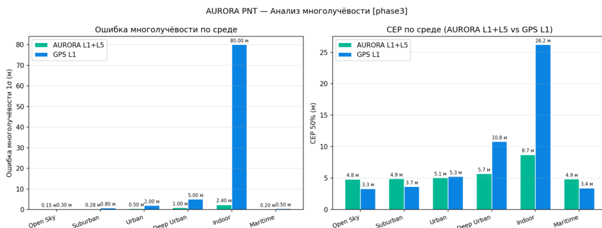
Рисунок 50 — Многолучёвость: ошибка
