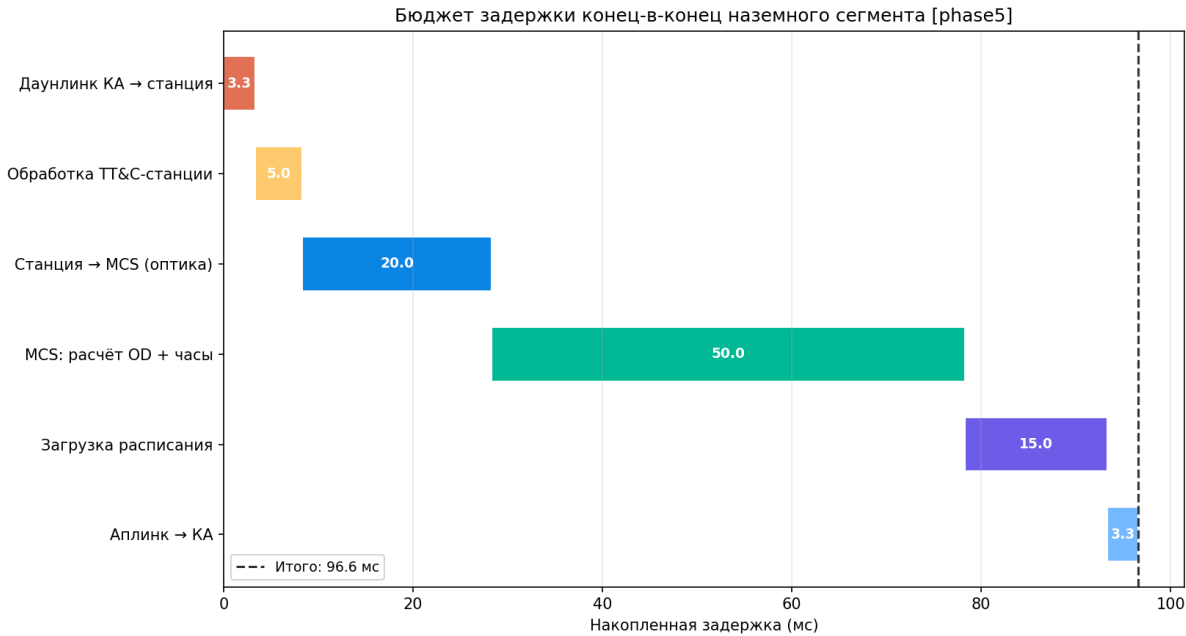
Рисунок 172 — Бюджет задержки
