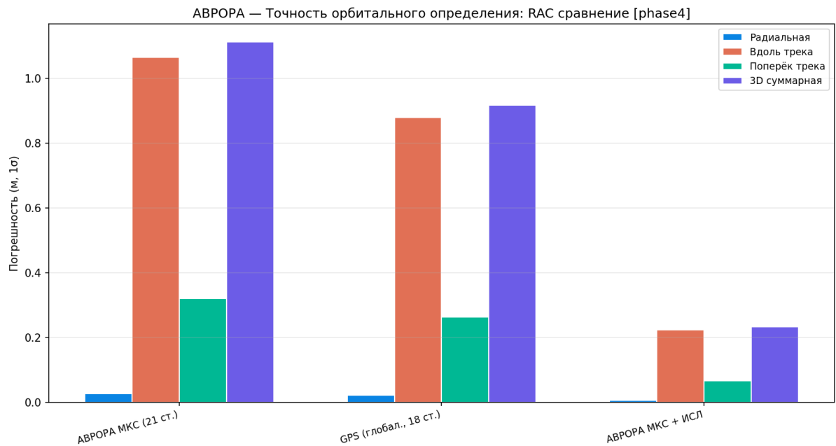
Рисунок 41 — Сравнение RAC ошибок
