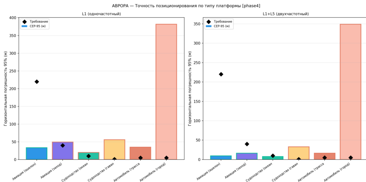
Рисунок 38 — Точность позиционирования по платформам
