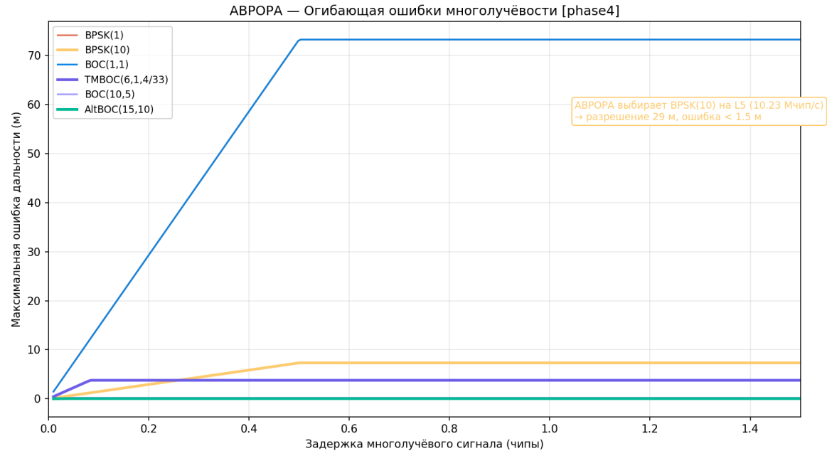
Рисунок 15 — Огибающая многолучёвости по модуляциям
