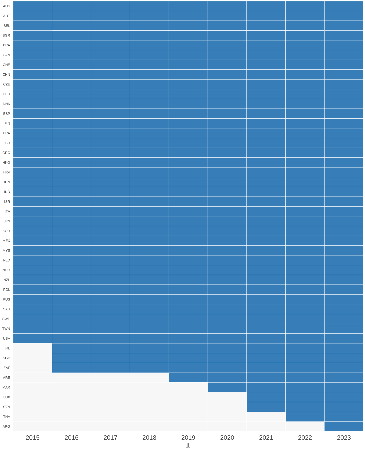
TOP500 2023
