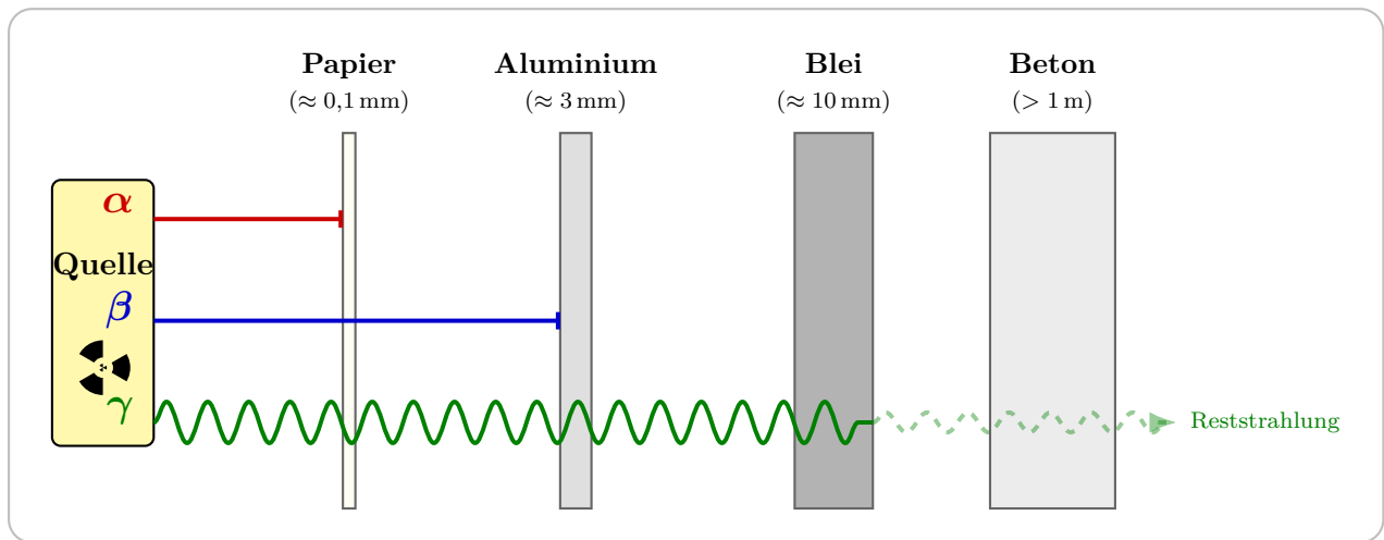
Abbildung 1: Abschirmung und Durchdringungsvermögen der drei Strahlungsarten.
