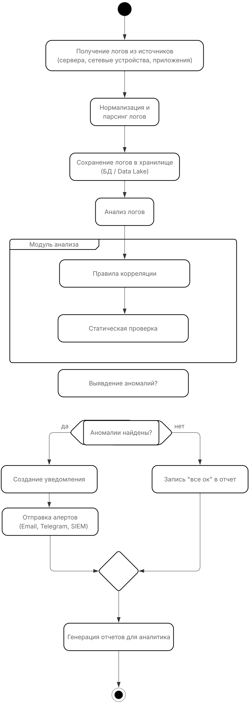
Диаграмма активности: Анализ логов и обнаружение аномалий
