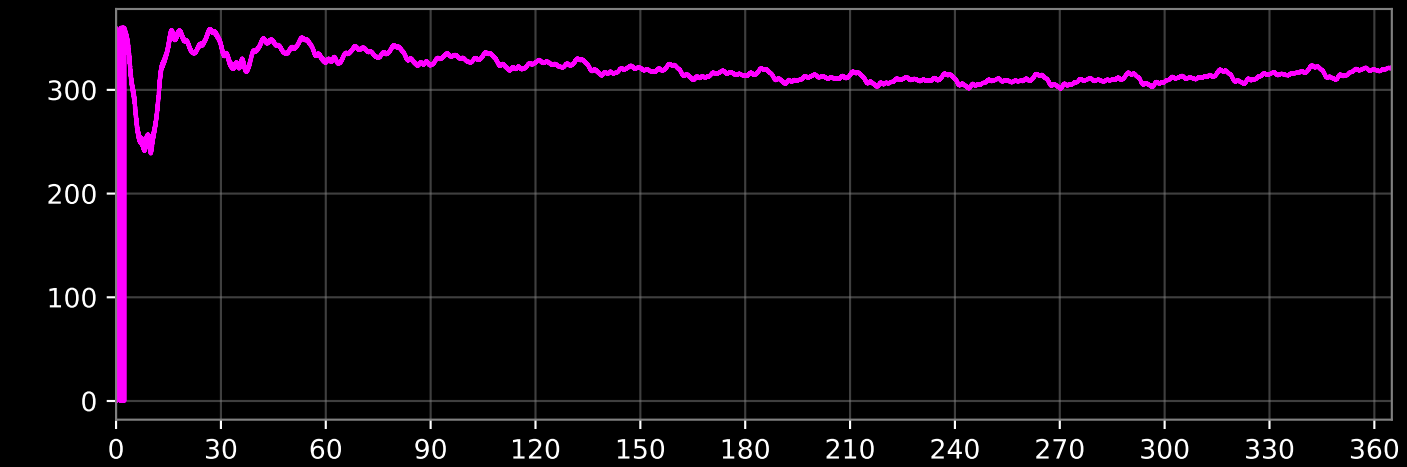
Perigee argument ( \omega , grader)
