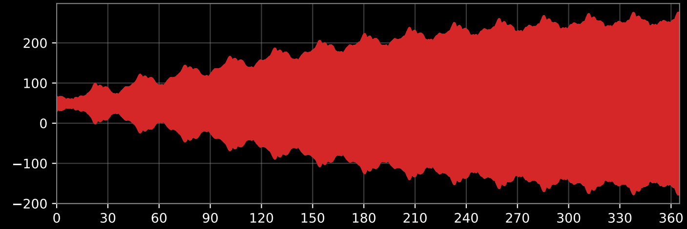
Inklinasjon (i, grader)
