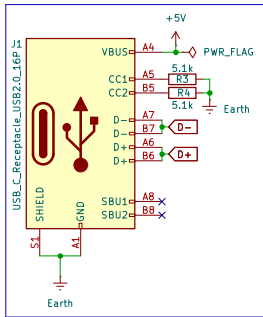
USB-C
