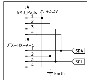
Extencion IMU
