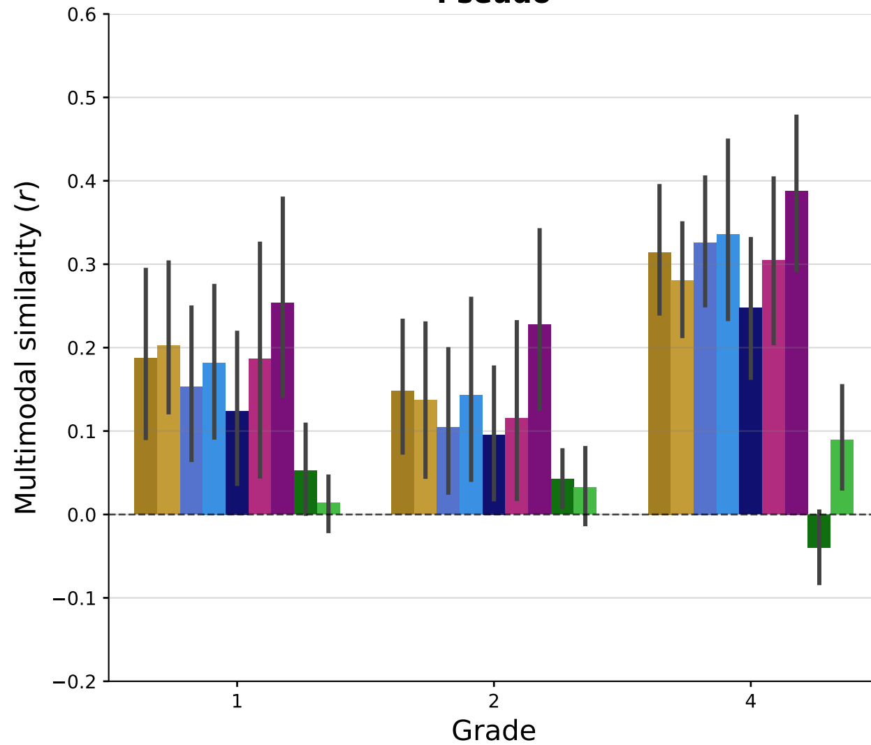
Pseudo
