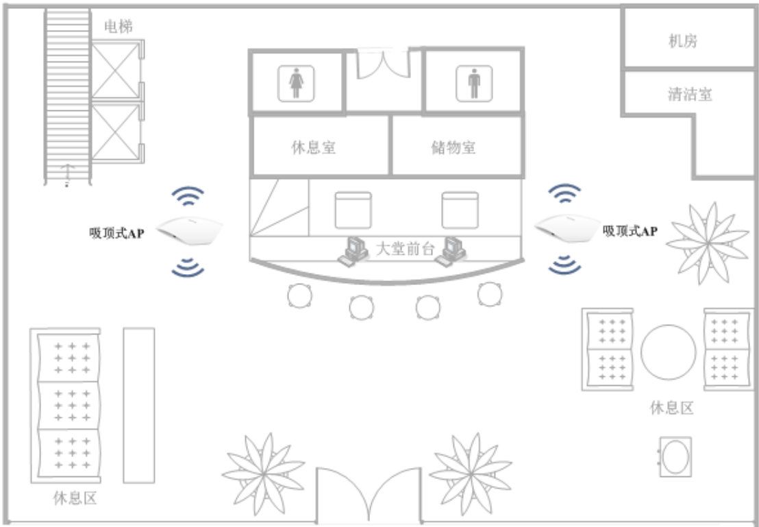
图 2 酒店大堂无线 AP 安装部署
