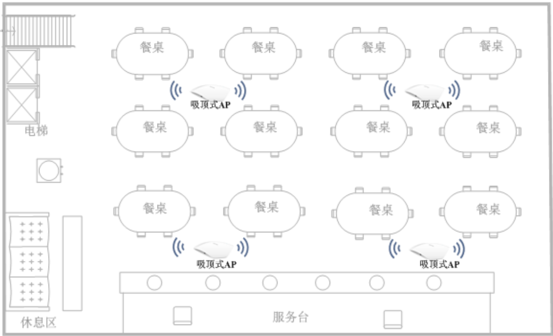
图 3 酒店餐厅无线 AP 安装部署
