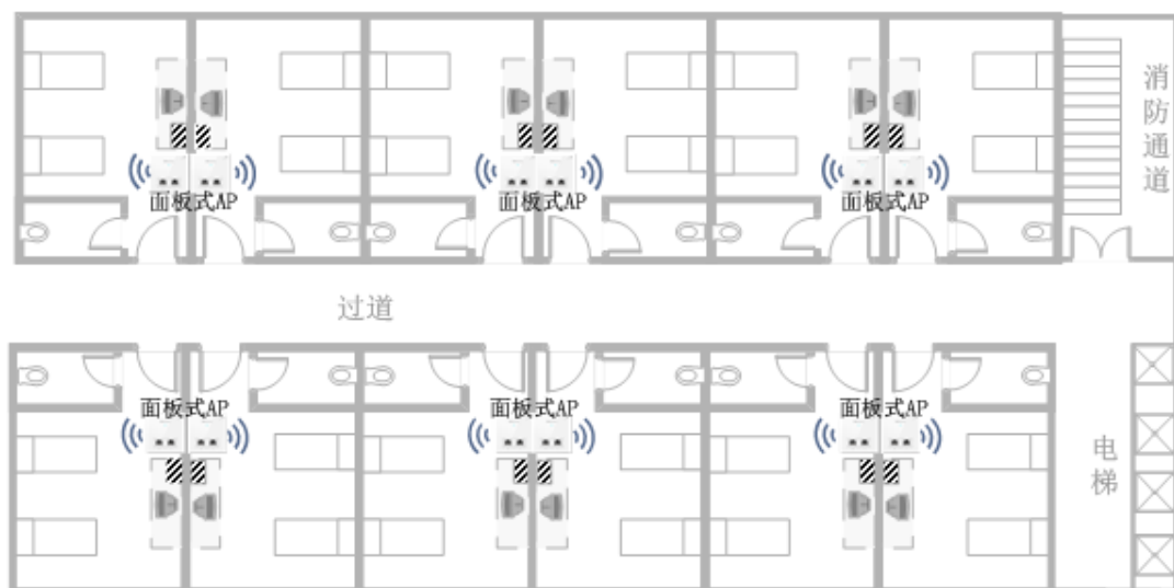
图 4 酒店客户无线 AP 安装部署
