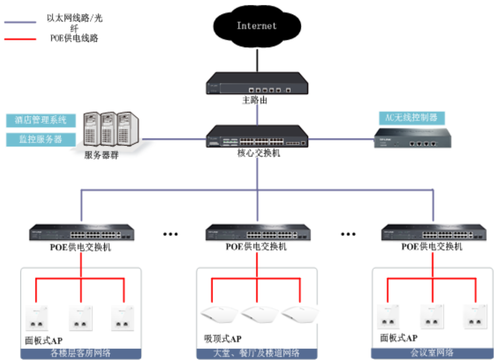
图 1 无线 AP 应用案例-酒店网络拓扑图
