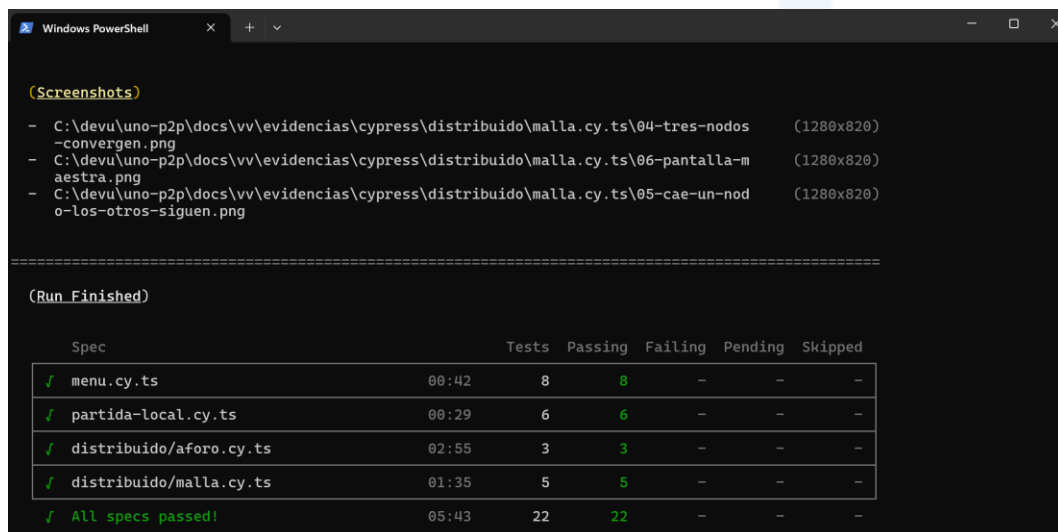
Figura 10. La suite completa ejecutándose en consola: los cuatro archivos, 22 pruebas, 22 pasadas, 0 fallos, en 5 minutos y 43 segundos.
