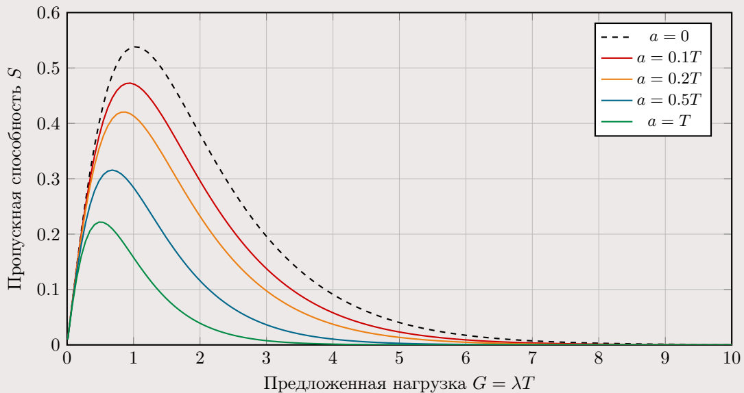
Зависимость пропускной способности от нагрузки (при T = 1 )
