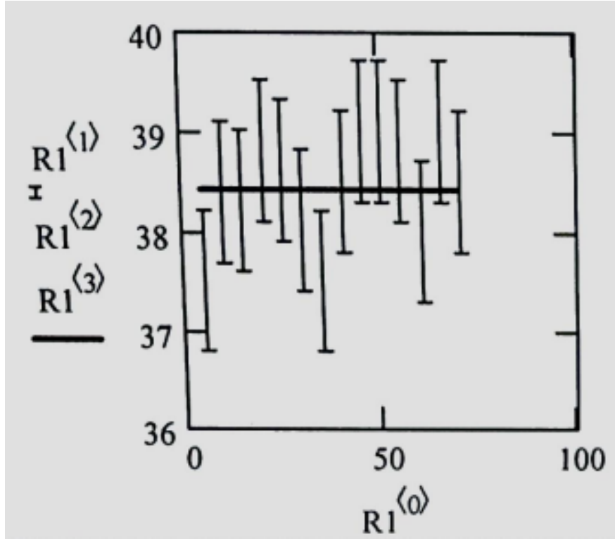
Рис. 5: Преломляющий угол призмы
