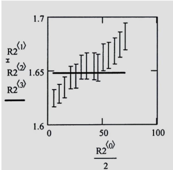
Рис. 6: Зависимость n_o от угла падения \theta
