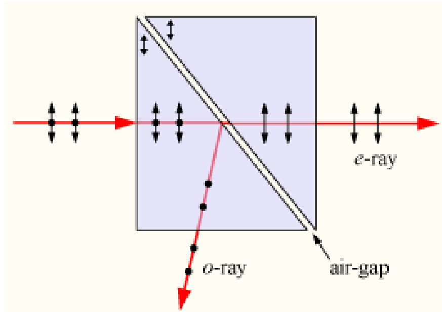
Рис. 8: Поляризация света в призме Глана
