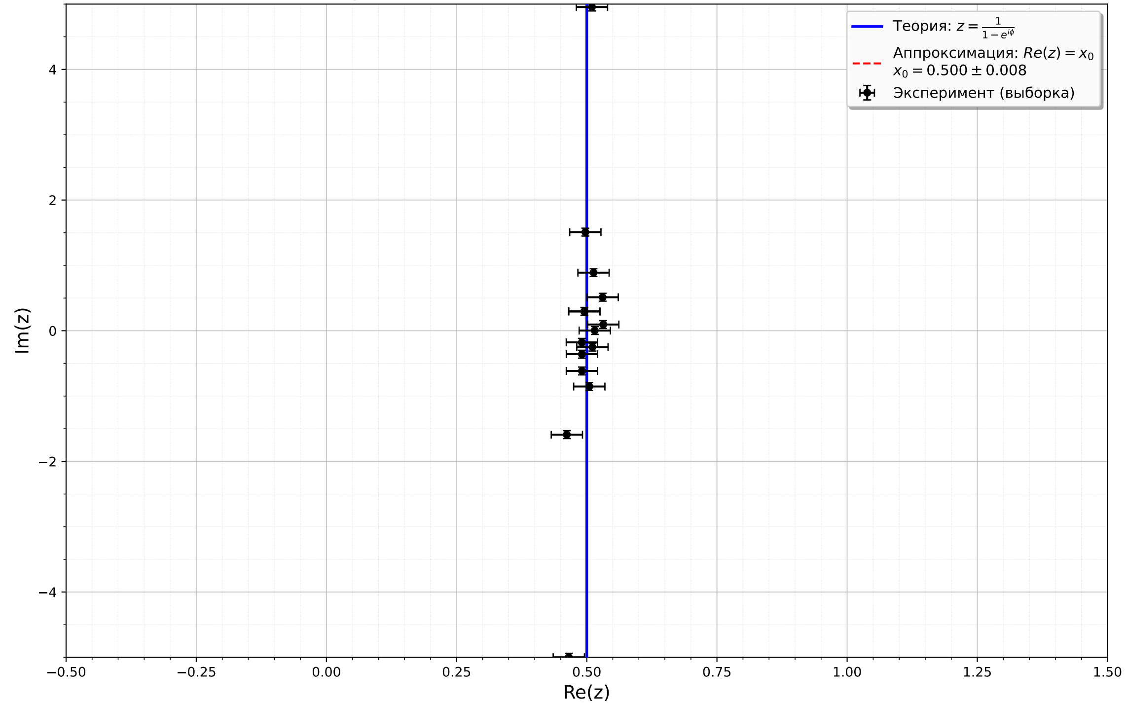
Кривая 1/(1 - e^{i\phi}) на комплексной плоскости
