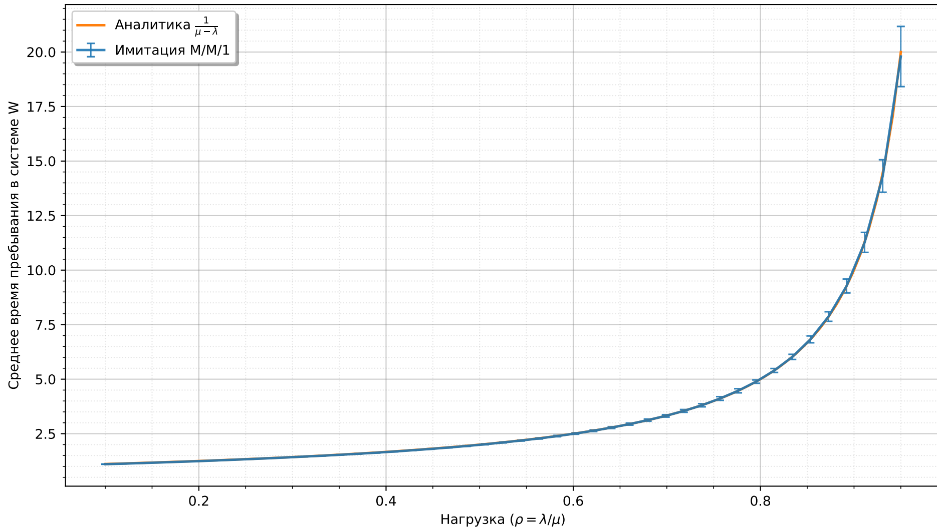
Зависимость времени пребывания от нагрузки (М/М/1)
