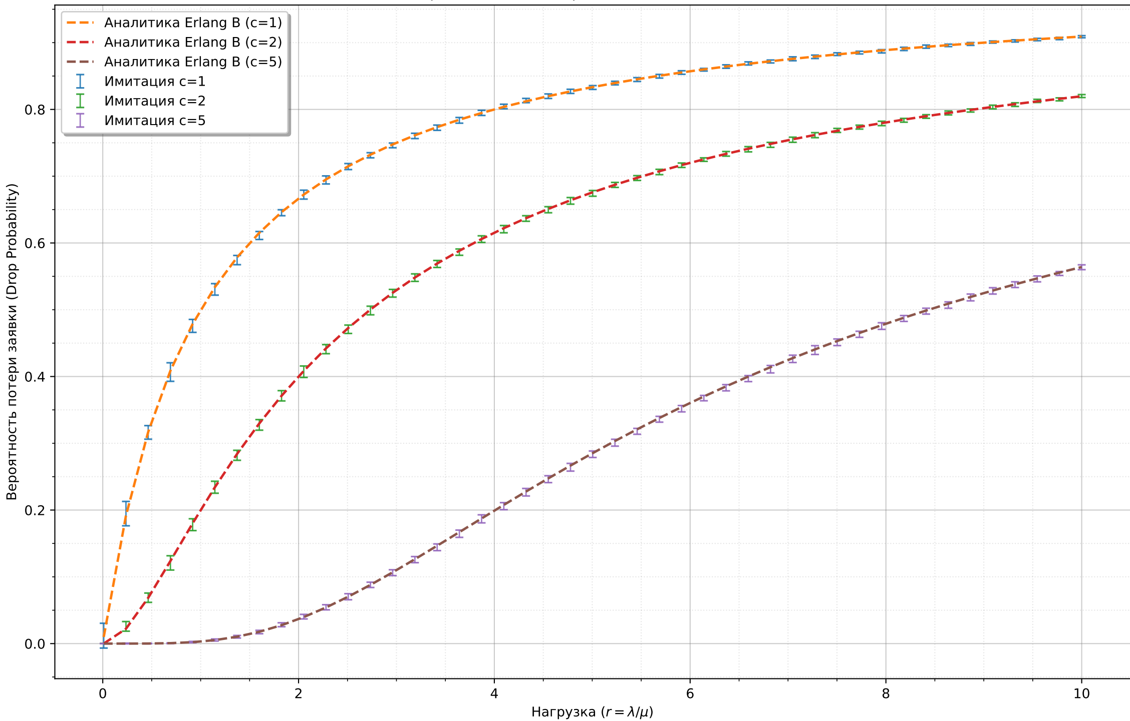
Вероятность блокировки в системе М/М/с/с
