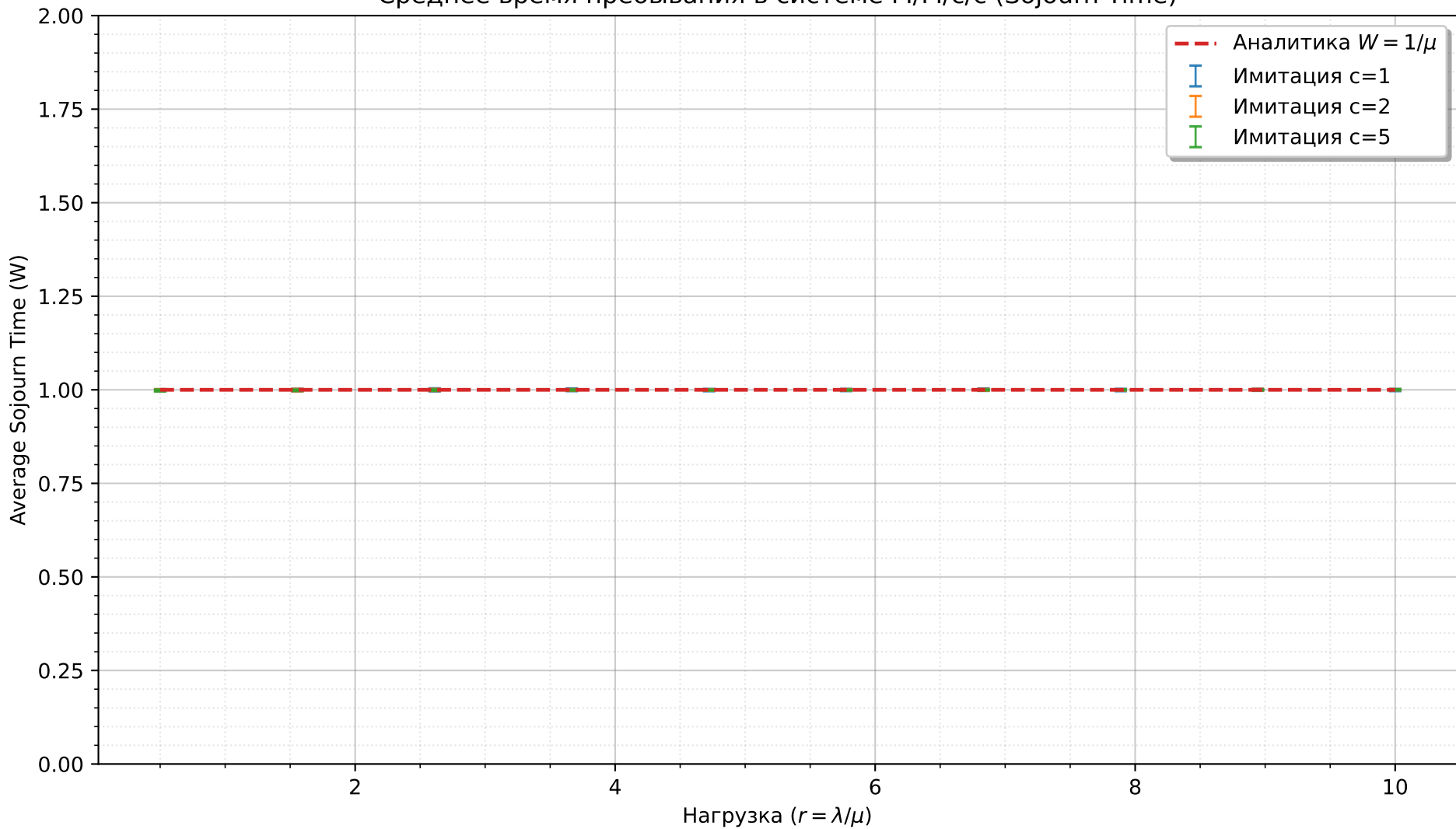
Среднее время пребывания в системе М/М/с/с (Sojourn Time)
