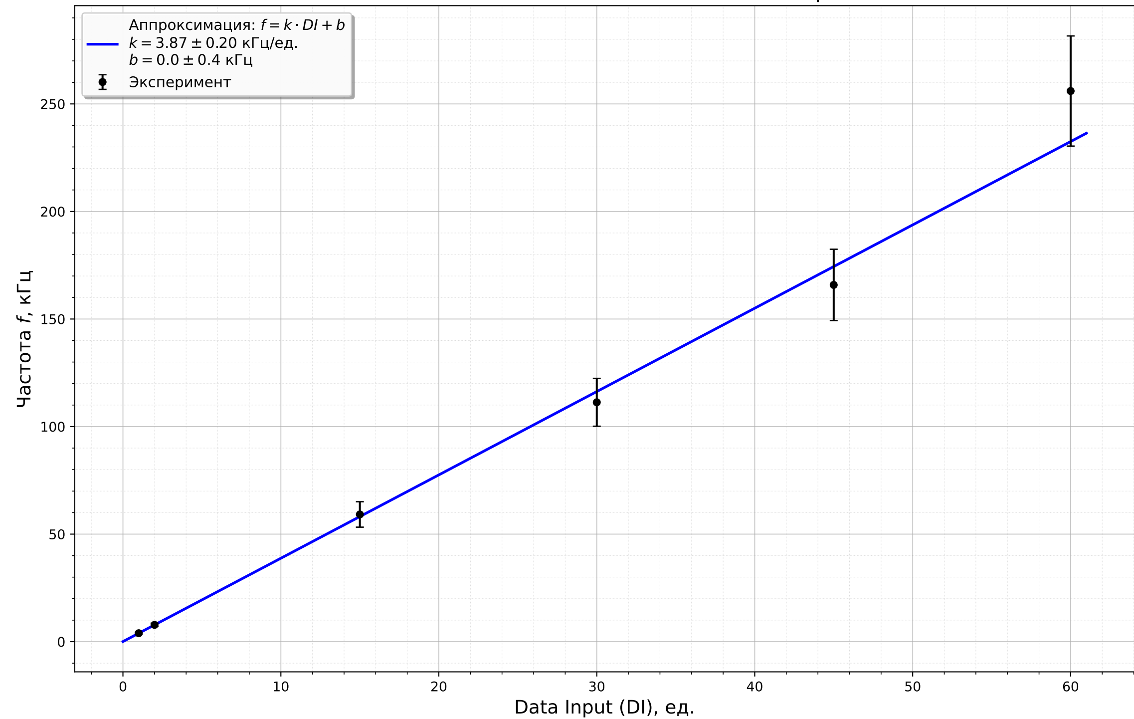
Зависимость частоты сигнала от Data Input
