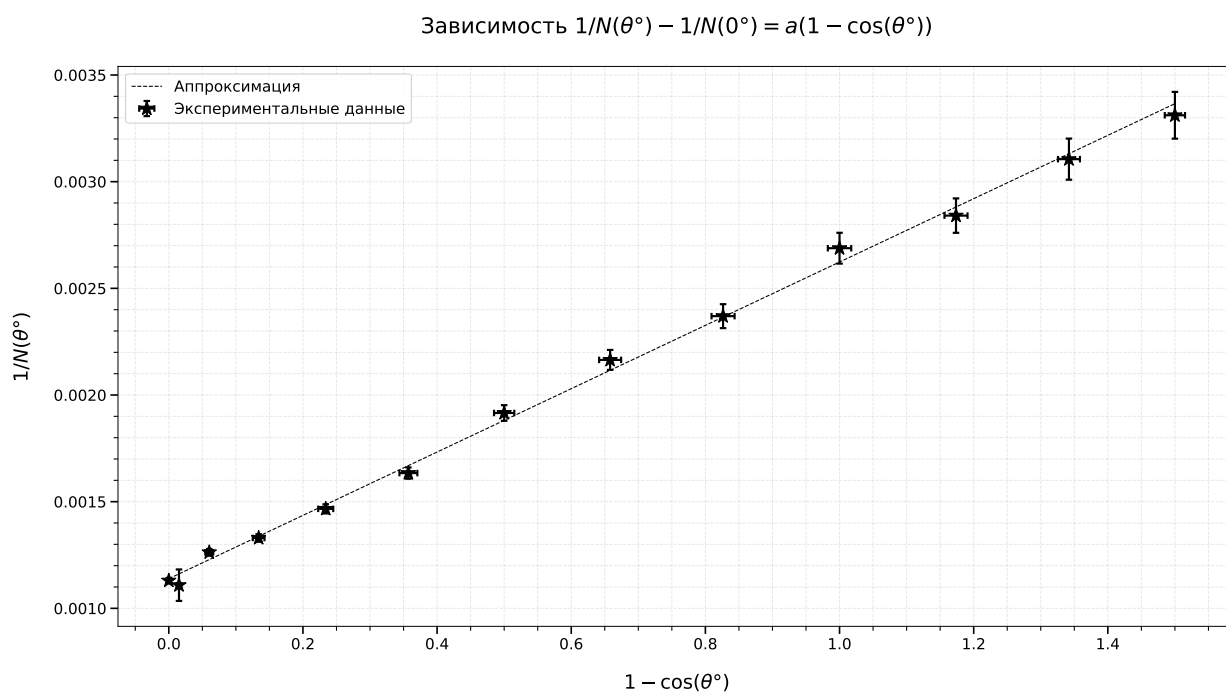
Рис. 1: Проверка соотношения для эффекта Комптона
