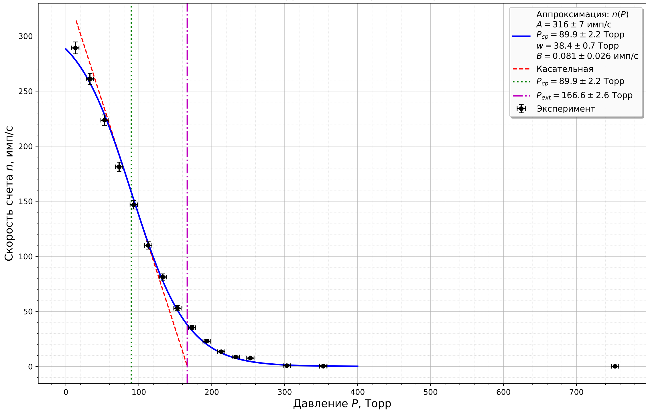
Зависимость счета от давления (Сцинтилляционный счетчик)
