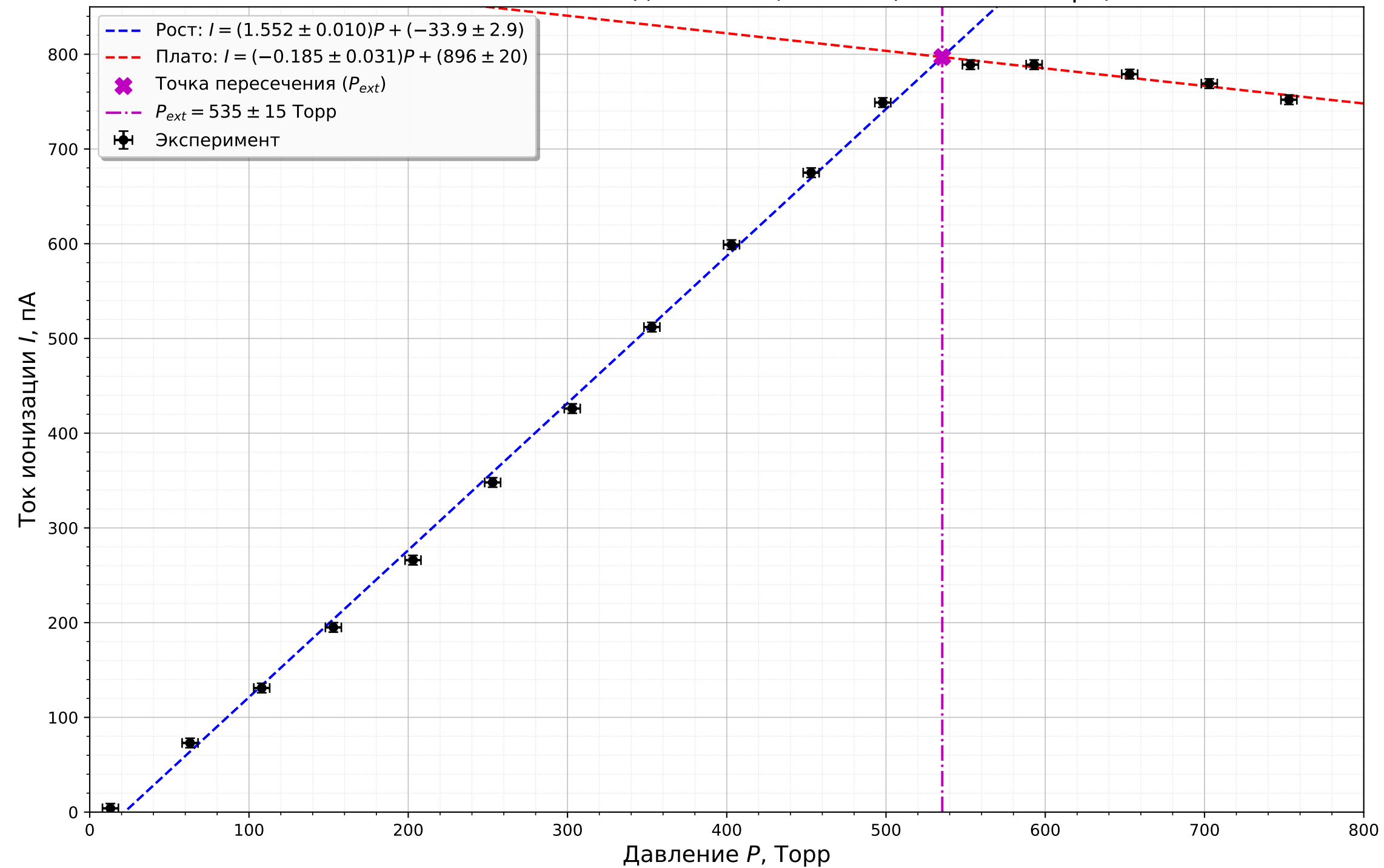
Зависимость тока от давления (Ионизационная камера)
