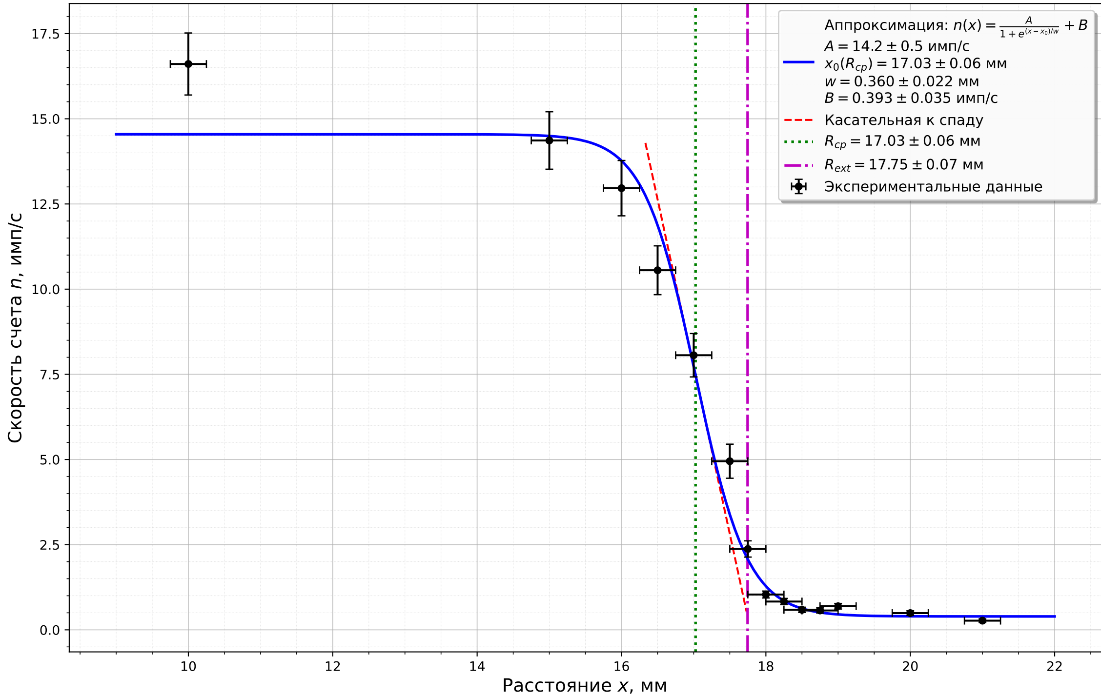
Кривая поглощения \alpha -частиц в воздухе (Счетчик Гейгера)
