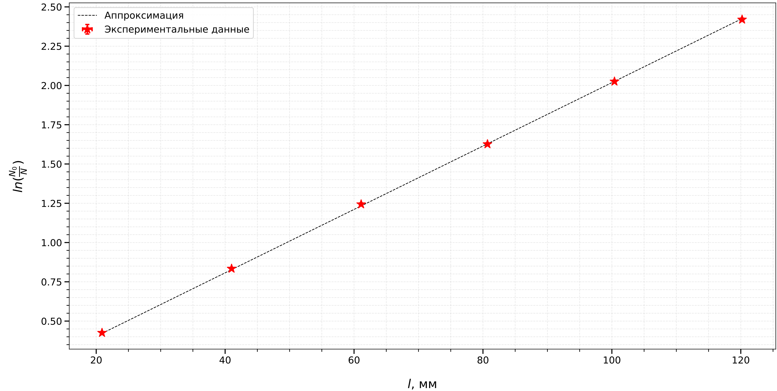
Зависимость \ln(\frac{N_0}{N}) = f(l) для алюминия
