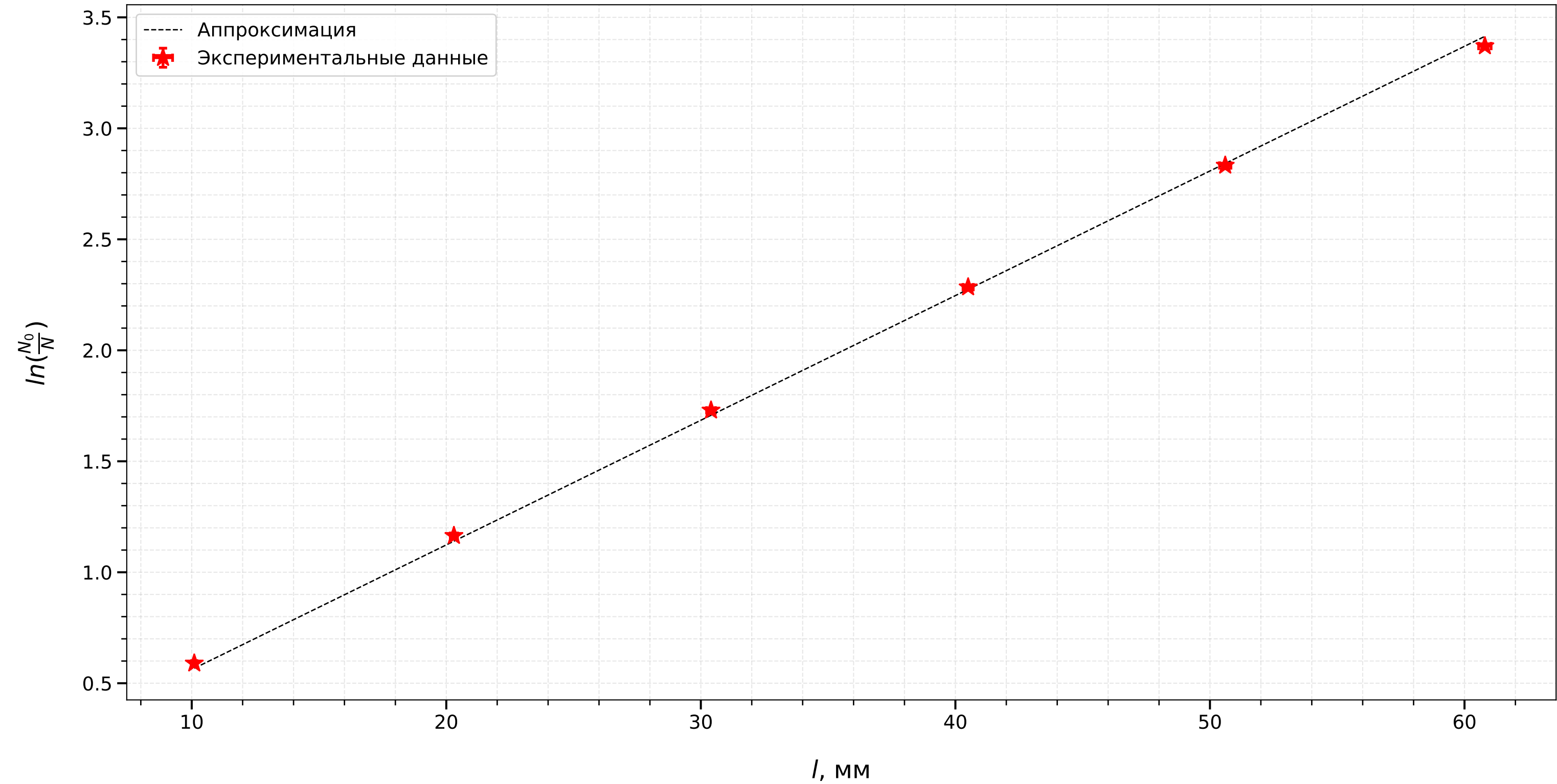
Зависимость \ln(\frac{N_0}{N}) = f(l) для железа
