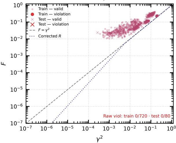
QAOA p=3
