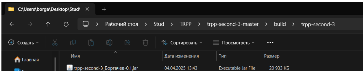
Рисунок 13 – Пример jar-файла
