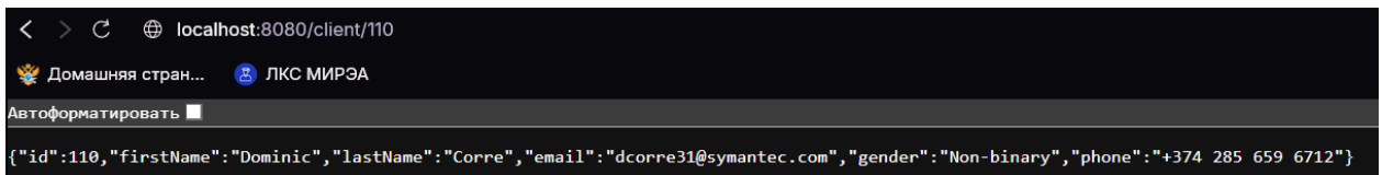
Рисунок 11 – Запрос клиента по идентификатору
