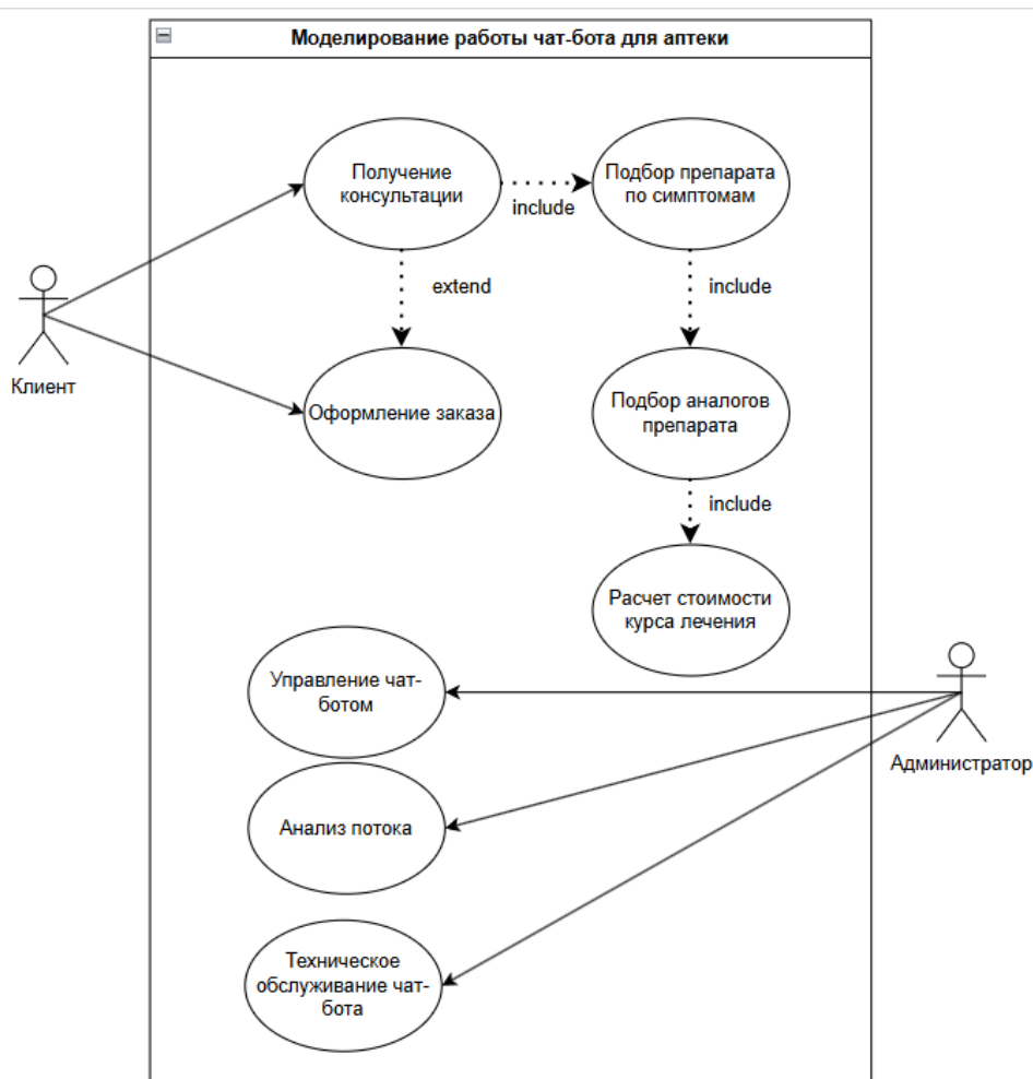
Рисунок 2 – Диаграмма вариантов использования системы «Моделирование работы чат-бота для аптеки»
