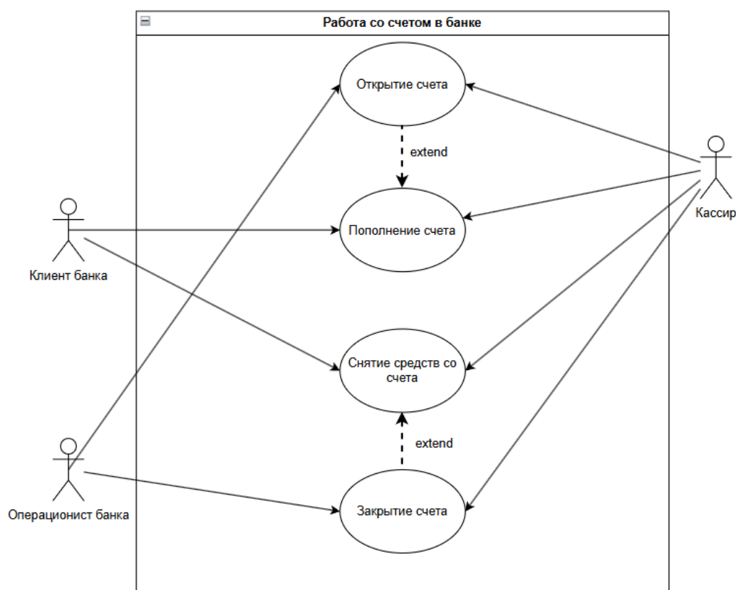
Рисунок 1 – Диаграмма вариантов использования
