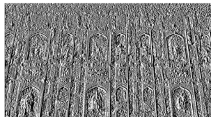
Gradient X
