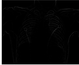
Gradient X
