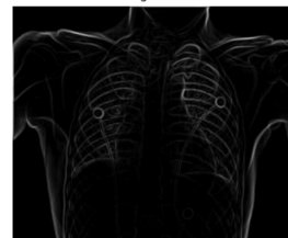
Magnitude
