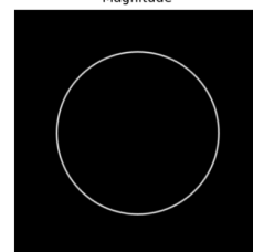
Magnitude
