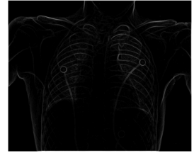
Magnitude
