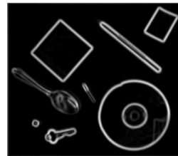
Magnitude
