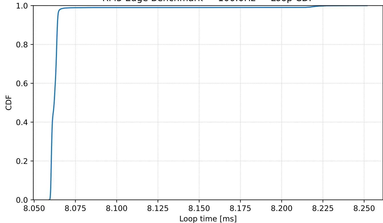
RPi5 Edge Benchmark — 100.0Hz — Loop CDF
