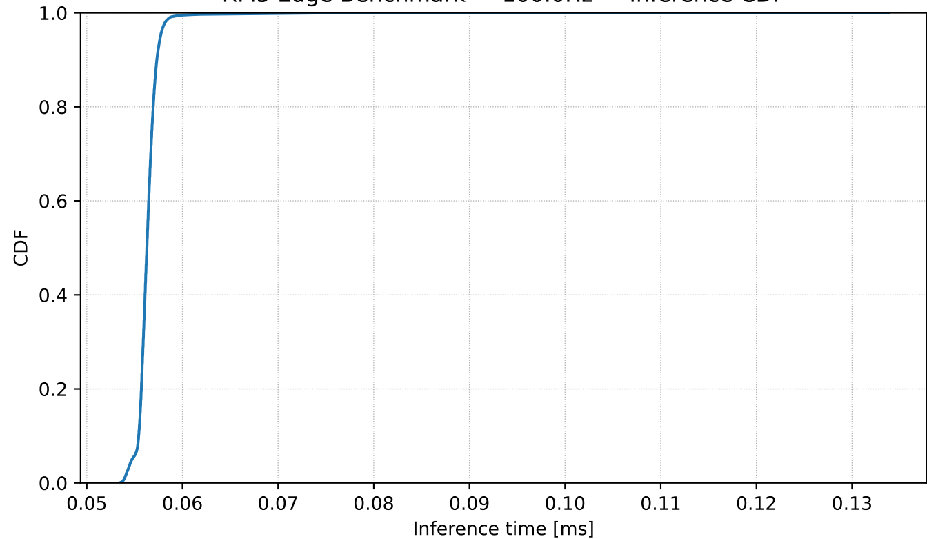
RPi5 Edge Benchmark — 100.0Hz — Inference CDF
