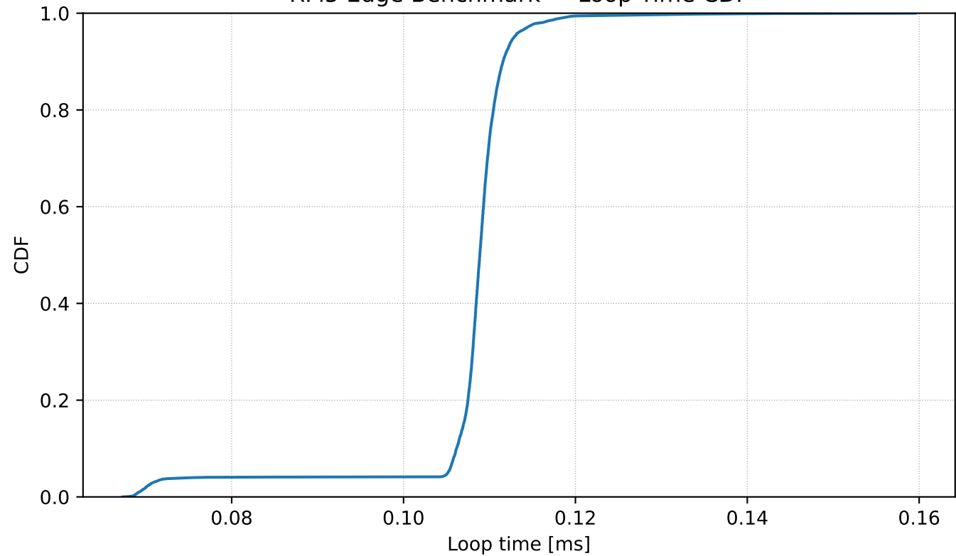
RPi5 Edge Benchmark — Loop Time CDF
