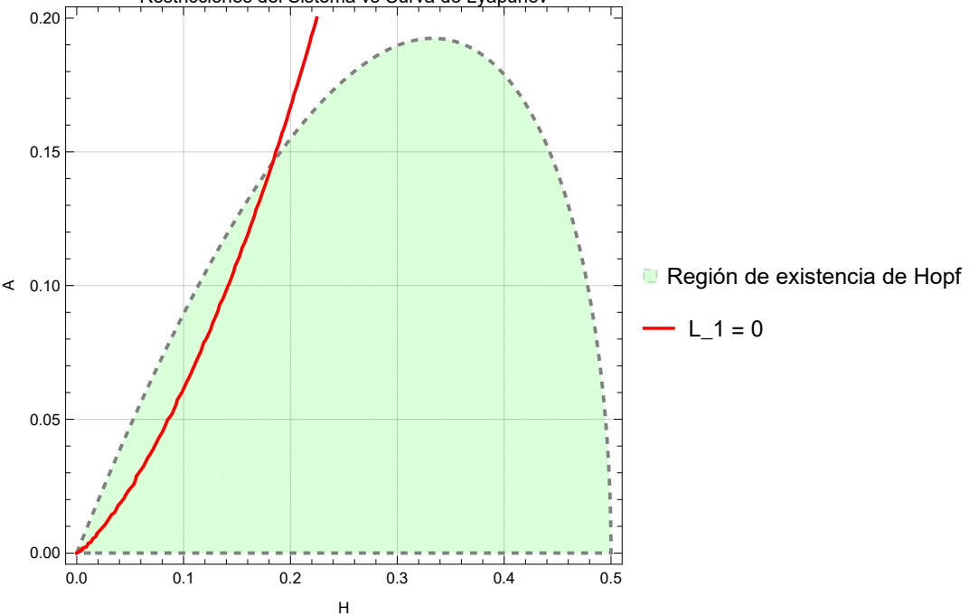
Restricciones del Sistema vs Curva de Lyapunov
