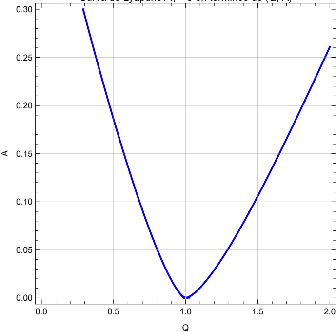
Curva de Lyapunov I_1 = 0 en términos de (Q, A)
