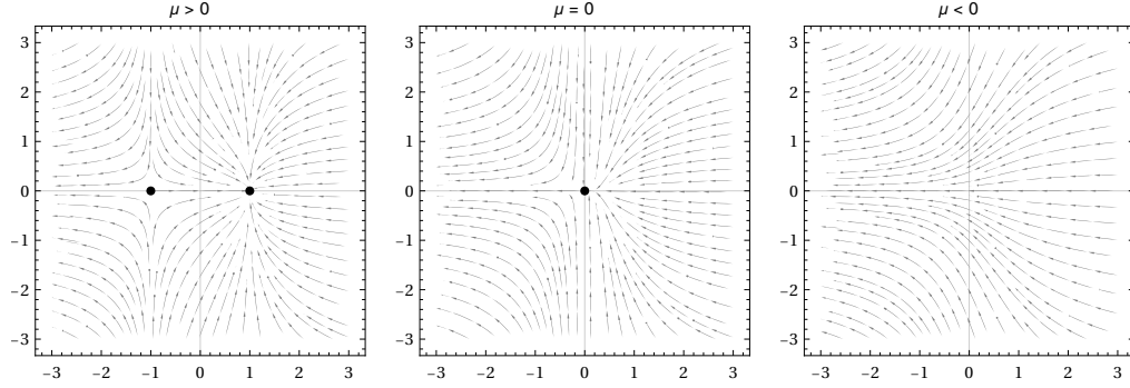
Figura 1.6: Retrato fase del sistema (1.10) para diferentes valores de \mu .
