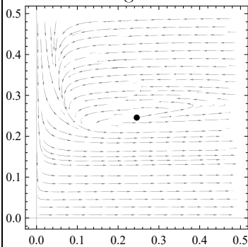
Centro lineal
