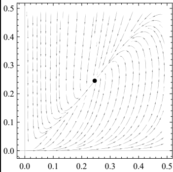
Nodo estable
