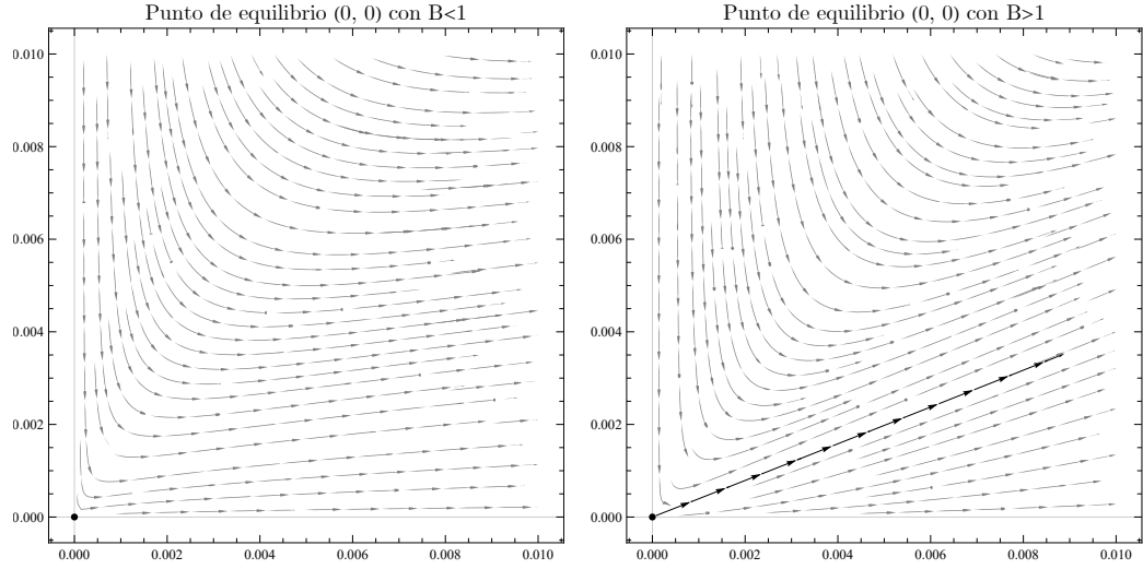
(a) Retrato fase del sistema (2.3) cerca al origen para valores paramétricos aleatorios con B < 1 . (b) Retrato fase del sistema (2.3) cerca al origen para valores paramétricos aleatorios con B > 1 .
