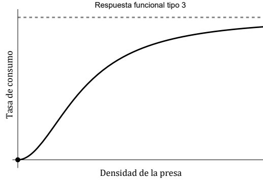
Figura 1.14: Respuesta funcional de Holling tipo 3.
