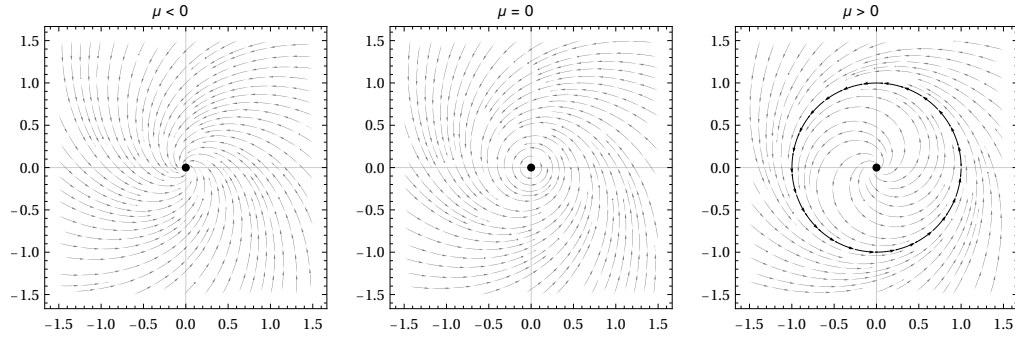
Figura 1.10: Ejemplo de bifurcación de Hopf supercrítica en el sistema (1.9) asociado a f_\mu(r, \theta) = (\mu r - r^3, 1 + r^2) .
