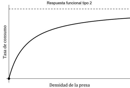
Figura 1.13: Respuesta funcional de Holling tipo 2.
