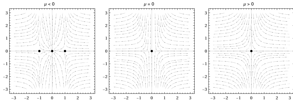
Figura 1.9: Ejemplo de bifurcación de pitchfork subcrítica en el sistema (1.9) asociado a f_\mu(x, y) = (\mu x + x^3, -y) .
