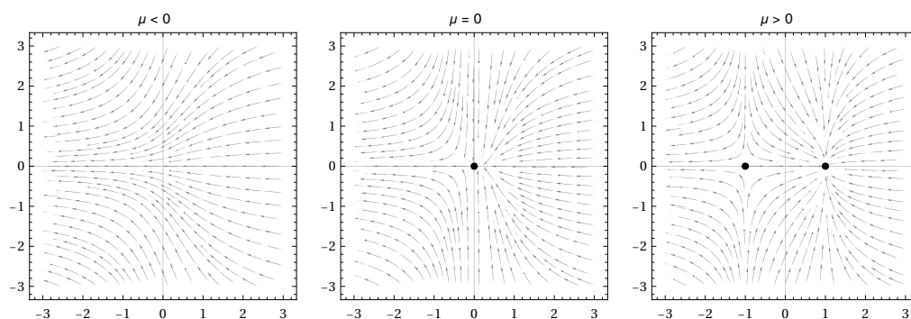
Figura 1.6: Ejemplo de bifurcación silla-nodo en el sistema (1.9) asociado a f_\mu(x, y) = (\mu - x^2, -y) .
