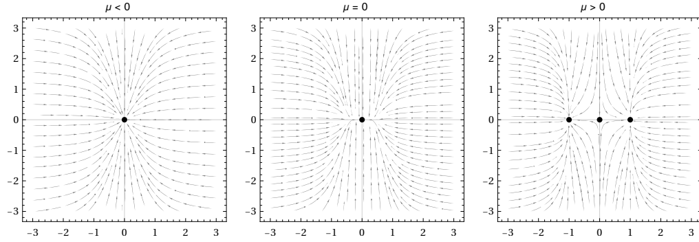
Figura 1.8: Ejemplo de bifurcación de pitchfork supercrítica en el sistema (1.9) asociado a f_\mu(x, y) = (\mu x - x^3, -y) .
