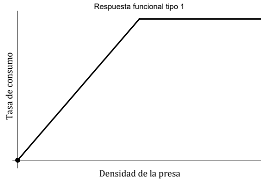
Figura 1.12: Respuesta funcional de Holling tipo 1.
