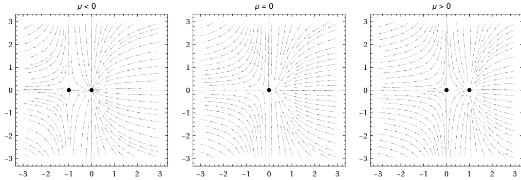
Figura 1.7: Ejemplo de bifurcación transcritical en el sistema (1.9) asociado a f_\mu(x, y) = (\mu x - x^2, -y) .
