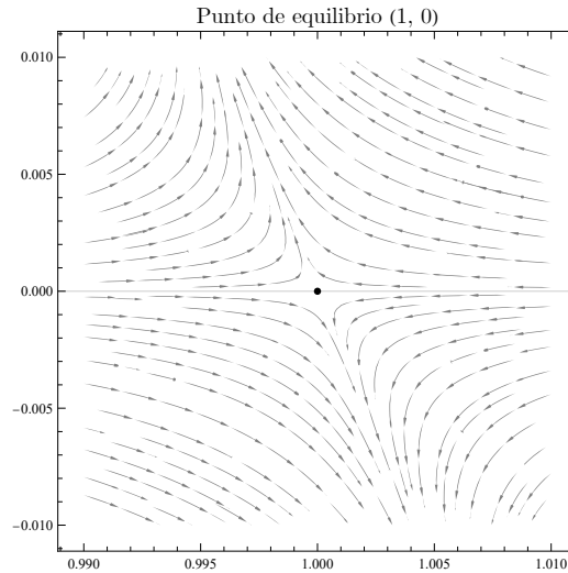
Figura 3.1: Punto de equilibrio (1, 0) para valores paramétricos aleatorios.
