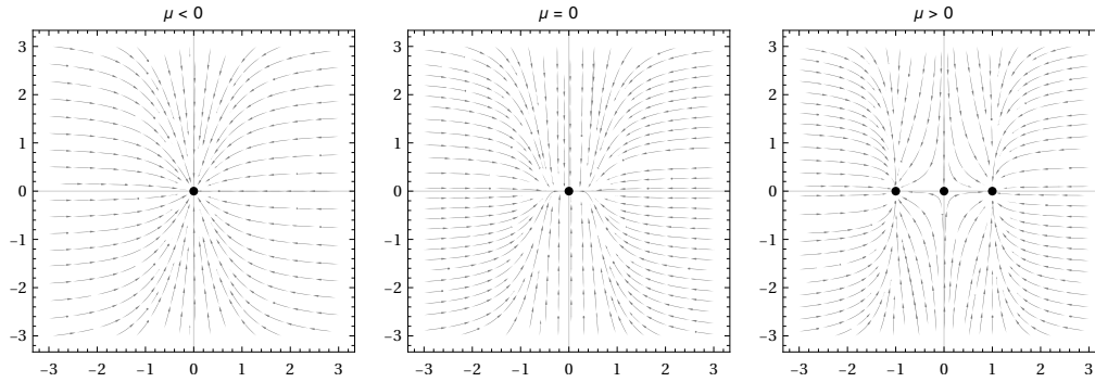
Figura 2.8: Ejemplo de bifurcación de pitchfork supercrítica en el sistema (2.9) asociado a f_\mu(x, y) = (\mu x - x^3, -y) .
