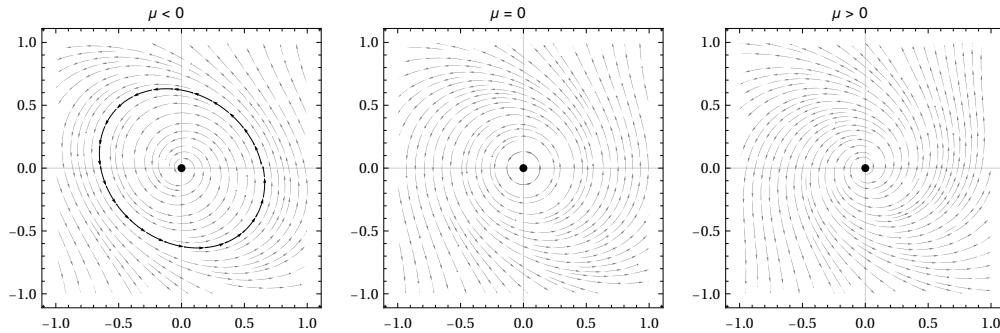
Figura 2.11: Ejemplo de bifurcación de Hopf subcrítica en el sistema (2.9) asociado a f_\mu(x, y) = (\mu x - y + xy^2, x + ay + y^3) .
