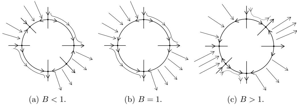
Figura 3.2: Blow-up en el origen del sistema (3.3) para diferentes valores de B .
