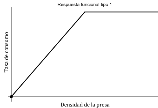
Figura 2.12: Respuesta funcional de Holling tipo 1.
