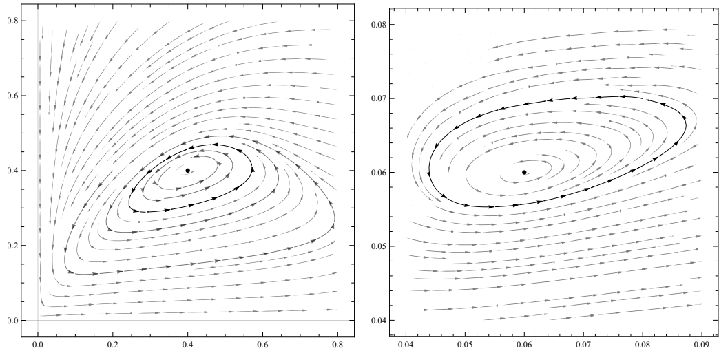
(a) Bifurcación de Hopf supercrítica ( L_1 = -0,0250864 ) del sistema (3.3) para los valores A = 0,05 ; H = 0,4 ; B = B_c = 0,181538 y Q = 0,609375 con el punto crítico de estudio como un foco débil inestable. (b) Bifurcación de Hopf subcrítica ( L_1 = 0,0589 ) del sistema (3.3) para los valores A = 0,05 ; H = 0,06 ; B = B_c = 0,109508 y Q = 1,59278 con el punto crítico de estudio como un foco débil estable.
