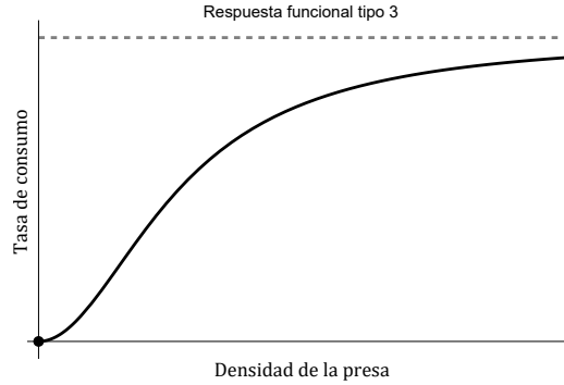
Figura 1.14: Respuesta funcional de Holling tipo 3.
