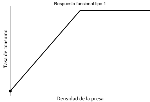
Figura 1.12: Respuesta funcional de Holling tipo 1.
