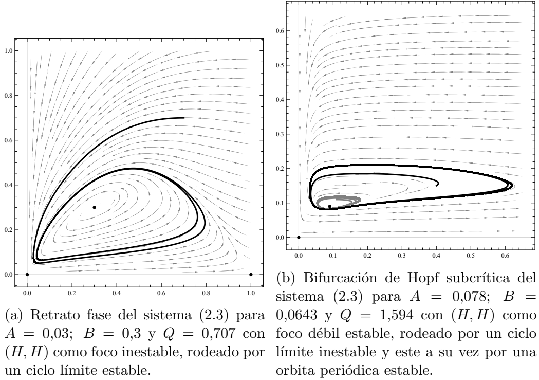
Figura 4.1: Órbitas periódicas del modelo de estudio.
