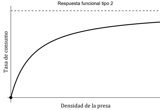
Figura 1.13: Respuesta funcional de Holling tipo 2.
