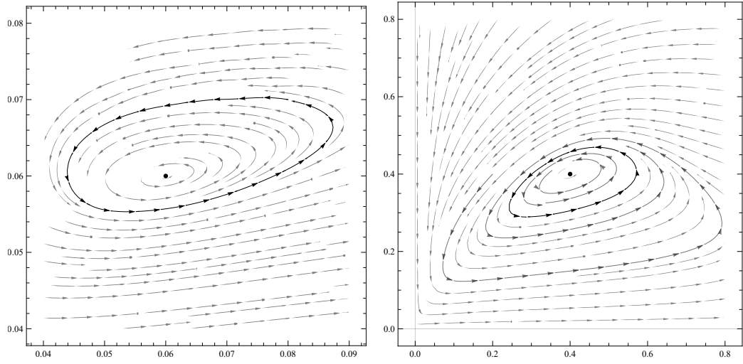
(a) Bifurcación de Hopf subcrítica ( l_1 = 0,0589 ) del sistema (2.3) para los valores A = 0,05 ; H = 0,06 ; B = B_c = 0,109508 y Q = 1,59278 con el punto crítico de estudio como un foco débil estable. (b) Bifurcación de Hopf supercrítica ( l_1 = -0,0250864 ) del sistema (2.3) para los valores A = 0,05 ; H = 0,4 ; B = B_c = 0,181538 y Q = 0,609375 con el punto crítico de estudio como un foco débil inestable.
