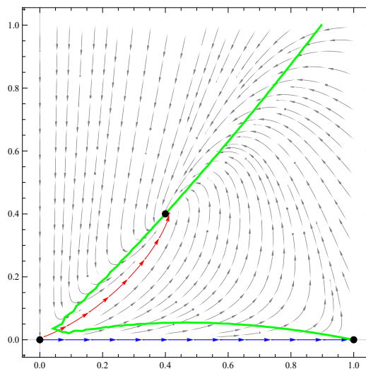
Figura 4.2: Variedad inestable e isoclina asociada a la pendiente \frac{B-1}{B} del sistema (2.3), para A = 0,05 ; B = 1,5 y Q = 0,61 .
