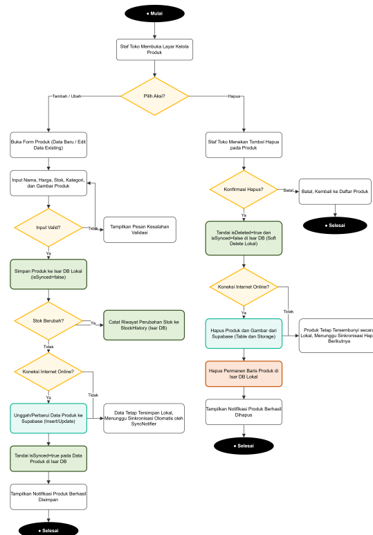
Gambar 3.8 Activity Diagram Kelola Produk (Tambah/Ubah/Hapus)
