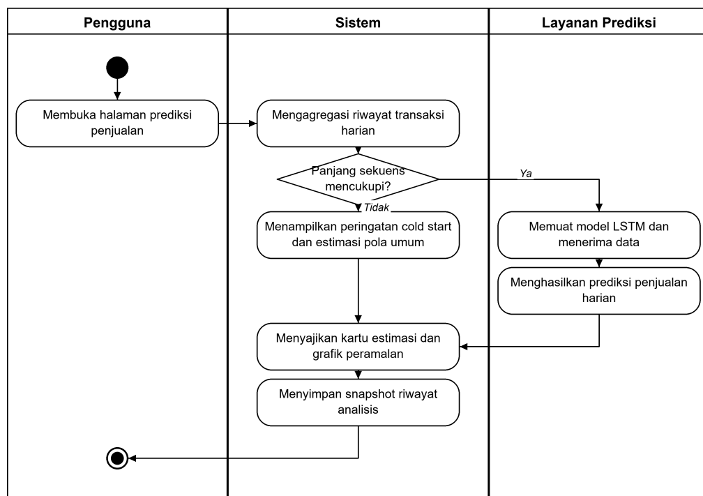
Gambar 3.5 Activity Diagram Melihat Prediksi Penjualan Harian
