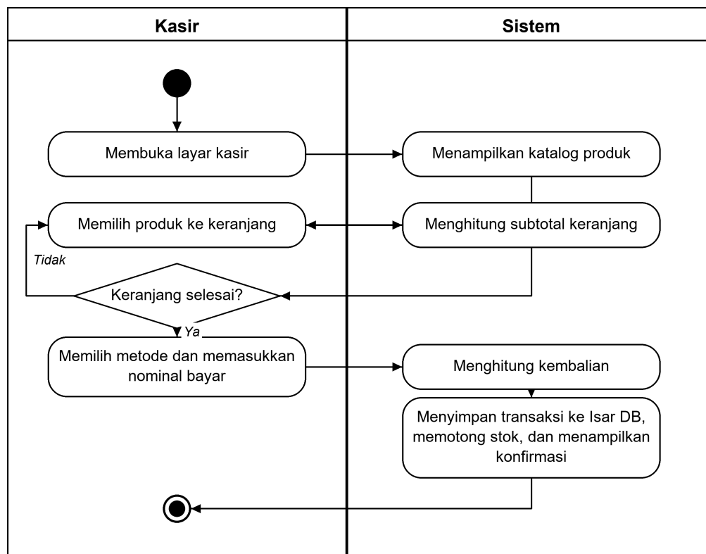
Gambar 3.4 Activity Diagram Melakukan Checkout
