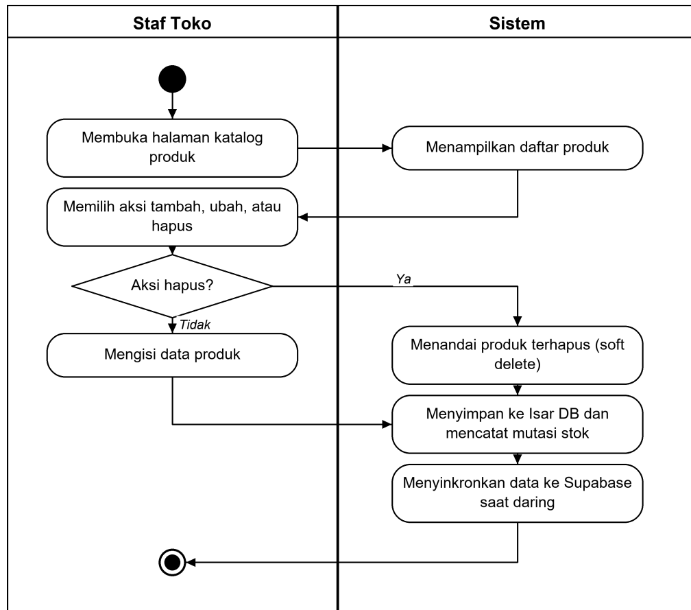
Gambar 3.3 Activity Diagram Mengelola Katalog Produk
