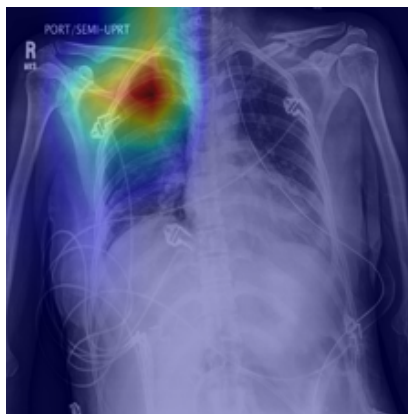
Grad-CAM · A
