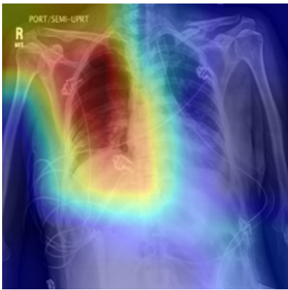
Grad-CAM · B
