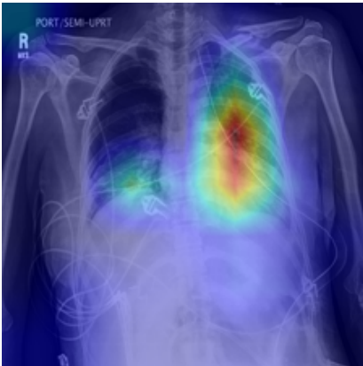
Grad-CAM · A
