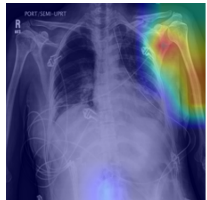
Grad-CAM · B
