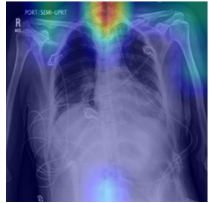
Grad-CAM · B
