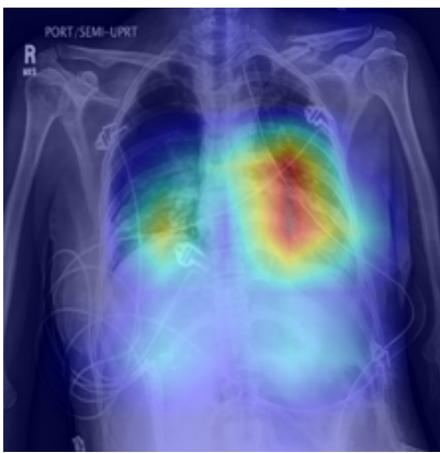
Grad-CAM · A
