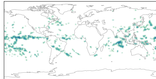
f553 — ascent
