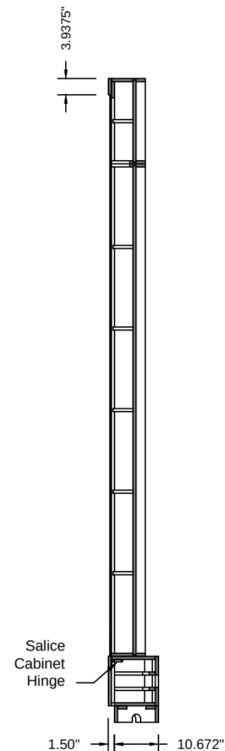
Section E SCALE: 3/8" = 1'-0"
