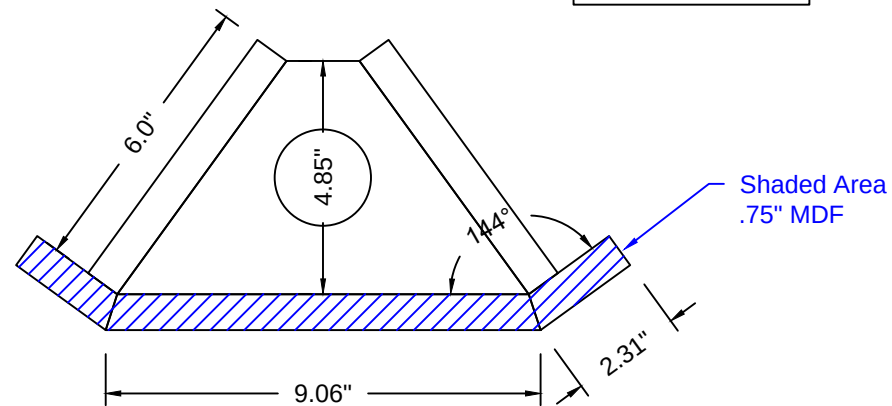
Plan View SCALE: 3" = 1'-0"
