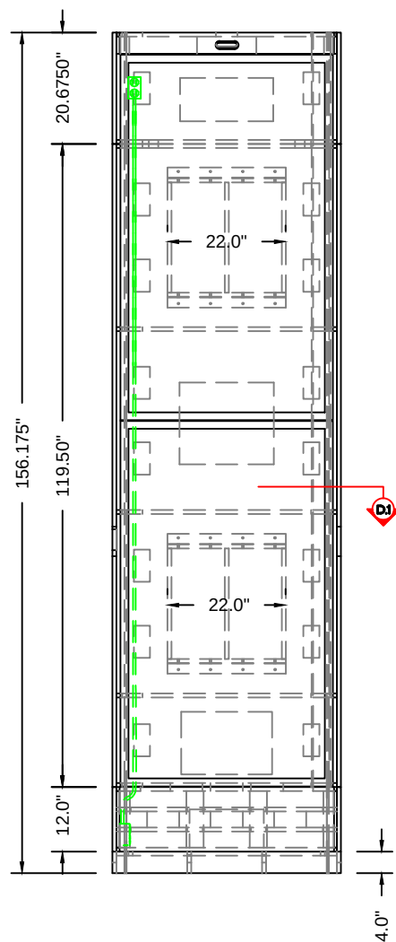
Front Elevation SCALE: 3/8" = 1'-0"
