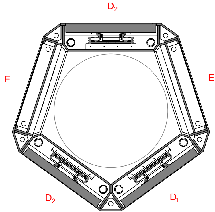
Column Section SCALE: 1/2" = 1'-0"
