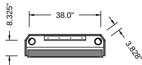
Section D.1 SCALE: 3/8" = 1'-0"
