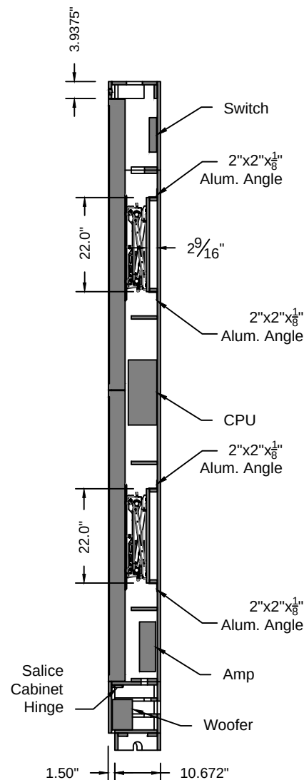
Section D SCALE: 3/8" = 1'-0"
