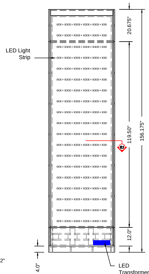
Front Elevation SCALE: 3/8" = 1'-0"
