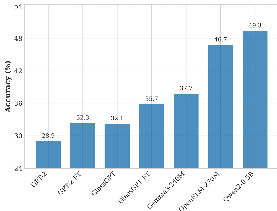
PIQA Benchmark
