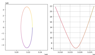
Figure 3.3.1 – Trajectoire de l'orbite de référence \gamma .
