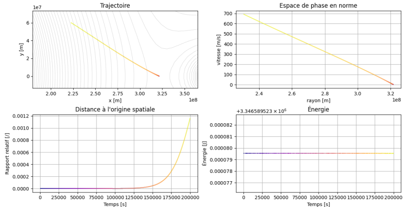
Figure 2.3.2 – Simulation numérique par schéma de Runge-Kutta 4 de la divergence de l'orbite autour de L1. Condition initiale : immobile à 100 m de L1.
