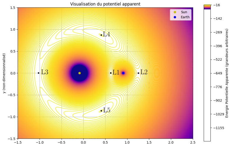
Figure 2.1.3 – Positions des points de Lagrange dans le plan d'étude.
