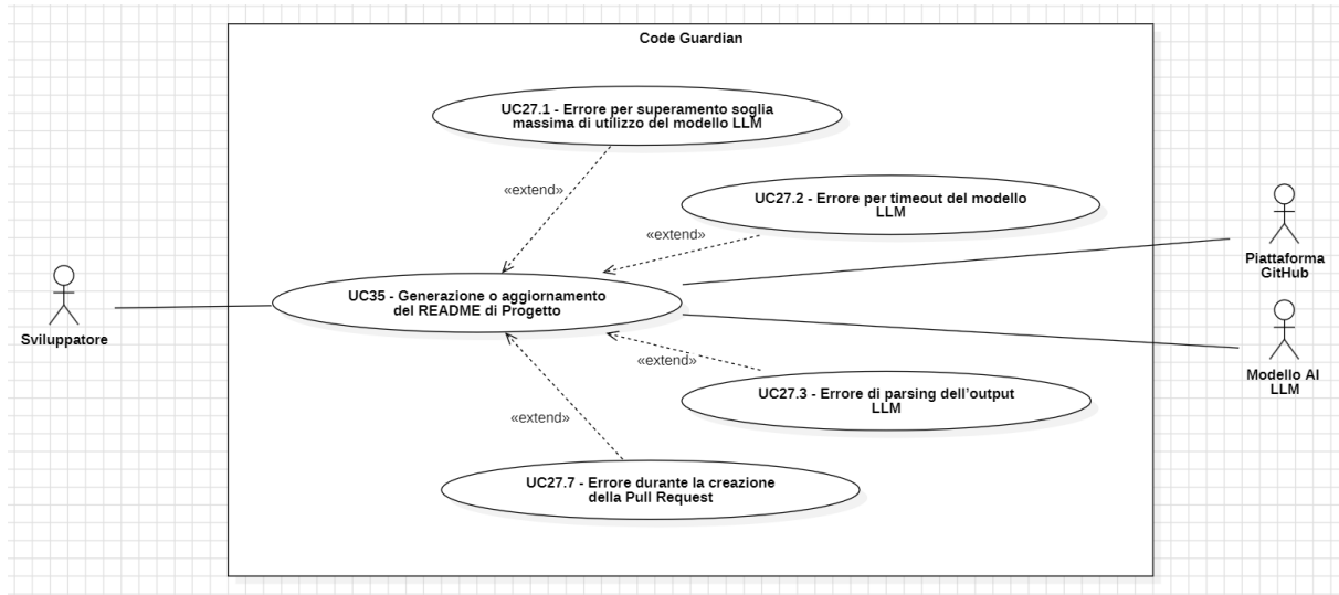
Figura 38: Aggiornamento del README di Progetto esistente
