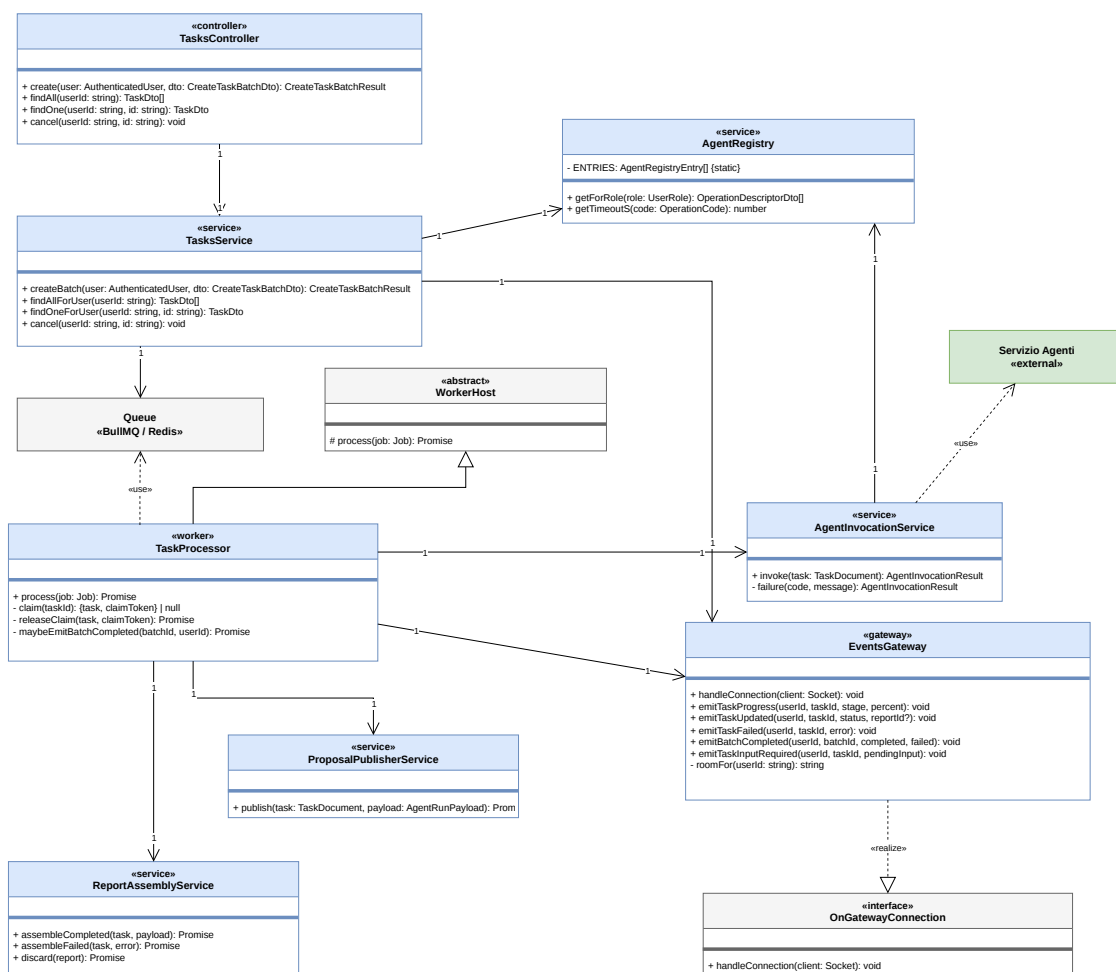
Figura 5: Struttura interna dell'orchestrazione ed esecuzione delle Task.
