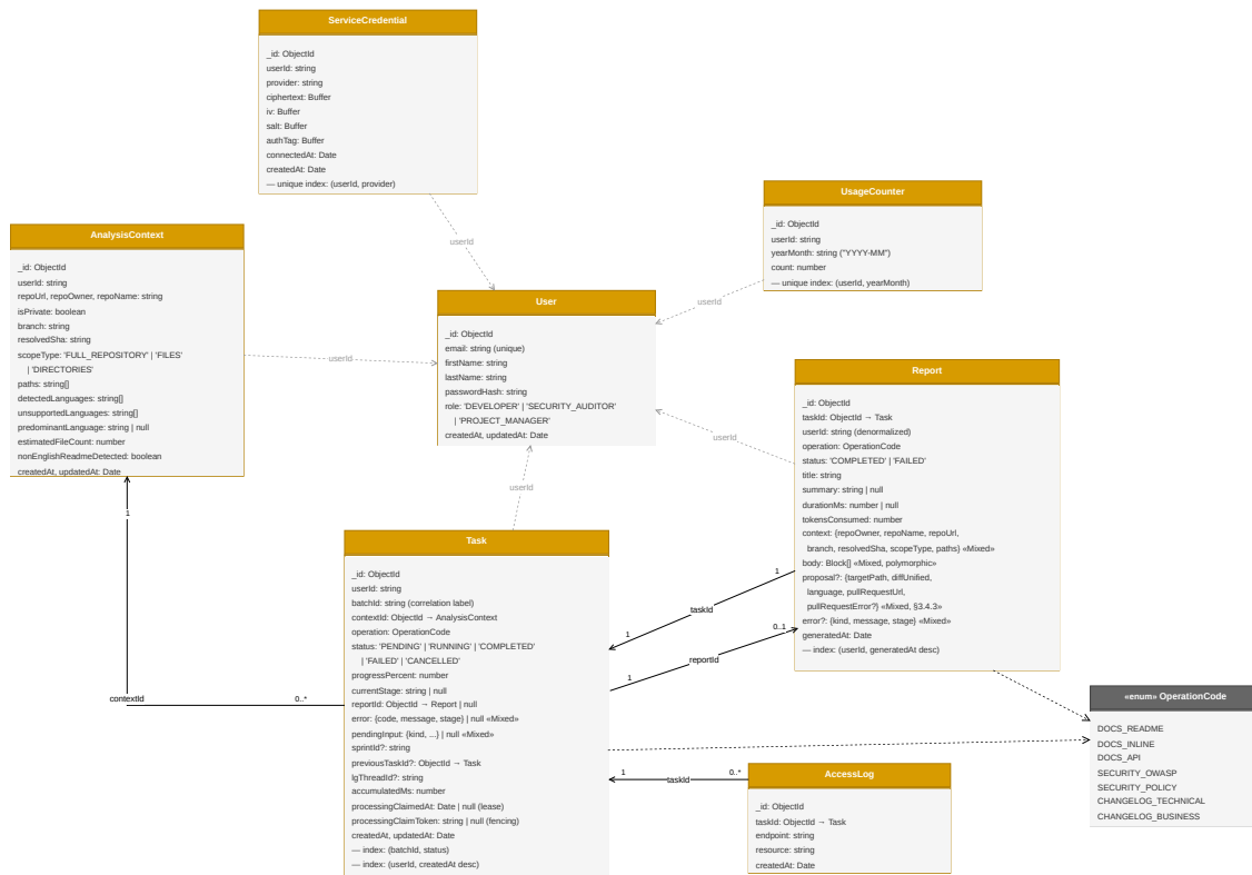
Figura 9: Modello dei dati persistenti su MongoDB.
