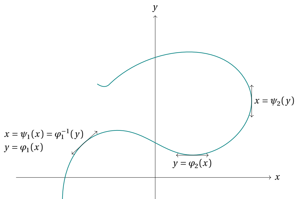
FIGURE 24 : Fonctions implicites.
