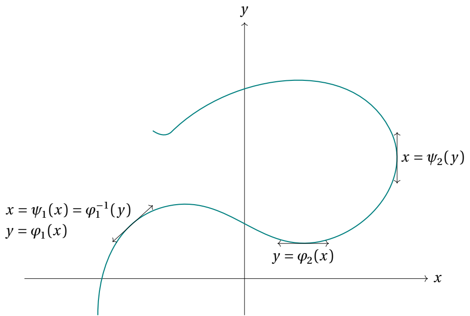
FIGURE 22 : Fonctions implicites.
