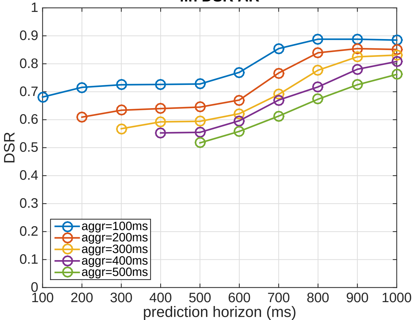
lin DSR AR
